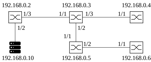
Figure 47. Réseau avec serveur TFTP
