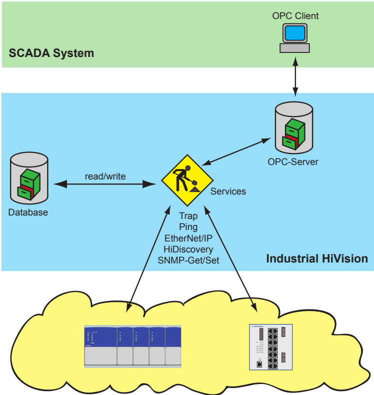
Abbildung 51. Anbindung an Prozessvisualisierungssystem
