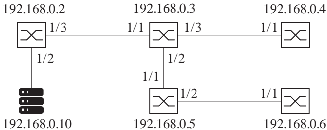
Abbildung 47. Netz mit TFTP-Server
