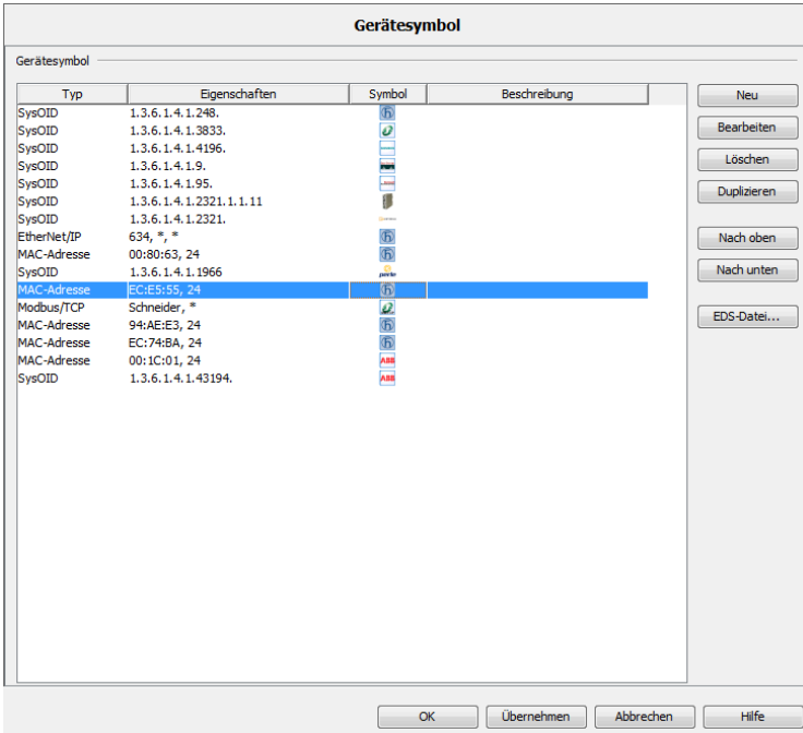
Abbildung 90. Zuweisungstabelle für Gerätesymbole
