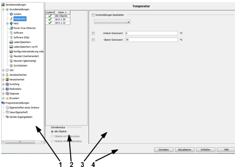
Abbildung 39. Übersicht Dialog MultiConfig™ .
