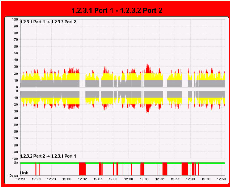
Abbildung 115. Verbindungsstatus-Widget mit aktivierten Funktionen Von oben nach unten und Gestapelt.
