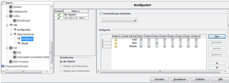
Abbildung 43. Gerät 1 TSN > Gate Control List > Konfiguriert
