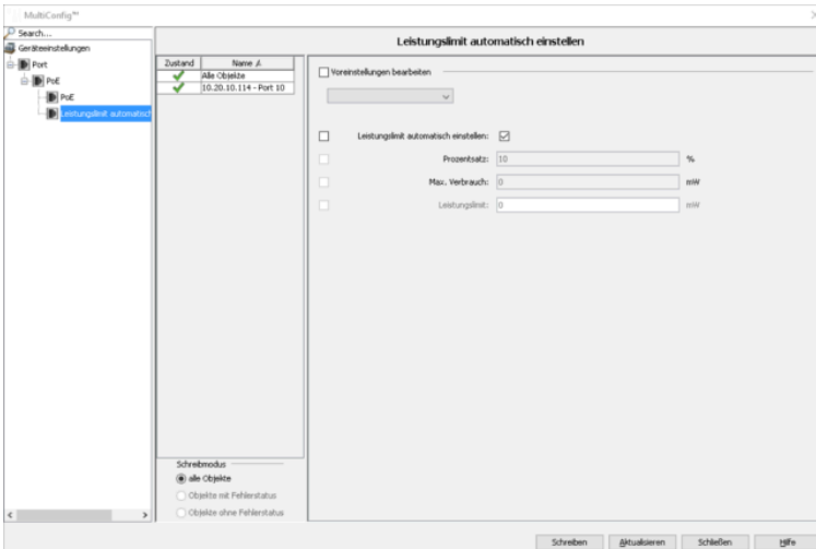
Abbildung 110. Konfiguration > MultiConfig™ > Geräteeinstellungen > PoE > Leistungslimit
