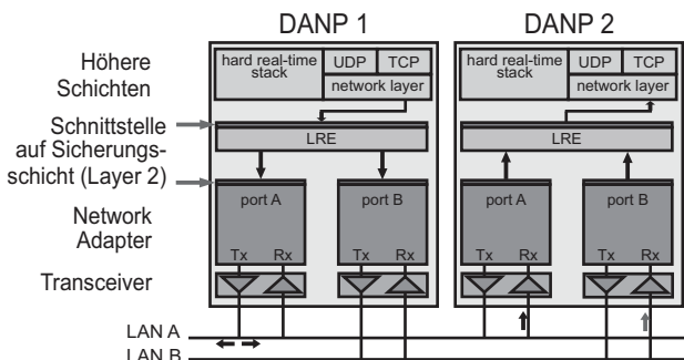
Abb. 38: Ablauf PRP/LRE
