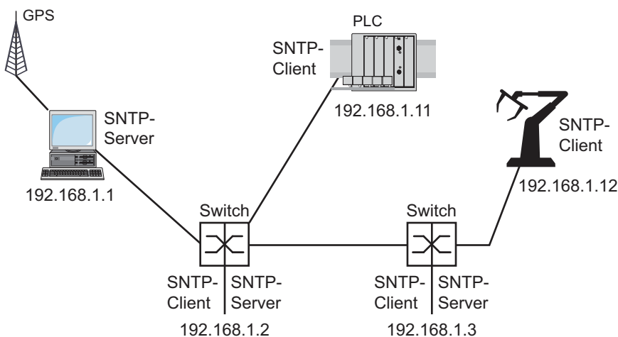
Abb. 20: Beispiel SNTP-Kaskade
