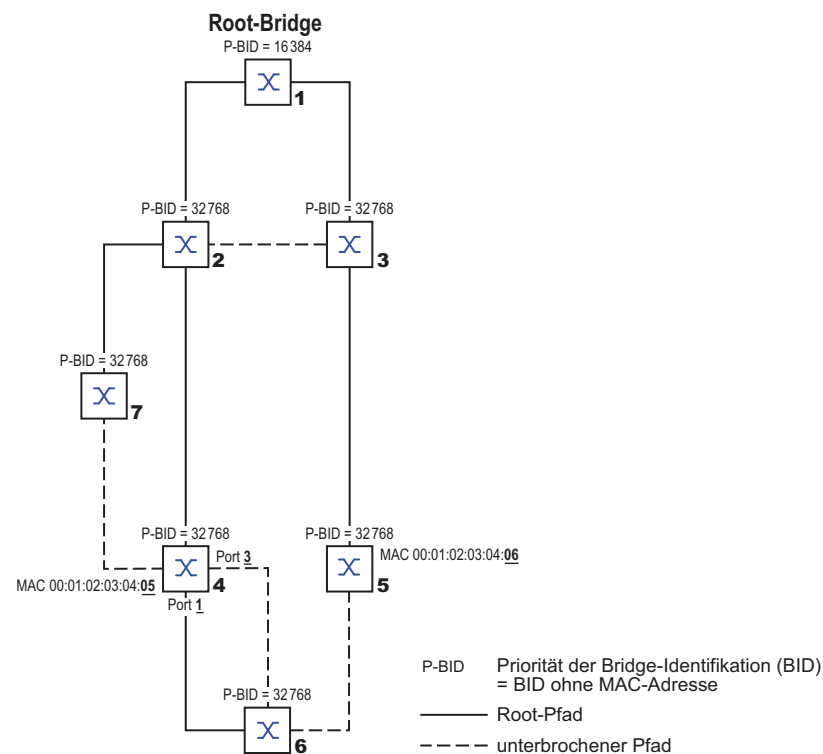
Abb. 50: Beispiel für die Bestimmung des Root-Pfads
