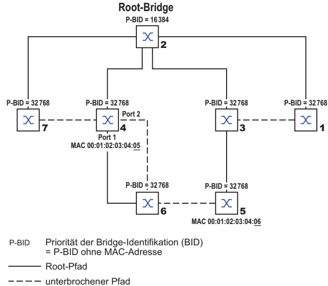
Abb. 52: Beispiel für die Manipulation der Baumstruktur
