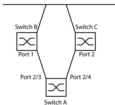
Abb. 40: Link-Backup Beispiel-Netzwerk
