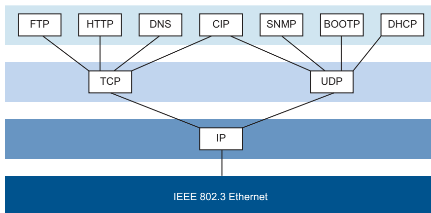
Abb. 54: IEEE 802.3 EtherNet/IP
