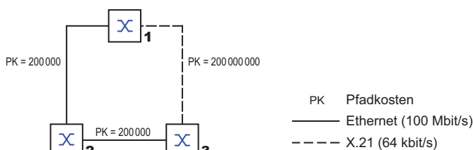
Abb. 34: Pfadkosten
