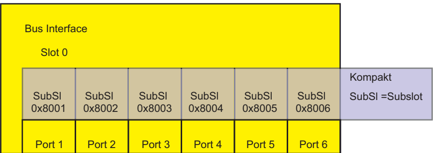
Abb. 56: Kompaktes Gerät
