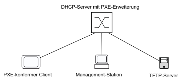
Abb. 46: Einfacher Aufbau eines Preboot eXecution Environment (PXE)-Setups
