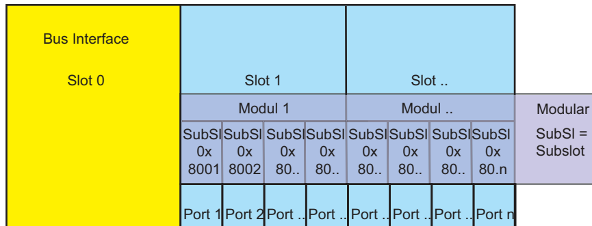
Abb. 57: Modulares Gerät
