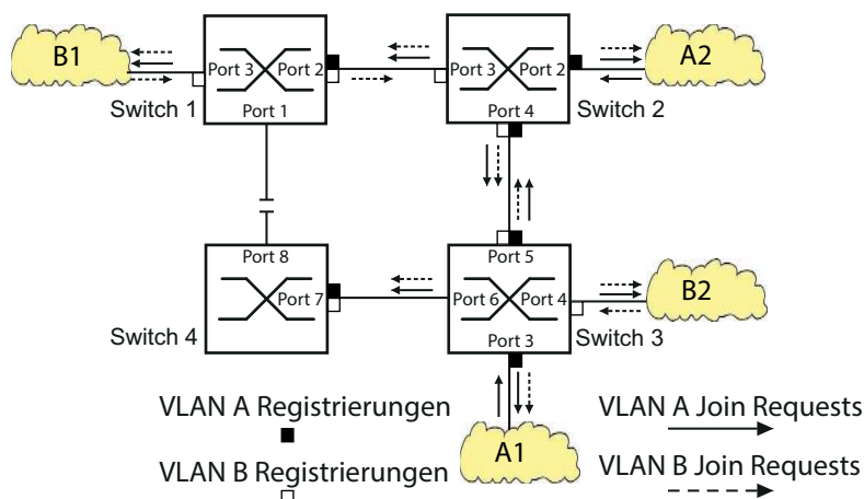
Abb. 91: MVRP-Beispiel-Netz für VLAN-Registrierung
