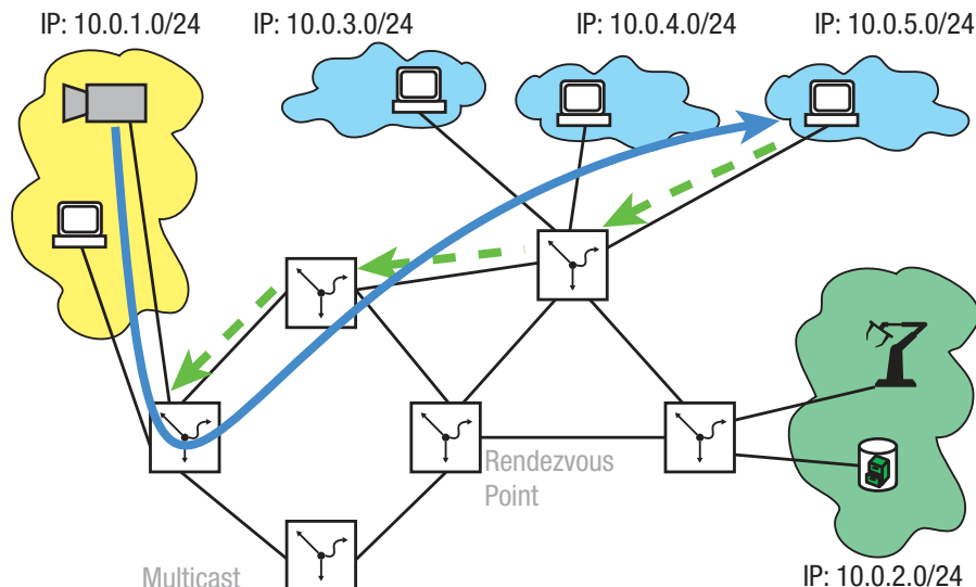
Abb. 115: Topologiewechsel vom RPT auf den direkten Pfad (STP)
