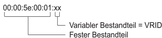
Abb. 93: Virtuelle MAC-Adresse
