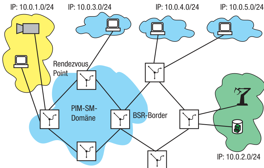
Abb. 117: Als BSR-Border-Router konfigurierte Router verwirfen Bootstrap-Nachrichten und begrenzen die PIM-SM-Domäne.
