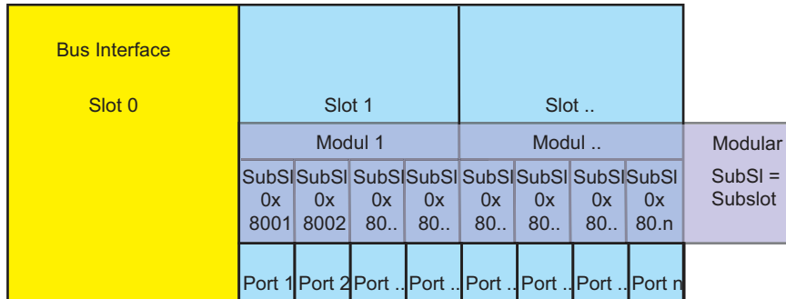
Abb. 138: Modulares Gerät
