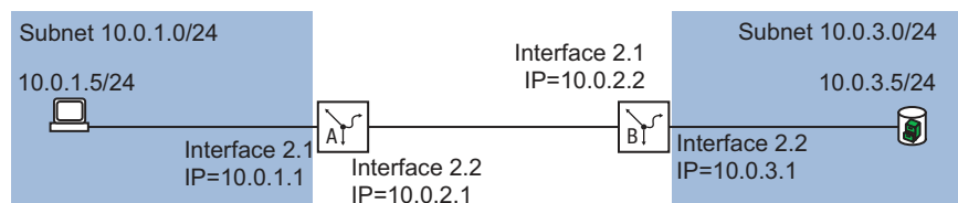
Abb. 84: Statisches Routing
