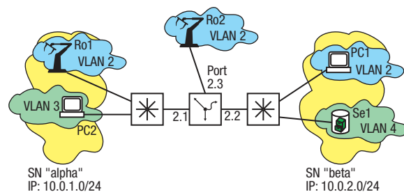
Abb. 108: Beispiel für ein Protokoll-basiertes VLAN
