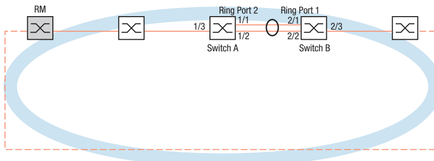
Abb. 39: Beispielkonfiguration für MRP-over-LAG
