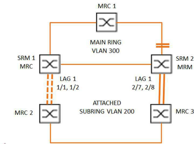
Abb. 57: Subring mit Link-Aggregation
