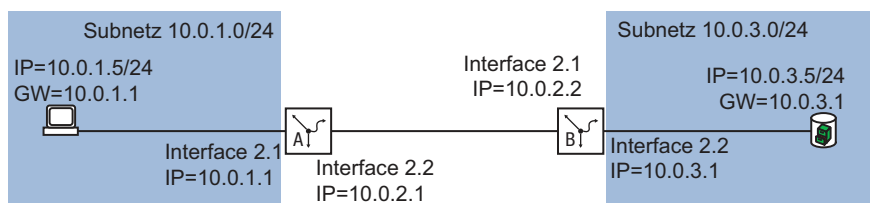
Abb. 107: Beispiel für die Konfiguration von OSPF
