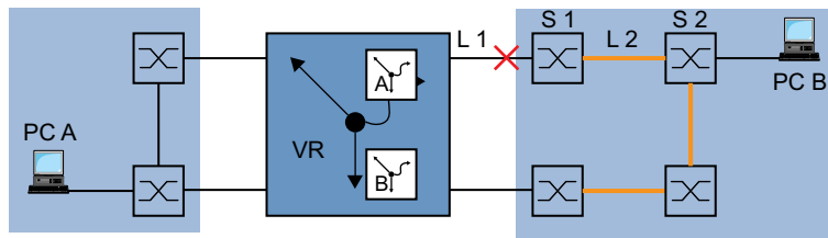
Abb. 75: Überwachen einer Leitung mit Interface-Tracking
