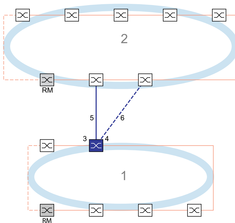
Abb. 65: Beispiel für die 1-Switch-Kopplung
