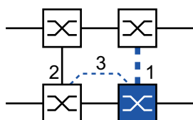
Abb. 72: 2-Switch-Kopplung mit Steuerleitung, Standby-Gerät
