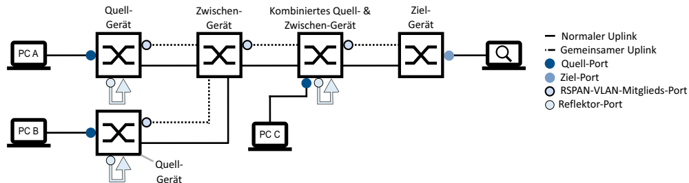
Abb. 81: Beispiel für eine komplexe Baum-Topologie mit Reflektor-Ports (mit separaten Uplinks)
