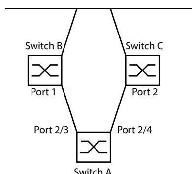
Abb. 50: Link-Backup Beispiel-Netzwerk
