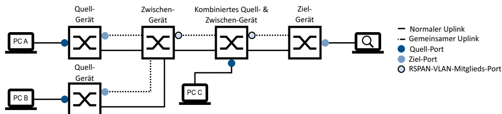
Abb. 82: Beispiel für eine komplexe Baum-Topologie, ohne Reflektor-Ports (mit separaten Uplinks)
