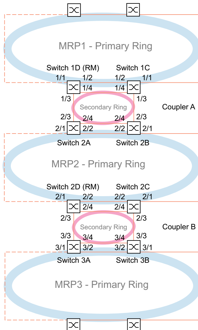
Abb. 74: Redundant Coupling Protocol-Zugtopologie: - Ports x/1 und x/2 sind MRP -Ring-Ports - Ports x/3 sind äußere RCP -Ports - Ports x/4 sind innere RCP -Ports
