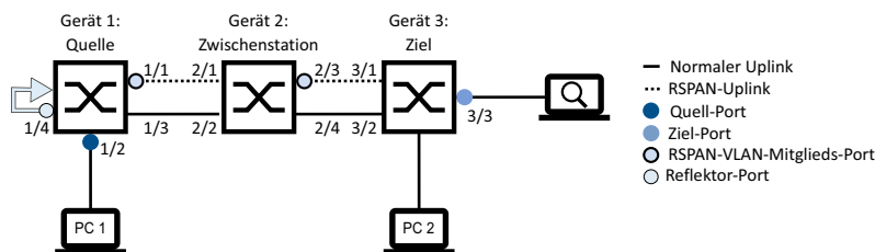
Abb. 84: RSPAN in einer Linien-Topologie, mittels Reflektor-Port (mit separaten Uplinks)
