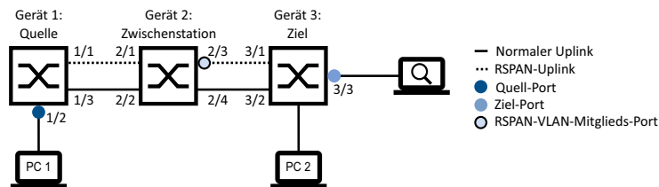
Abb. 86: RSPAN in einer Linien-Topologie, ohne einen Reflektor-Port (mit separaten Uplinks)
