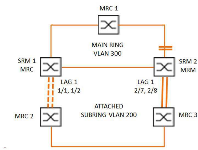
Abb. 57: Sub-Ring mit Link-Aggregation
