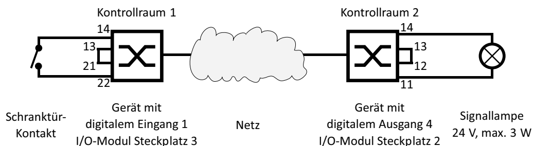
Abb. 90: Ein I/O-Signal über das Netz spiegeln
