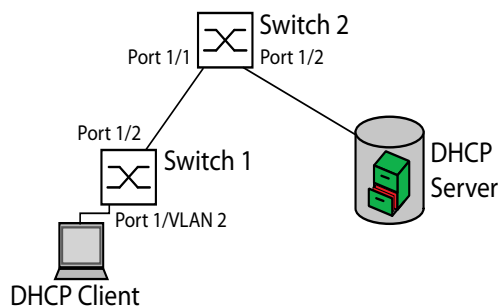
Abb. 89: Beispiel: DHCP-Schicht-2-Netz
