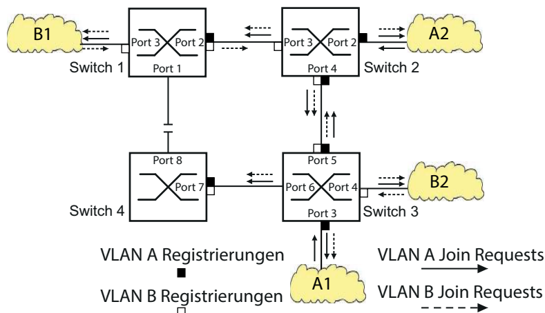
Abb. 92: MVRP -Beispiel-Netz für VLAN-Registrierung
