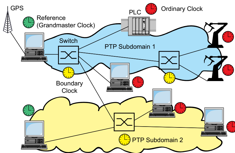
Abb. 17: Beispiel für PTP-Domänen
