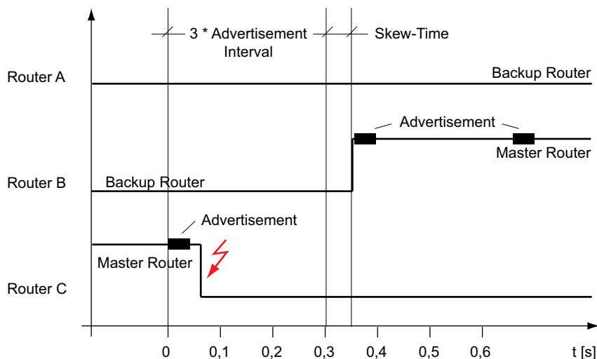
Abb. 92: Umschaltzeiten Master-Router <-> Backup-Router nach HiVRRP
