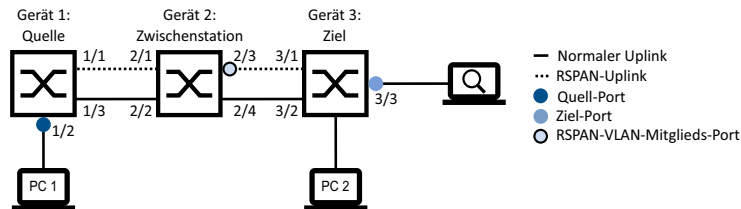
Abb. 126: RSPAN in einer Linien-Topologie, ohne einen Reflektor-Port (mit separaten Uplinks)
