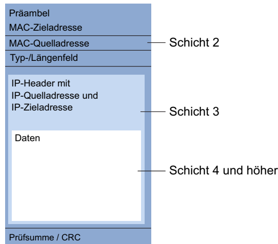
Abb. 81: Aufbau eines Datenpaketes aus Sicht des ISO/OSI-Referenzmodells
