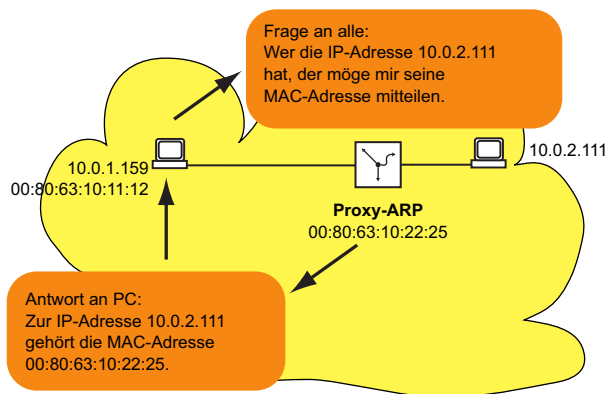
Abb. 82: Funktion Proxy-ARP
