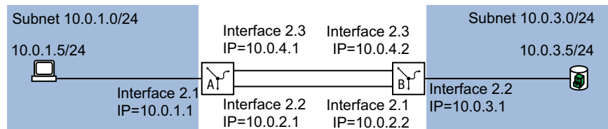
Abb. 88: Redundante statische Route
