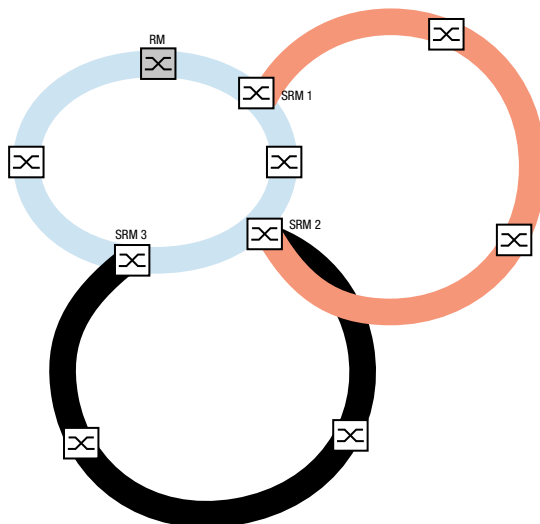
Abb. 56: Sonderfall: Ein Sub-Ring-Manager-Gerät verwaltet 2 Sub-Ringe (2 Instanzen). Das Sub-Ring-Manager-Gerät ist in der Lage, bis zu 20 Instanzen zu verwalten.
