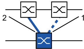
Abb. 69: 1-Switch-Kopplung 1: Kopplungs-Port 2: Partner-Kopplungs-Port
