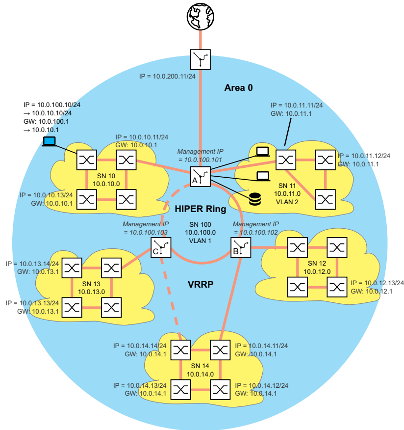
Abb. 109: Netzplan mit Management-IP-Adressen
