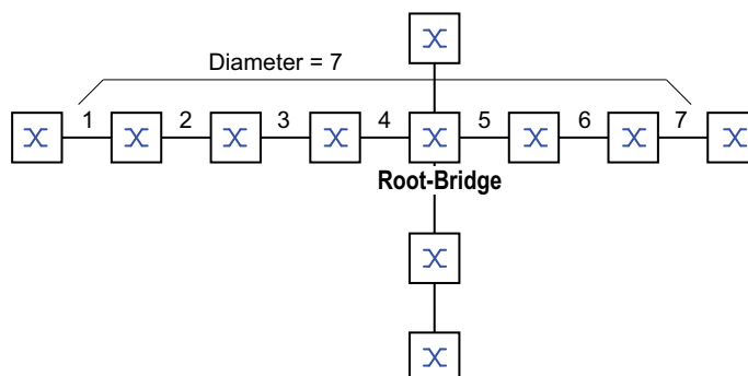
Abb. 45: Definition „Diameter“
