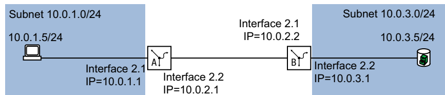
Abb. 87: Statisches Routing
