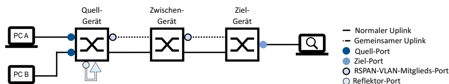
Abb. 119: Beispiel für eine Linien-Topologie mit einem Reflektor-Port (mit separaten Uplinks)
