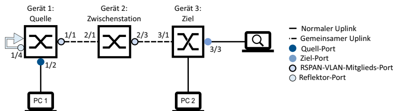
Abb. 125: RSPAN in einer Linien-Topologie, mittels Reflektor-Port (mit gemeinsamen Uplinks)
