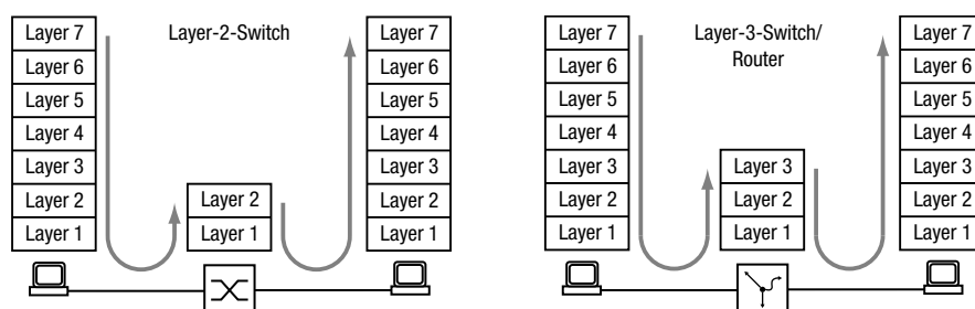
Abb. 78: Datentransport durch einen Switch und einen Router in den Schichten des OSI-Referenzmodells
