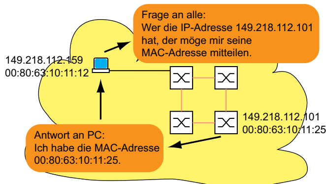
Abb. 80: ARP-Anfrage und -Antwort
