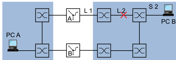
Abb. 112: Überwachen einer Leitung mit Ping-Tracking
