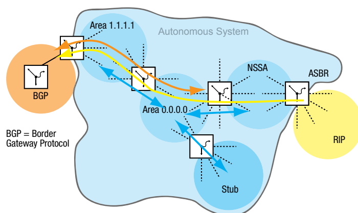
Abb. 100: LSA-Verteilung in die Area-Typen
