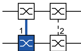
Abb. 63: 2-Switch-Kopplung, primäres Gerät 1: Kopplungs-Port 2: Partner-Kopplungs-Port
