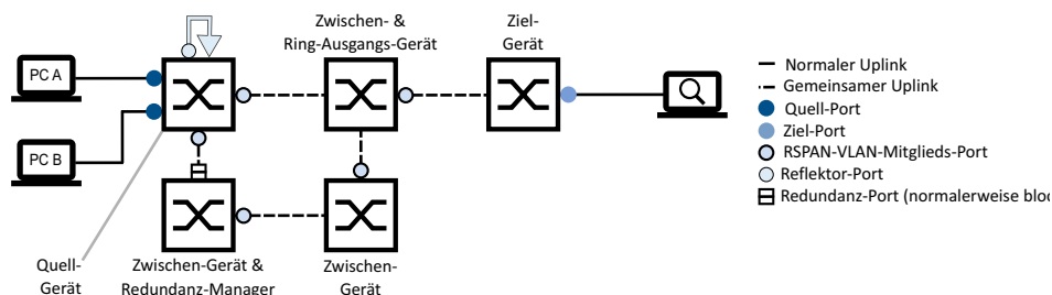
Abb. 123: Beispiel für eine einfache Ring-Topologie auf der Grundlage eines bestehenden redundanten Rings (mit gemeinsamen Links)
