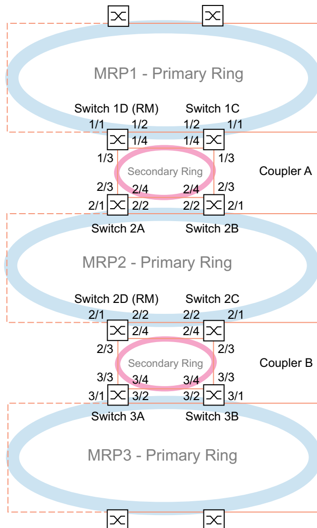
Abb. 77: Redundant Coupling Protocol-Zugtopologie: - Ports x/1 und x/2 sind MRP -Ring-Ports - Ports x/3 sind äußere RCP -Ports - Ports x/4 sind innere RCP -Ports
