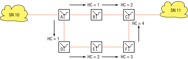
Abb. 96: Zählen des Hop Count
