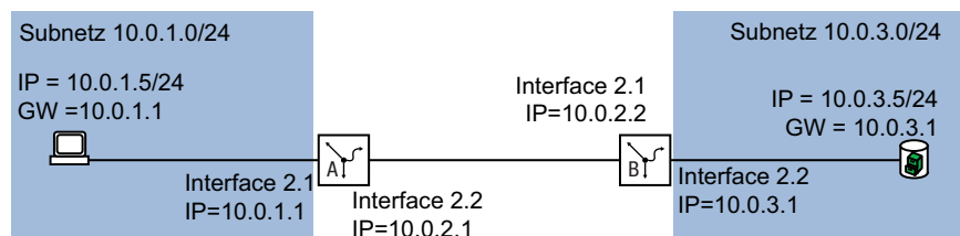
Abb. 98: Anwendungsbeispiel für ein RIP-Setup
