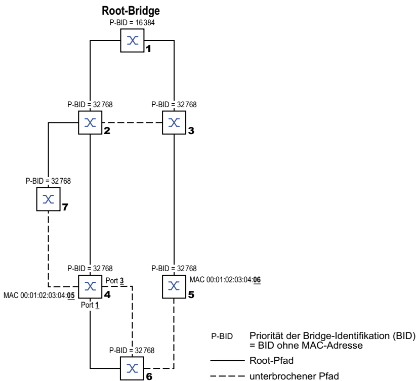
Abb. 48: Beispiel eines Netzplans für die Bestimmung des Root-Pfads
