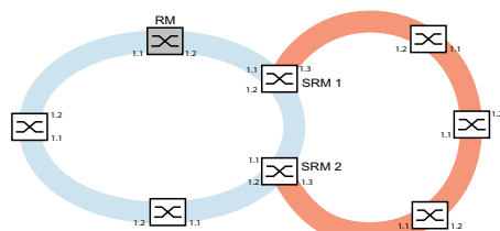
Abb. 54: Beispiel für eine Sub-Ring-Struktur blauer Ring = Hauptring orangefarbener Ring = Sub-Ring SRM = Sub-Ring-Manager RM = Ring-Manager
