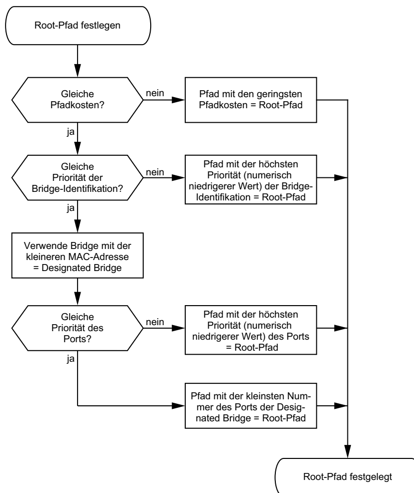
Abb. 47: Flussdiagramm Root-Pfad festlegen
