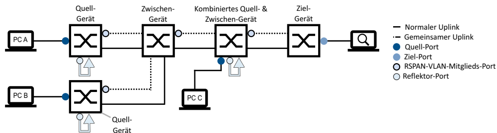
Abb. 121: Beispiel für eine komplexe Baum-Topologie mit Reflektor-Ports (mit separaten Uplinks)
