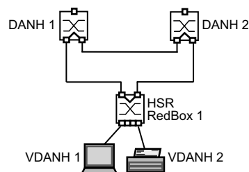
Abb. 40: VDANH mit einem HSR-Netz verbinden
