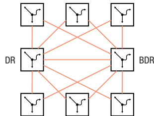
Abb. 103: LSA-Verteilung mit Designated-Router und Backup-Designated-Router
