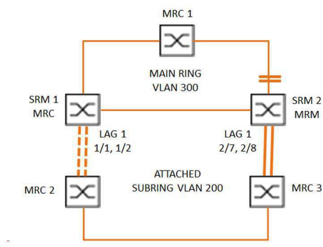
Abb. 60: Sub-Ring mit Link-Aggregation
