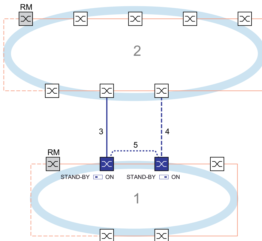
Abb. 65: Beispiel für die 2-Switch-Kopplung mit Steuerleitung 1: Ring 2: Backbone 3: Hauptleitung 4: Redundante Leitung 5: Steuerleitung
