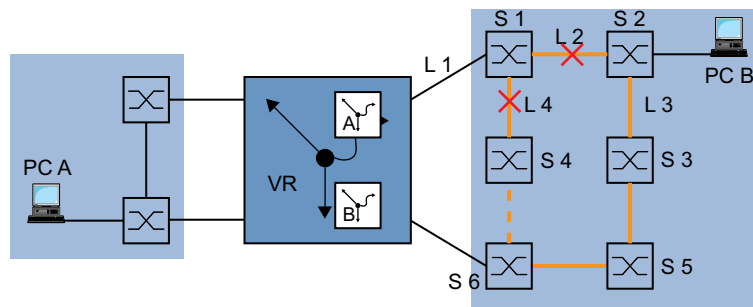
Abb. 113: Überwachen der Erreichbarkeit eines Geräts in einem redundanten Ring
