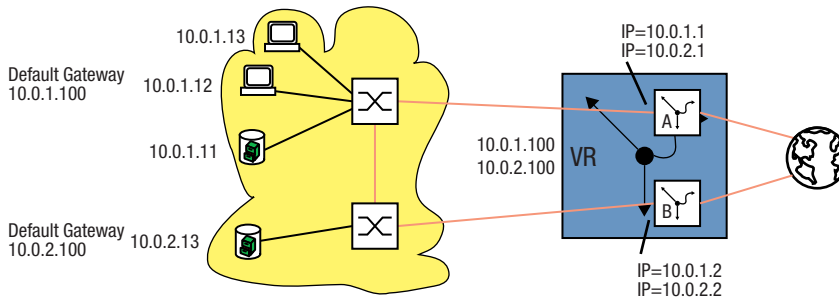
Abb. 95: Virtueller Router mit Multinetting
