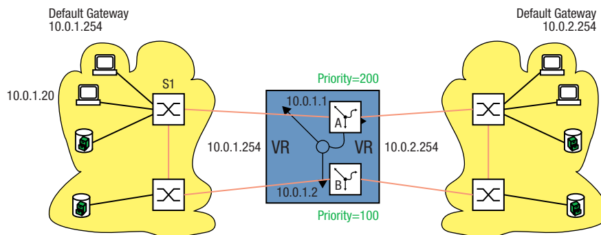
Abb. 94: Virtueller Router mit Lastverteilung
