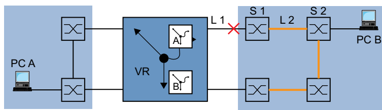
Abb. 111: Überwachen einer Leitung mit Interface-Tracking
