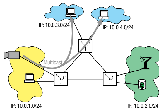
Abb. 106: Beispiel für eine Multicast-Anwendung
