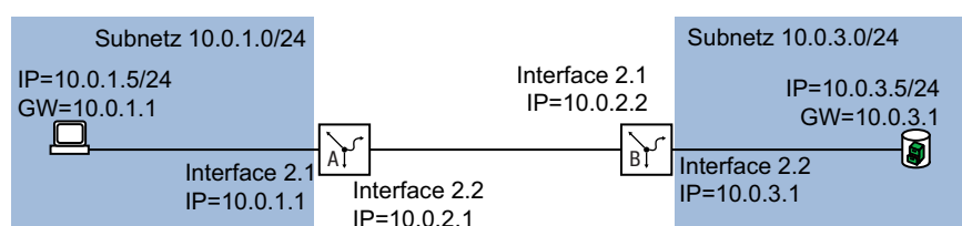
Abb. 104: Anwendungsbeispiel für ein OSPF-Setup
