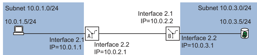
Abb. 89: Statisches Routing
