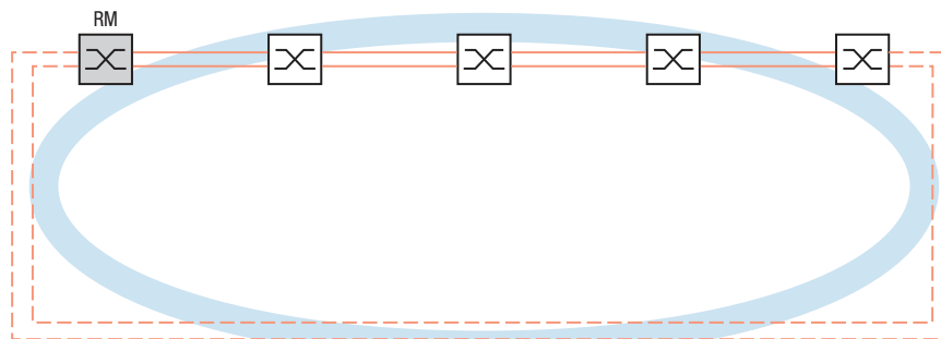
Abb. 41: Link-Aggregation für den gesamten MRP-Ring
