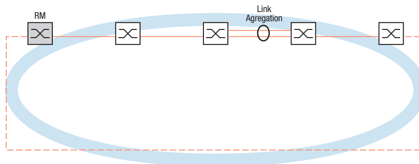
Abb. 40: Link-Aggregation über eine einzelne Verbindung eines MRP-Rings
