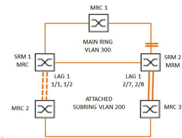
Abb. 62: Sub-Ring mit Link-Aggregation
