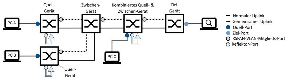
Abb. 123: Beispiel für eine komplexe Baum-Topologie mit Reflektor-Ports (mit separaten Uplinks)
