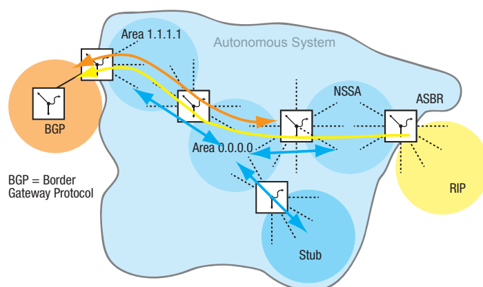
Abb. 102: LSA-Verteilung in die Area-Typen
