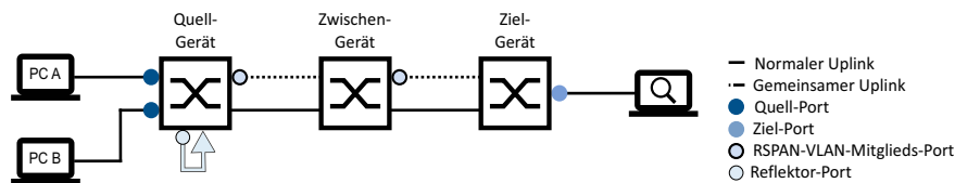
Abb. 121: Beispiel für eine Linien-Topologie mit einem Reflektor-Port (mit separaten Uplinks)
