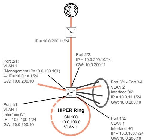
Abb. 112: IP-Parameter für Schicht-3-Gerät A
