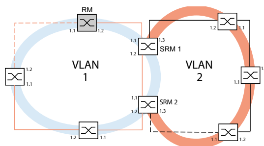
Abb. 60: Beispiel für eine Sub-Ring-Struktur mit VLANs orangefarbene Linie= Mitglieder des Hauptrings in VLAN 1 schwarze Linie= Mitglieder des Sub-Rings in VLAN 2 orange gestrichelte Linie= unterbrochenes Segment im Hauptring schwarz gestrichelte Linie= unterbrochenes Segment im Sub-Ring SRM = Sub-Ring-Manager RM = Ring-Manager
