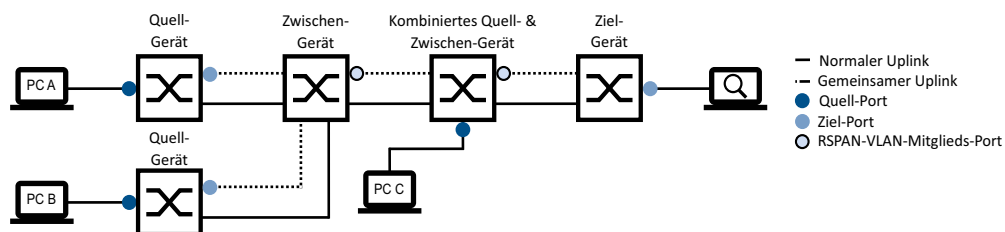
Abb. 124: Beispiel für eine komplexe Baum-Topologie, ohne Reflektor-Ports (mit separaten Uplinks)
