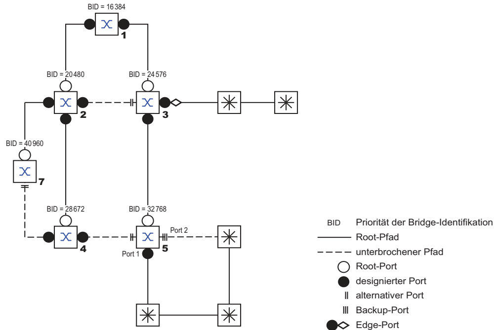
Abb. 53: Port-Rollen-Zuweisung
