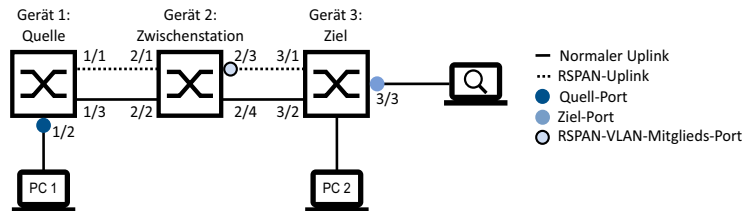
Abb. 128: RSPAN in einer Linien-Topologie, ohne einen Reflektor-Port (mit separaten Uplinks)
