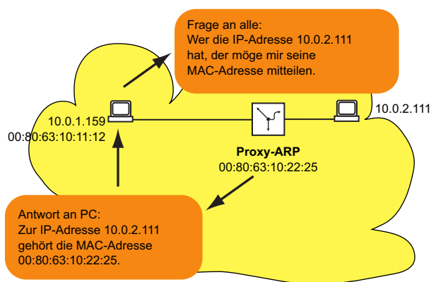
Abb. 84: Funktion Proxy-ARP
