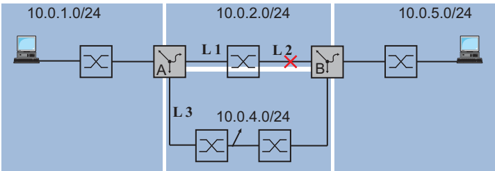
Abb. 116: Beispiel für statisches Route-Tracking
