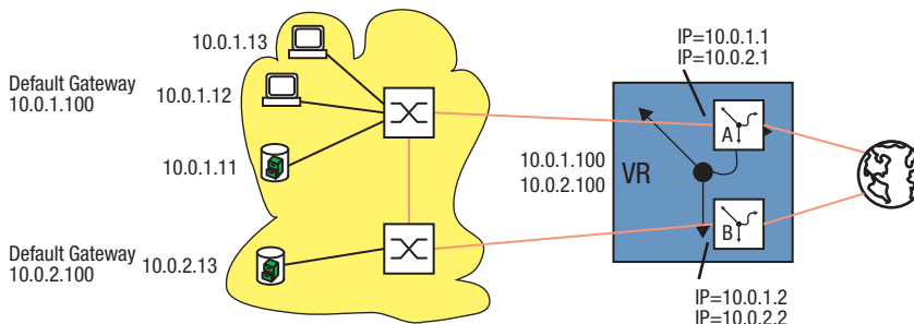
Abb. 97: Virtueller Router mit Multinetting
