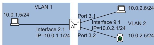
Abb. 88: VLAN-basiertes Router-Interface
