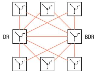
Abb. 105: LSA-Verteilung mit Designated-Router und Backup-Designated-Router
