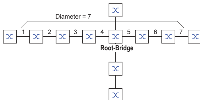
Abb. 47: Definition „Diameter“
