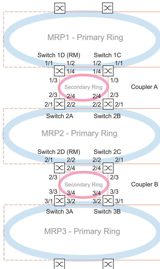
Abb. 79: Redundant Coupling Protocol-Zugtopologie: - Ports x/1 und x/2 sind MRP -Ring-Ports - Ports x/3 sind äußere RCP -Ports - Ports x/4 sind innere RCP -Ports
