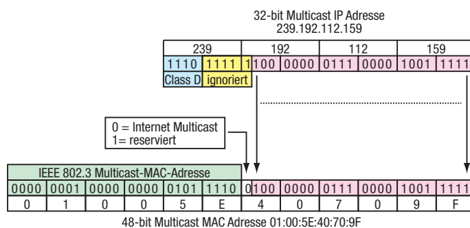
Abb. 109: Umsetzung der IP-Adresse in die MAC-Adresse
