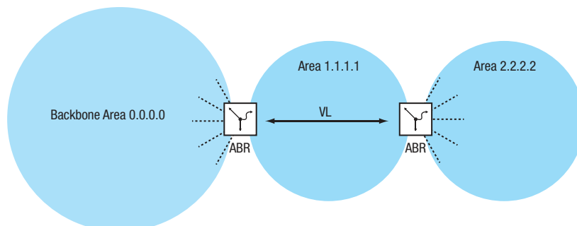
Abb. 103: Anbinden einer entfernten Area an die Backbone Area durch eine virtuelle Verbindung (VL)
