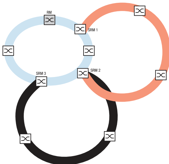
Abb. 58: Sonderfall: Ein Sub-Ring-Manager-Gerät verwaltet 2 Sub-Ringe (2 Instanzen). Das Sub-Ring-Manager-Gerät ist in der Lage, bis zu 20 Instanzen zu verwalten.
