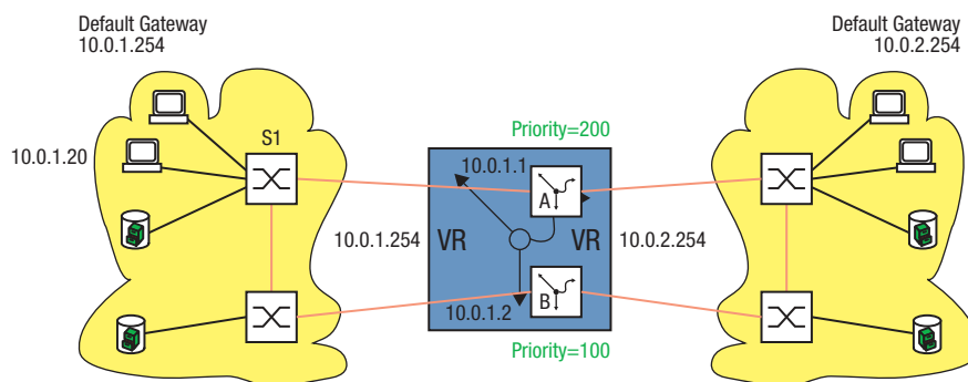
Abb. 96: Virtueller Router mit Lastverteilung
