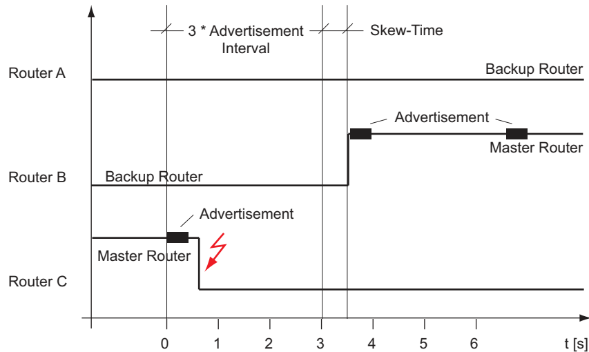
Abb. 93: Umschaltzeiten Master-Router <-> Backup-Router nach RFC 2338 VRRP-Priorität Router A = 64 VRRP-Priorität Router B = 128 VRRP-Priorität Router C = 254
