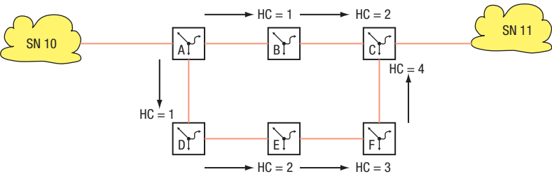
Abb. 98: Zählen des Hop Count
