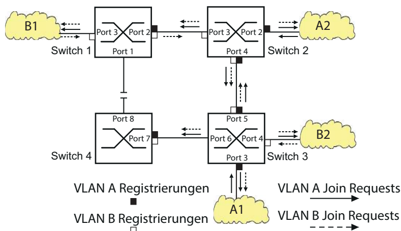
Abb. 133: MVRP-Beispiel-Netz für VLAN-Registrierung
