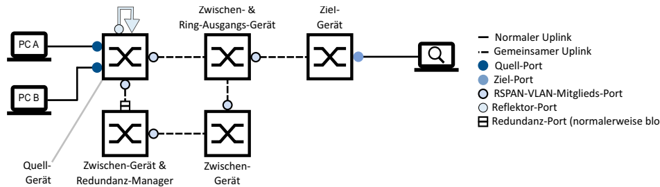
Abb. 125: Beispiel für eine einfache Ring-Topologie auf der Grundlage eines bestehenden redundanten Rings (mit gemeinsamen Links)
