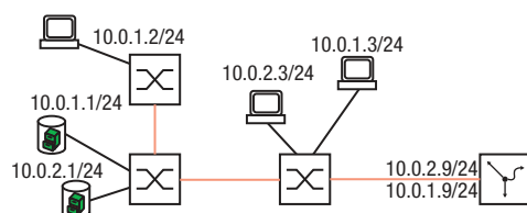
Abb. 85: Beispiel für Multinetting
