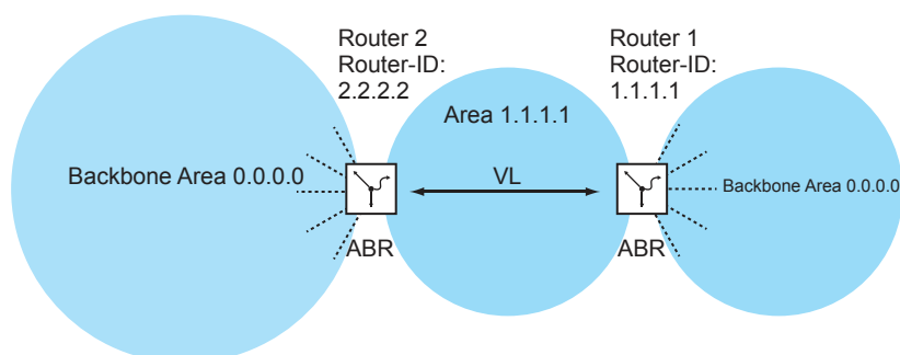
Abb. 104: Erweiterung der Backbone-Area durch eine virtuelle Verbindung (VL)
