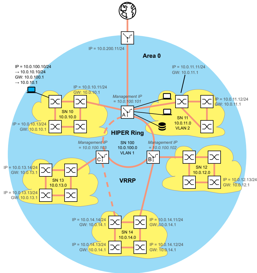
Abb. 111: Netzplan mit Management-IP-Adressen
