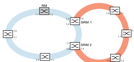
Abb. 56: Beispiel für eine Sub-Ring-Struktur blauer Ring = Hauptring oranger Ring = Sub-Ring SRM = Sub-Ring-Manager RM = Ring-Manager
