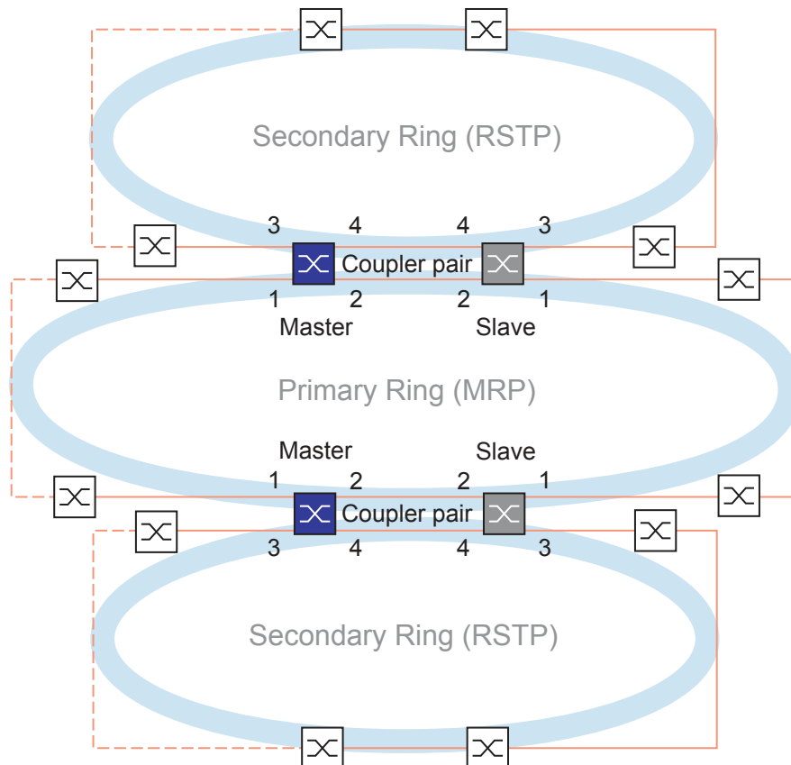
Abb. 78: Beispiel für eine redundante Zwei-Switch-Kopplung (2 Kopplerpaare)
