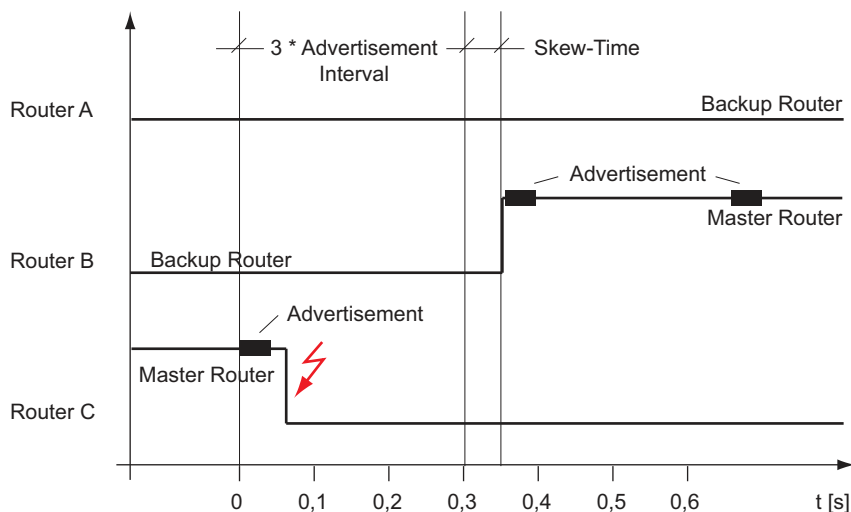
Abb. 94: Umschaltzeiten Master-Router <-> Backup-Router nach HiVRRP
