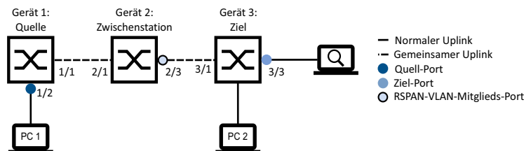
Abb. 129: RSPAN in einer Linien-Topologie, ohne einen Reflektor-Port (mit gemeinsamen Uplinks)
