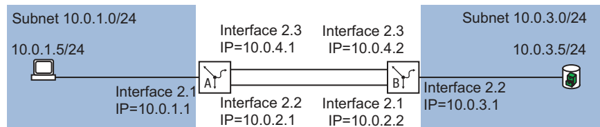
Abb. 90: Redundante statische Route
