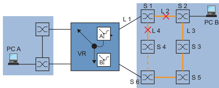
Abb. 115: Überwachen der Erreichbarkeit eines Geräts in einem redundanten Ring
