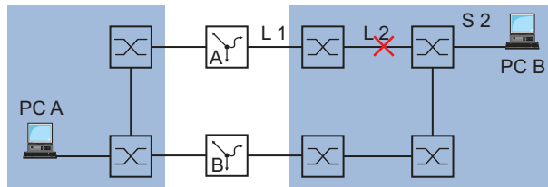
Abb. 114: Überwachen einer Leitung mit Ping-Tracking
