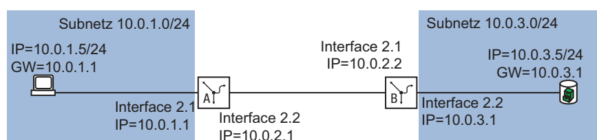
Abb. 106: Anwendungsbeispiel für ein OSPF-Setup
