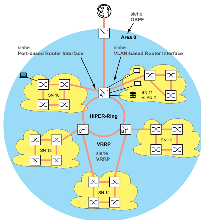
Abb. 110: Netzplan
