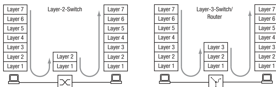
Abb. 80: Datentransport durch einen Switch und einen Router in den Schichten des OSI-Referenzmodells
