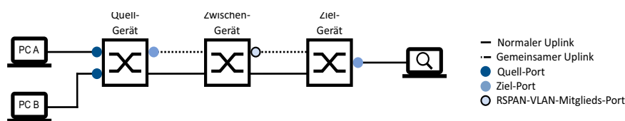
Abb. 122: Beispiel für eine Linien-Topologie, ohne Reflektor-Port (mit separaten Uplinks)
