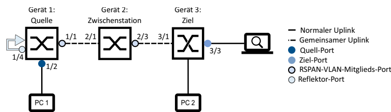
Abb. 127: RSPAN in einer Linien-Topologie, mittels Reflektor-Port (mit gemeinsamen Uplinks)
