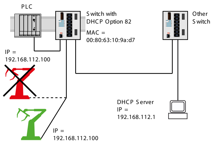
Abb. 154: Anwendungsbeispiel für den Einsatz von Option 82
