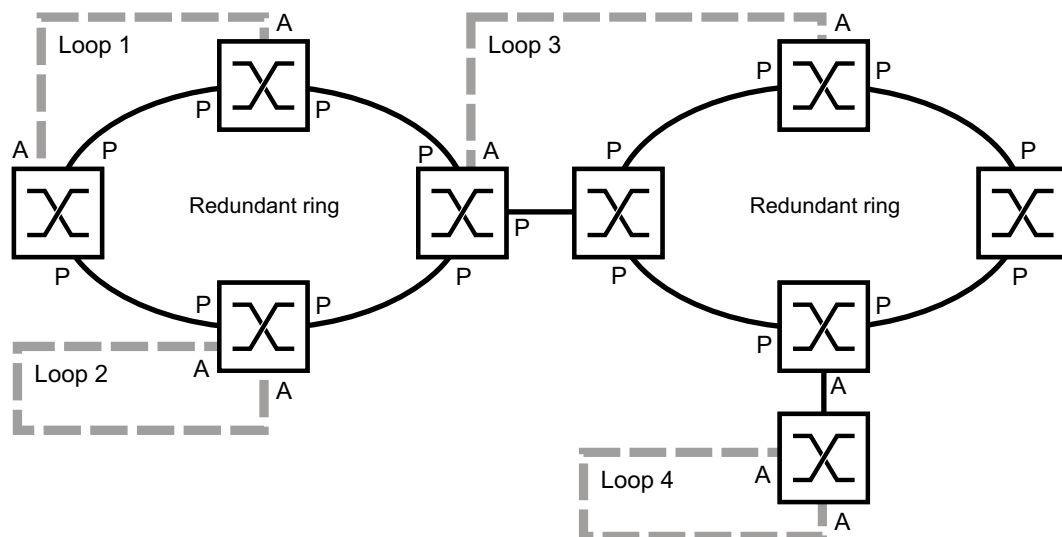
Abb. 118: Beispiele für unbeabsichtigte Schicht-2-Loops
