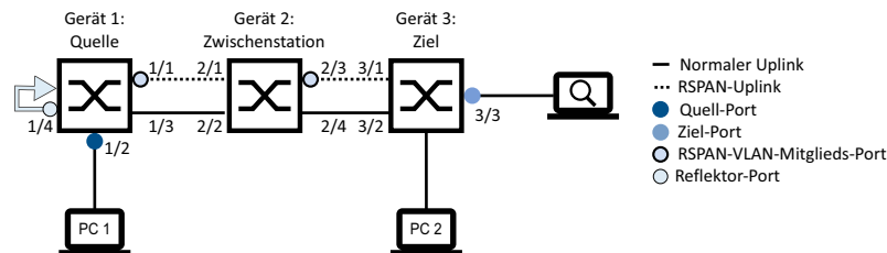
Abb. 126: RSPAN in einer Linien-Topologie, mittels Reflektor-Port (mit separaten Uplinks)
