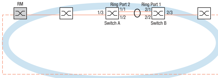
Abb. 43: Anwendungsbeispiel für ein MRP-über-LAG-Setup
