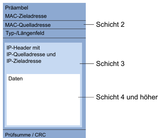
Abb. 83: Aufbau eines Datenpaketes aus Sicht des ISO/OSI-Referenzmodells
