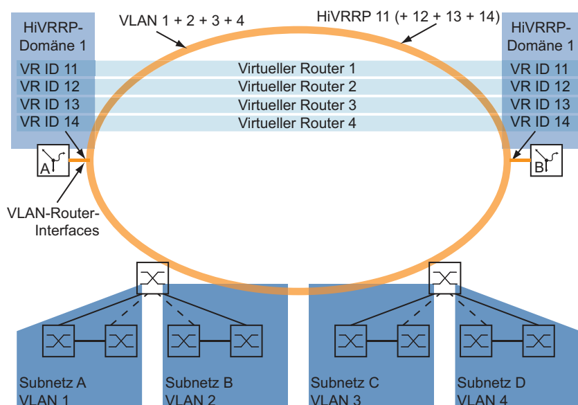
Abb. 95: Beispiel für die Anwendung einer HiVRRP-Domäne
