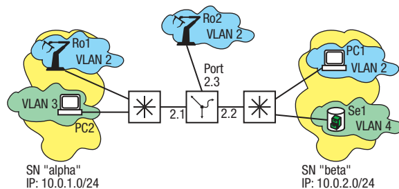
Abb. 107: Anwendungsbeispiel für ein Protokoll-basiertes VLAN
