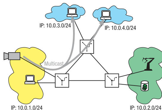
Abb. 108: Beispiel für eine Multicast-Anwendung
