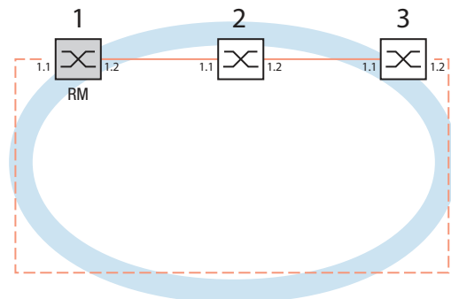
Abb. 39: Beispiel für einen MRP-Ring RM = Ring-Manager — Hauptleitung - - - redundante Leitung
