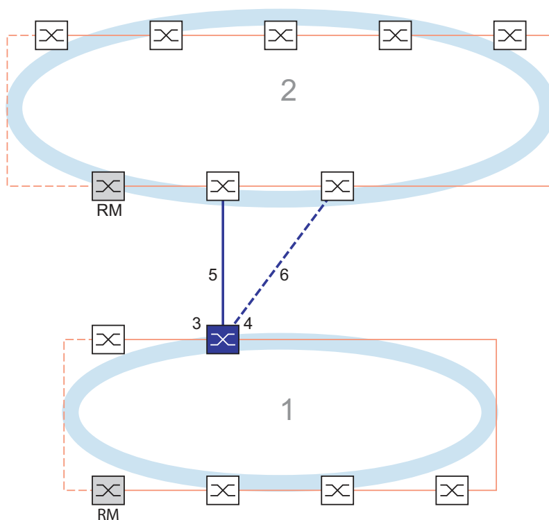
Abb. 70: Beispiel für die 1-Switch-Kopplung
