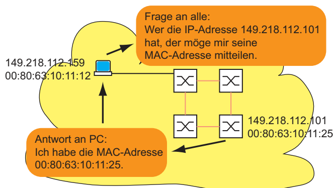
Abb. 82: ARP-Anfrage und -Antwort
