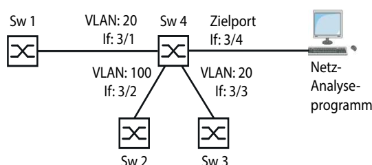
Abb. 120: Anwendungsbeispiel für ein VLAN-Mirroring-Setup
