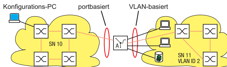
Abb. 86: Statische Routen: Beispiel für eine Verbindung zwischen zwei Fertigungszellen.
