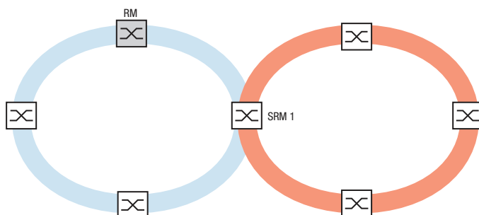
Abb. 59: Sonderfall: Ein Sub-Ring-Manager-Gerät verwaltet beide Enden eines Sub-Rings an unterschiedlichen Ports (Single-Sub-Ring-Manager).
