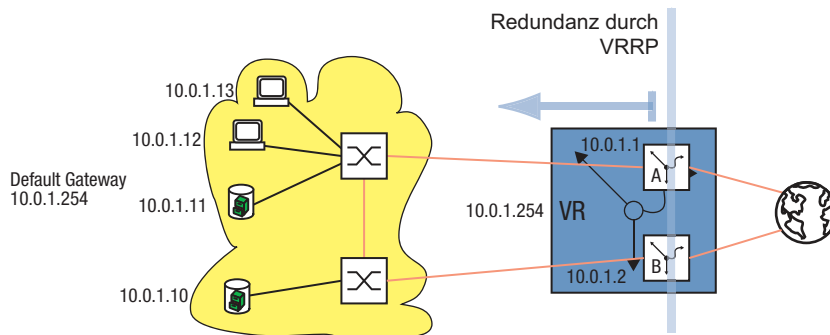
Abb. 91: Darstellung des virtuellen Routers
