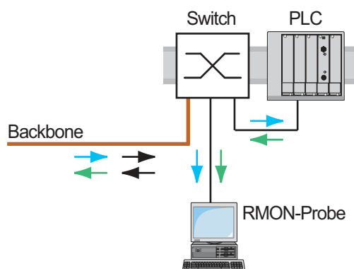
Abb. 119: Anwendungsbeispiel für ein Port-Mirroring-Setup
