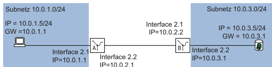
Abb. 100: Anwendungsbeispiel für ein RIP-Setup
