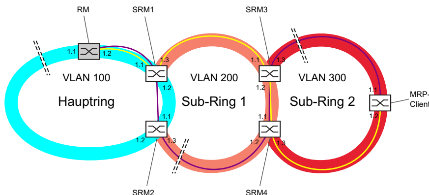
Abb. 61: Beispiel einer Struktur kaskadierter Sub-Ringe
