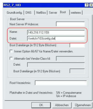
Abb. 143: Konfigurationsdatei auf dem tftp-Server
