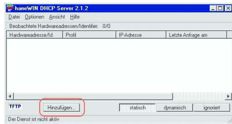
Abb. 145: Statische Adressen hinzufügen
