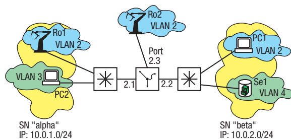
Abb. 107: Anwendungsbeispiel für ein Protokoll-basiertes VLAN
