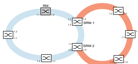
Abb. 56: Beispiel für eine Sub-Ring-Struktur blauer Ring = Hauptring orangefarbener Ring = Sub-Ring SRM = Sub-Ring-Manager RM = Ring-Manager
