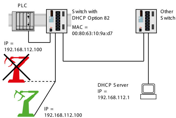
Abb. 153: Anwendungsbeispiel für den Einsatz von Option 82
