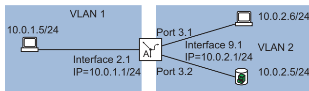
Abb. 88: VLAN-basiertes Router-Interface
