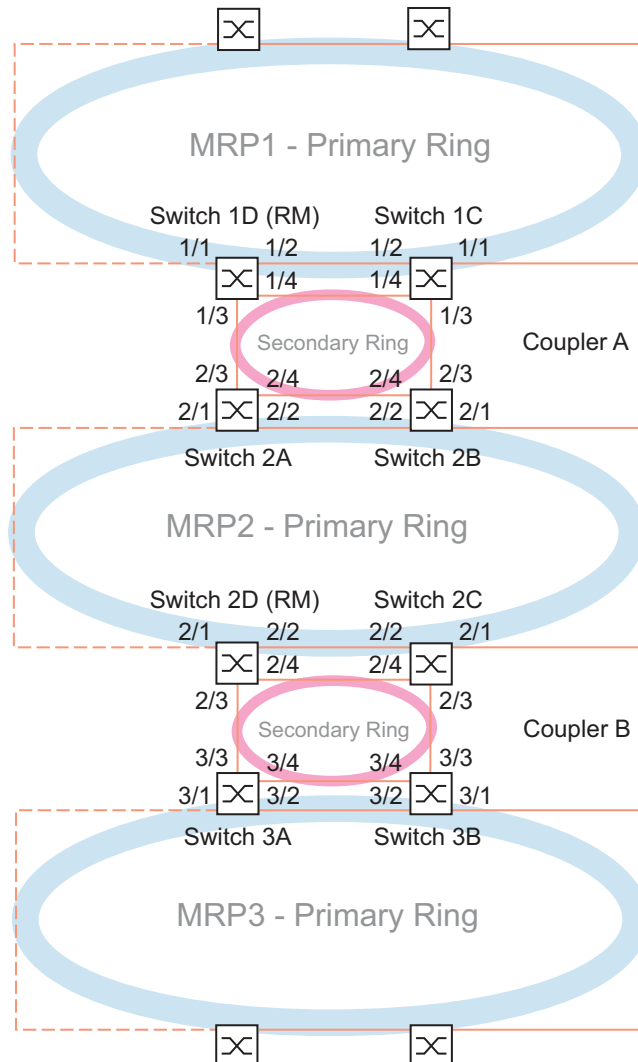
Abb. 79: Redundant Coupling Protocol-Zugtopologie:
