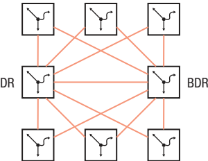
Abb. 105: LSA-Verteilung mit Designated-Router und Backup-Designated-Router
