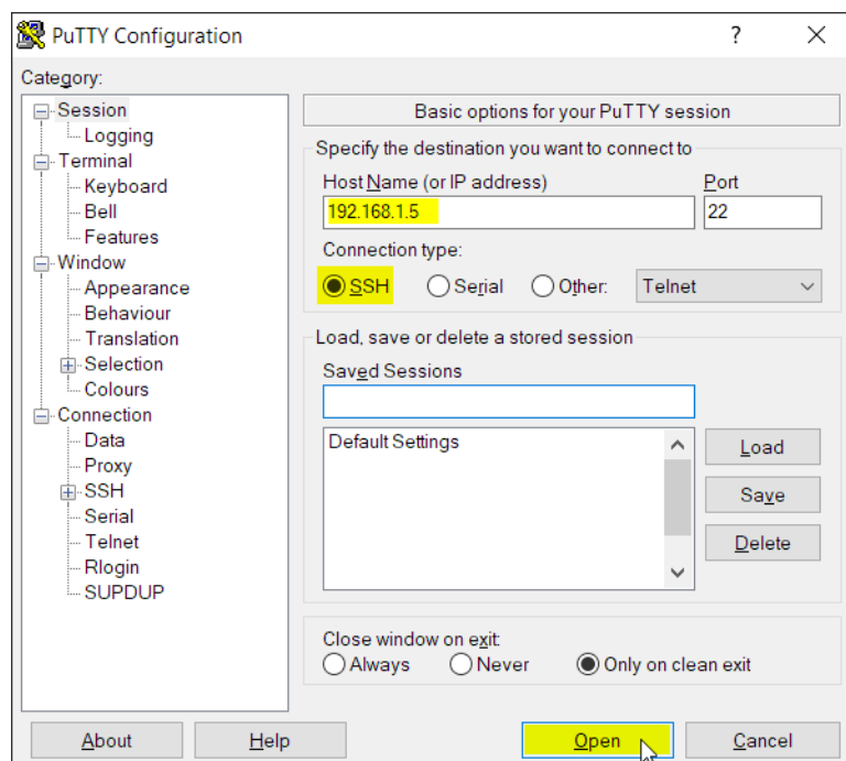
Abb. 154: PuTTY-Eingabemaske
