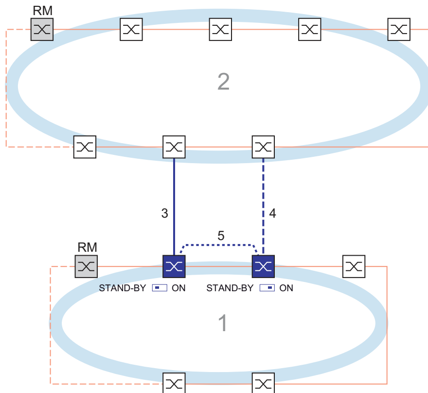
Abb. 75: Beispiel für die 2-Switch-Kopplung mit Steuerleitung 1: Ring 2: Backbone 3: Hauptleitung 4: Redundante Leitung 5: Steuerleitung
