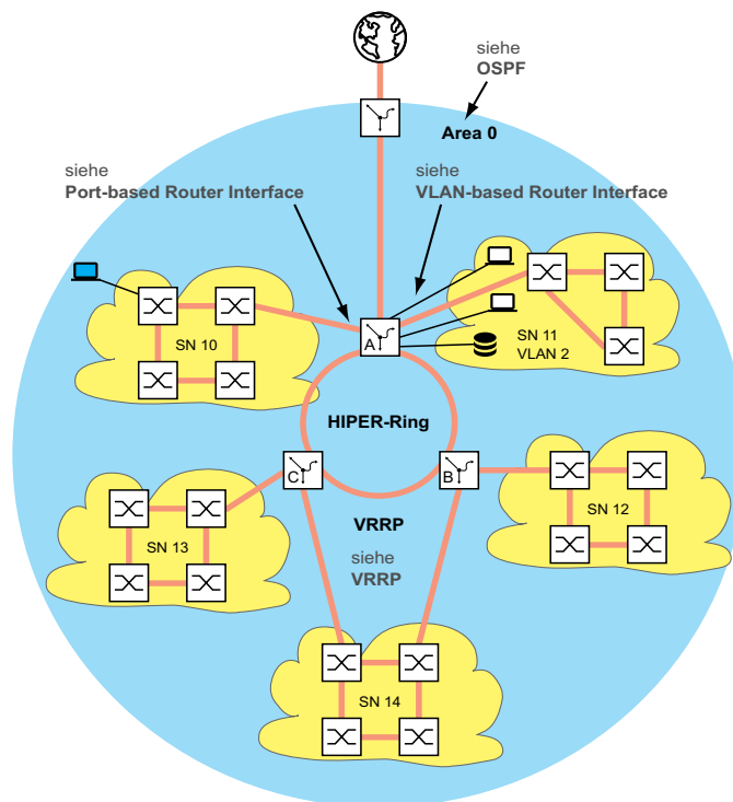
Abb. 110: Netzplan
