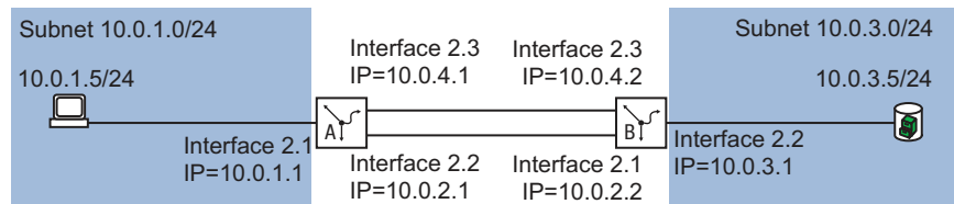
Abb. 90: Redundante statische Route
