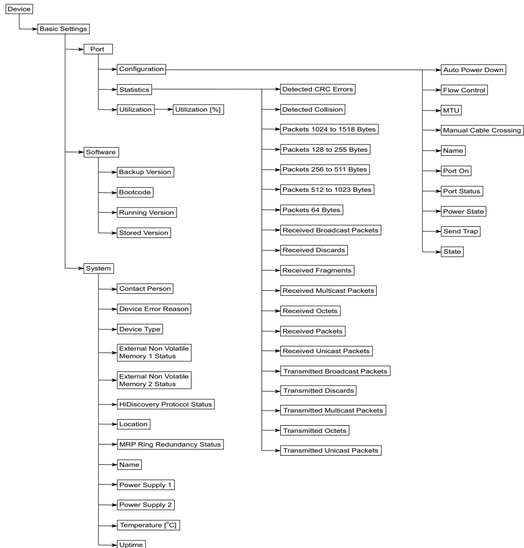
Abb. 136: OPC UA-Informationsmodell
