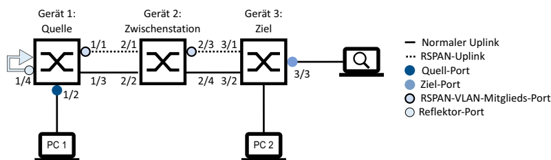
Abb. 126: RSPAN in einer Linien-Topologie, mittels eines Reflektor-Ports (mit separaten Uplinks)
