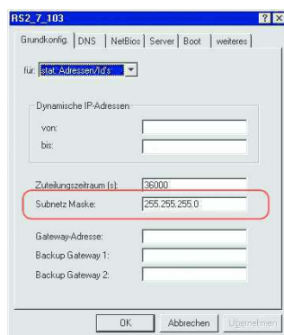
Abb. 141: Netzmaske im Konfigurationsprofil
