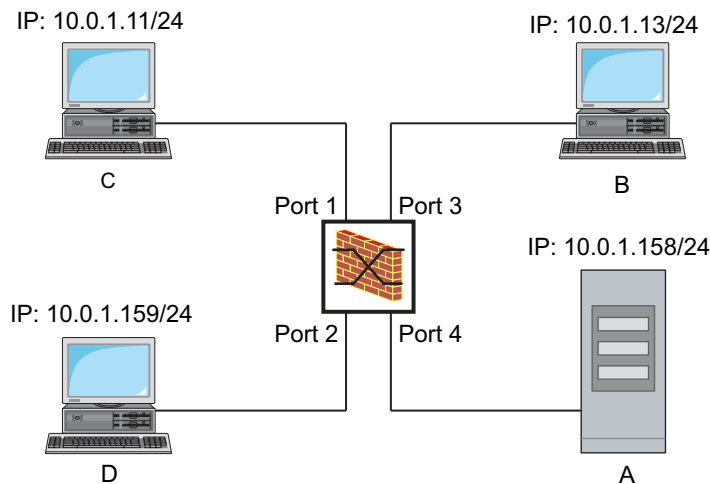
Abb. 23: Anwendungsbeispiel für eine IP-ACL
