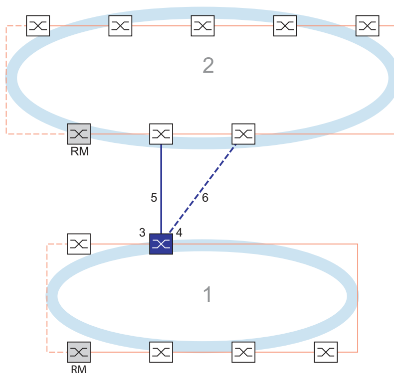
Abb. 70: Beispiel für die 1-Switch-Kopplung 1: Ring 2: Backbone 3: Partner-Kopplungs-Port 4: Kopplungs-Port 5: Hauptleitung 6: Redundante Leitung
