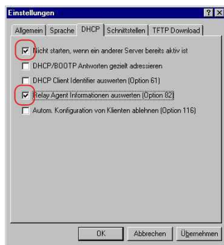
Abb. 149: DHCP-Einstellung
