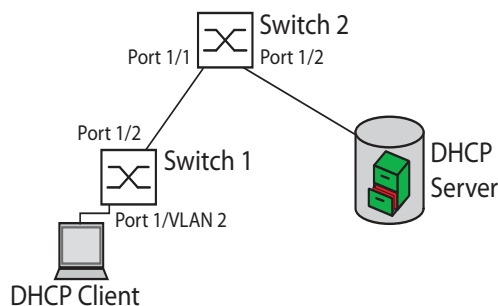
Abb. 130: Beispiel: DHCP-Schicht-2-Netz
