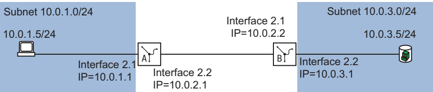
Abb. 89: Statisches Routing
