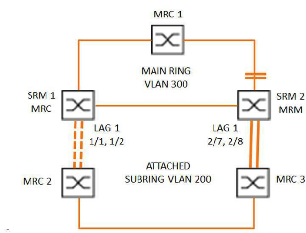
Abb. 62: Sub-Ring mit Link-Aggregation
