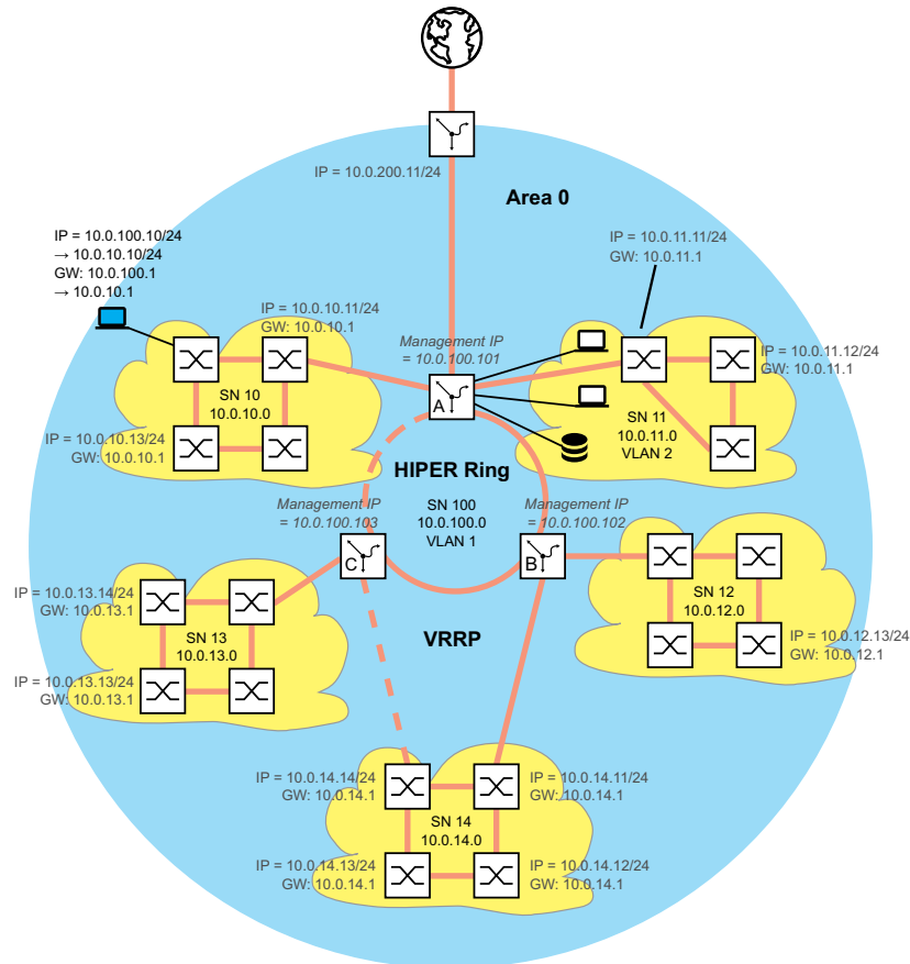
Abb. 111: Netzplan mit Management-IP-Adressen
