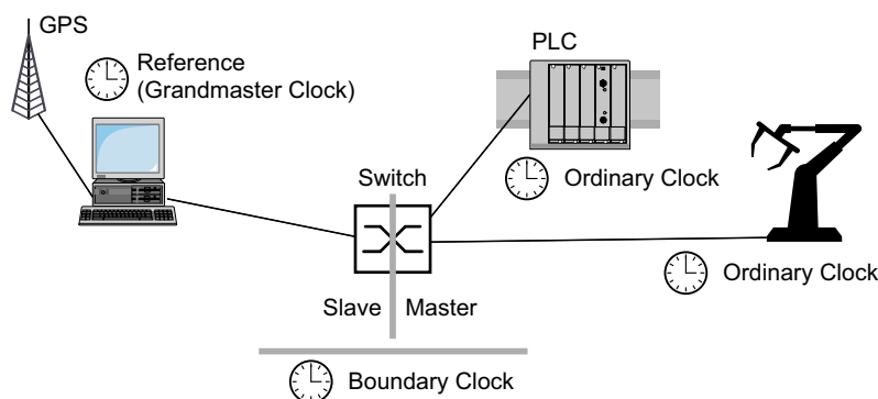
Abb. 15: Position der Boundary-Clock in einem Netz
