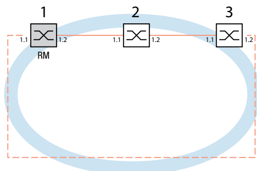
Abb. 28: Beispiel für einen MRP-Ring RM = Ring-Manager — Hauptleitung - - - redundante Leitung
