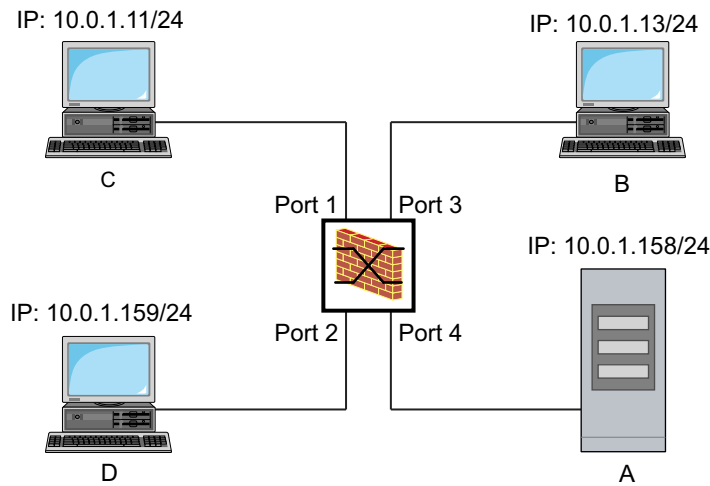
Abb. 17: Anwendungsbeispiel für eine IP-ACL
