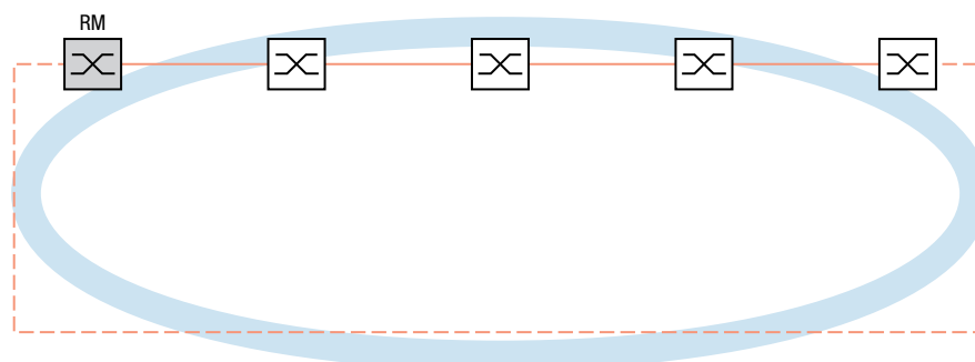
Abb. 27: Redundante Ringstruktur RM = Ring-Manager — Hauptleitung - - - redundante Leitung
