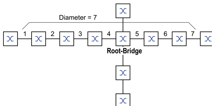
Abb. 32: Definition „Diameter“
