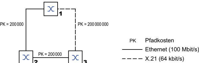
Abb. 30: Pfadkosten
