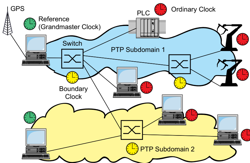
Abb. 16: Beispiel für PTP-Domänen
