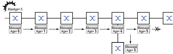
Abb. 33: Übertragung einer STP-BPDU abhängig von MaxAge
