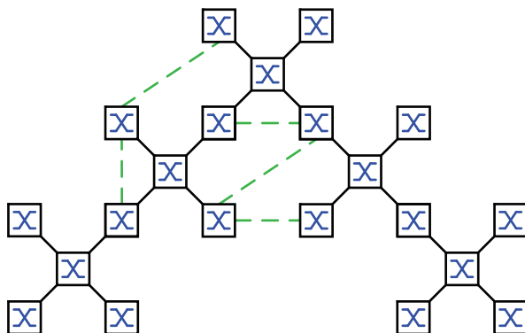
Abb. 24: Maschen-Topologie: Baum-Topologie mit physischen Schleifen
