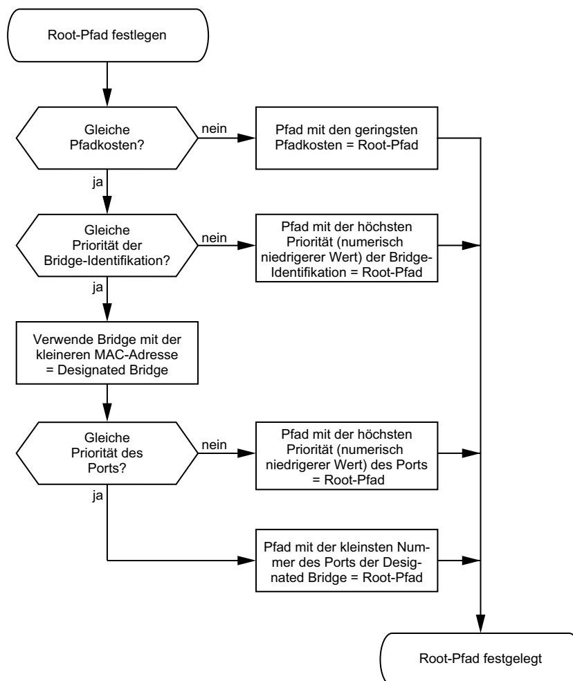
Abb. 34: Flussdiagramm Root-Pfad festlegen
