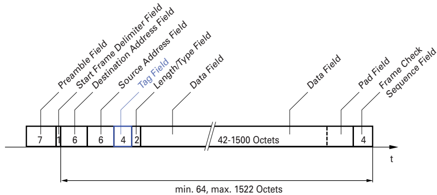
Abb. 18: Ethernet-Datenpaket mit Tag
