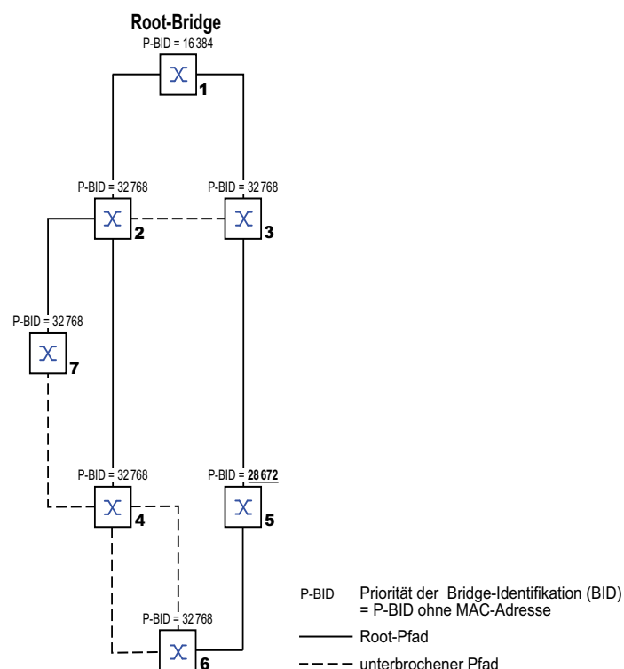
Abb. 36: Beispiel eines Netzplans für die Manipulation des Root-Pfads
