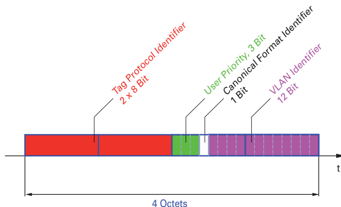
Abb. 19: Aufbau des VLAN-Tag
