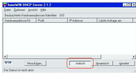
Abb. 59: Statische Adresseingabe
