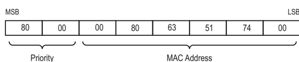
Abb. 33: Bridge-Identifikation, Beispiel (Interpretation nach IEEE 802.1D-1998, Werte in Hexadezimalschreibweise)
