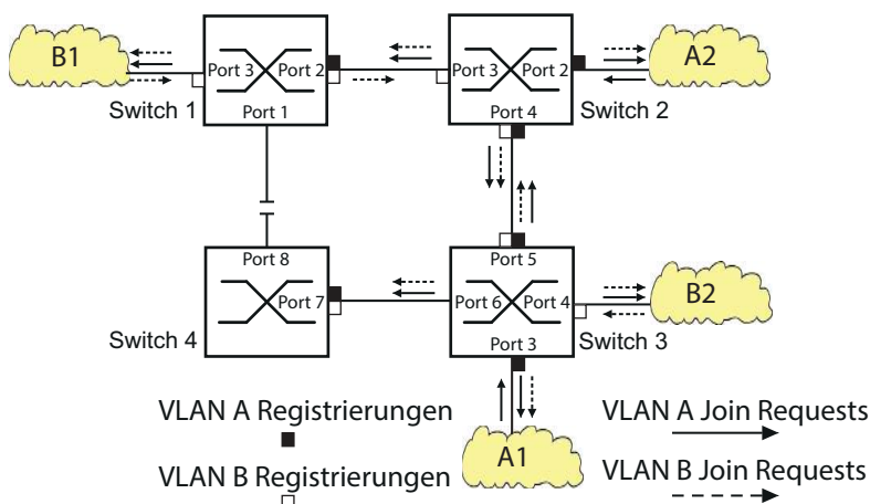
Abb. 49: MVRP -Beispiel-Netz für VLAN-Registrierung
