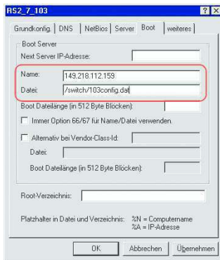
Abb. 57: Konfigurationsdatei auf dem tftp-Server
