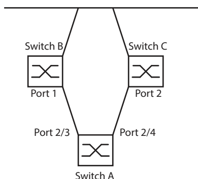
Abb. 44: Link-Backup Beispiel-Netzwerk
