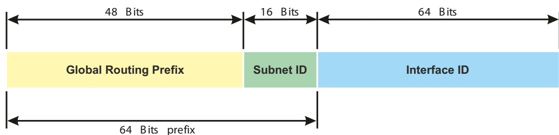
Abb. 13: Allgemeines Format der IPv6-Global-Unicast-Adresse
