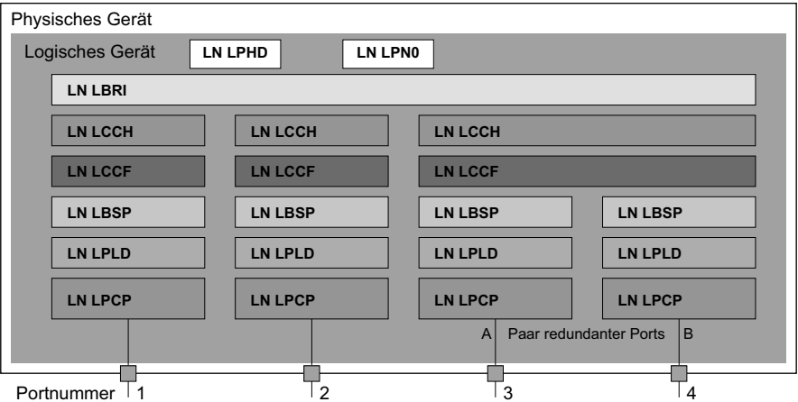
Abb. 95: Bridge-Modell nach Technical Report IEC 61850 90-4
