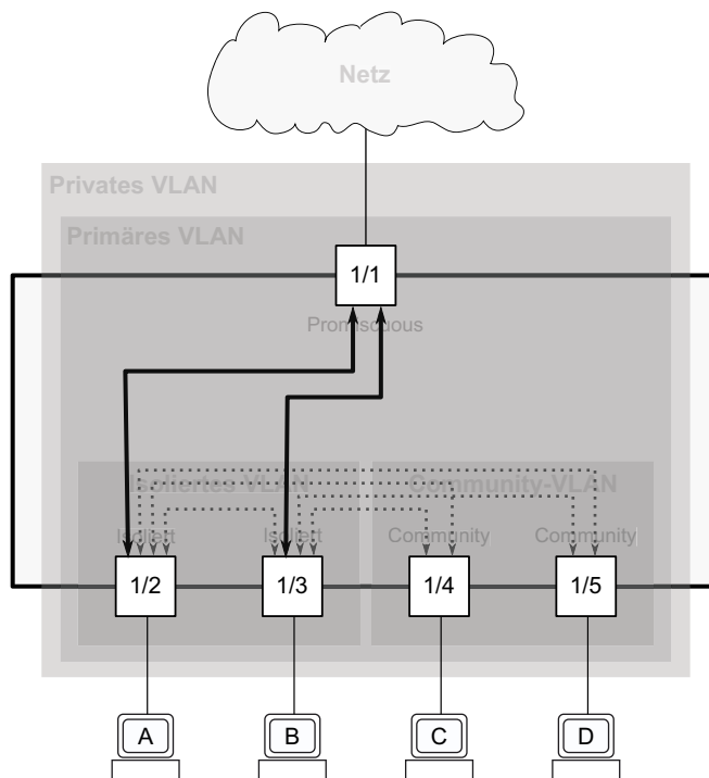
Abb. 26: Kommunikationsfluss der isolierten Ports
