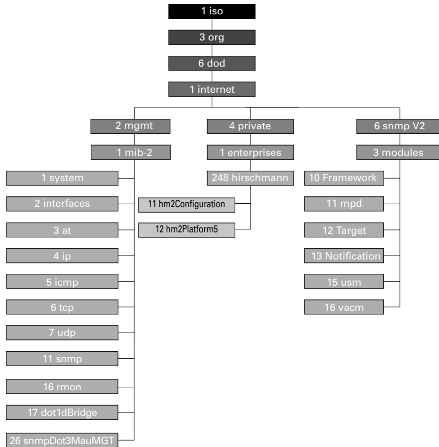
Abb. 115: Baumstruktur der Hirschmann-MIB
