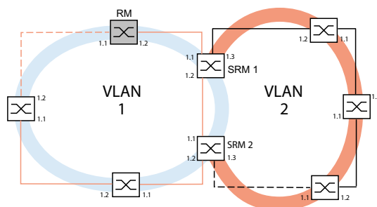
Abb. 57: Beispiel für eine Sub-Ring-Struktur mit VLANs orangefarbene Linie= Mitglieder des Hauptrings in VLAN 1 schwarze Linie= Mitglieder des Sub-Rings in VLAN 2 orange gestrichelte Linie= unterbrochenes Segment im Hauptring schwarz gestrichelte Linie= unterbrochenes Segment im Sub-Ring SRM = Sub-Ring-Manager RM = Ring-Manager
