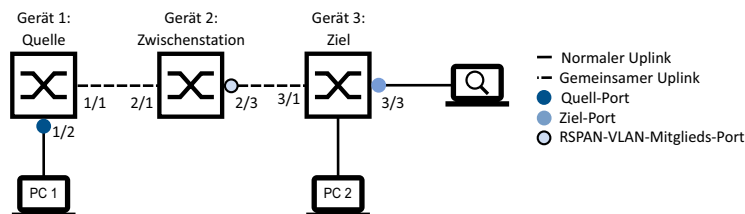
Abb. 89: RSPAN in einer Linien-Topologie, ohne einen Reflektor-Port (mit gemeinsamen Uplinks)
