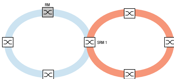
Abb. 56: Sonderfall: Ein Sub-Ring-Manager-Gerät verwaltet beide Enden eines Sub-Rings an unterschiedlichen Ports (Single-Sub-Ring-Manager).
