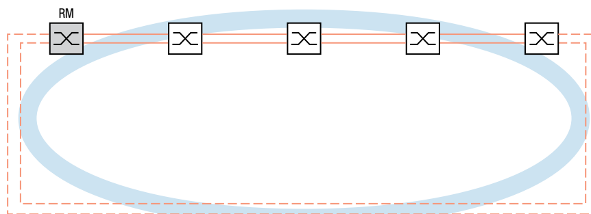
Abb. 36: Link-Aggregation für den gesamten MRP-Ring
