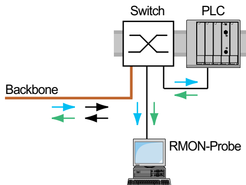
Abb. 79: Anwendungsbeispiel für ein Port-Mirroring-Setup
