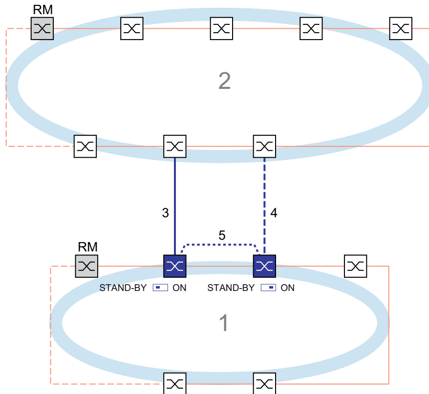
Abb. 72: Beispiel für die 2-Switch-Kopplung mit Steuerleitung
