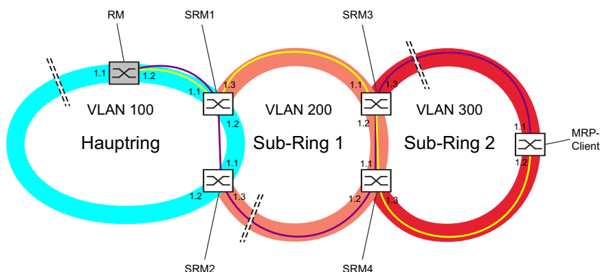
Abb. 58: Beispiel einer Struktur kaskadierter Sub-Ringe
