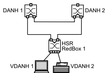
Abb. 39: VDANH mit einem HSR-Netz verbinden
