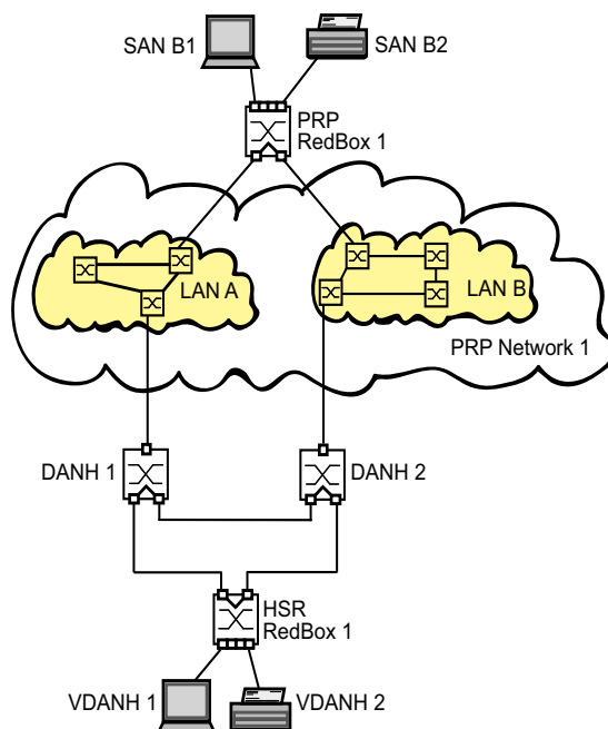
Abb. 40: PRP-Netz mit einem HSR-Netz verbinden
