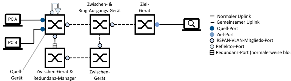
Abb. 85: Beispiel für eine einfache Ring-Topologie auf der Grundlage eines bestehenden redundanten Rings (mit gemeinsamen Links)
