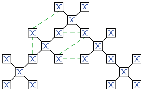
Abb. 30: Maschen-Topologie: Baum-Topologie mit physischen Schleifen
