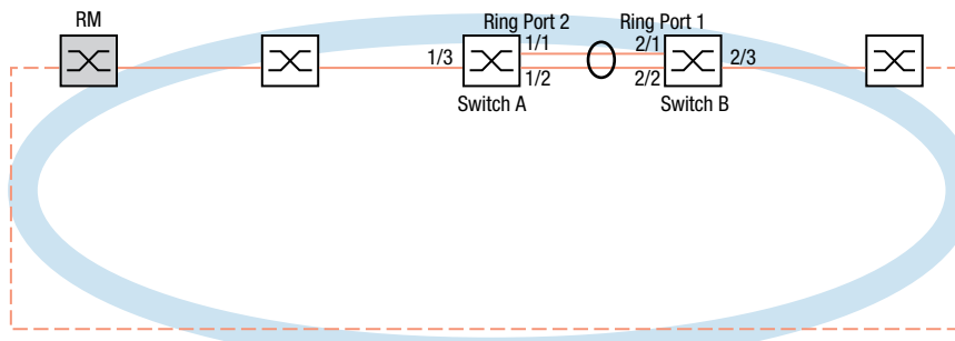
Abb. 38: Anwendungsbeispiel für ein MRP-über-LAG-Setup
