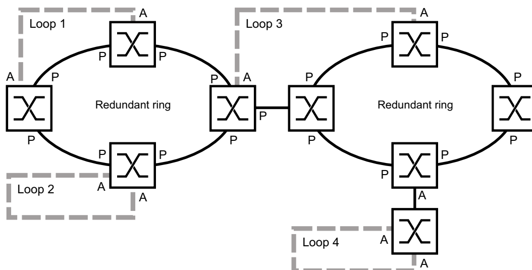
Abb. 78: Beispiele für unbeabsichtigte Schicht-2-Loops
