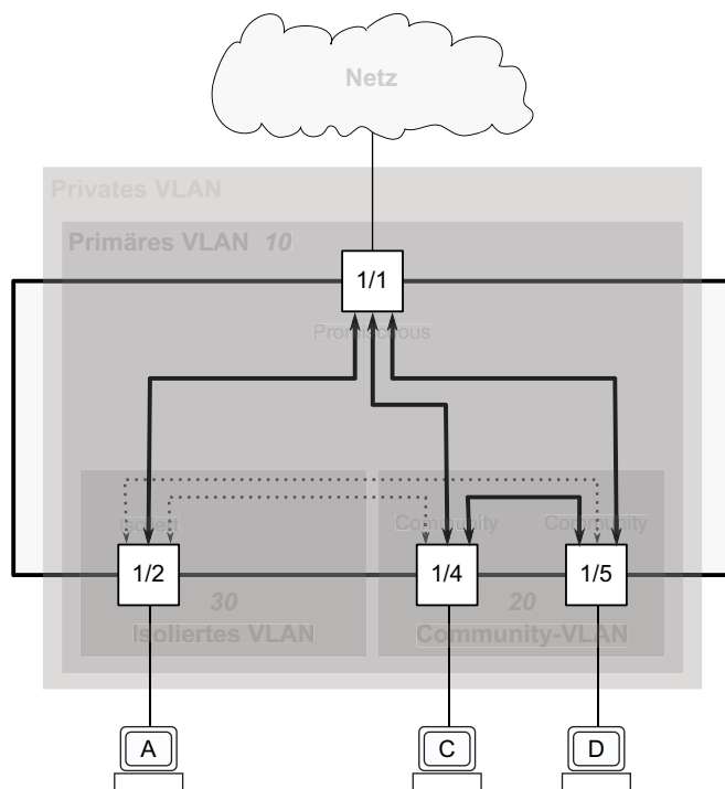
Abb. 28: Beispiel für ein privates VLAN
