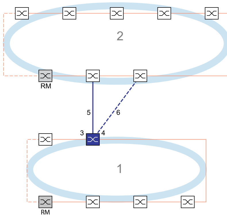
Abb. 60: Beispiel für die 1-Switch-Kopplung
