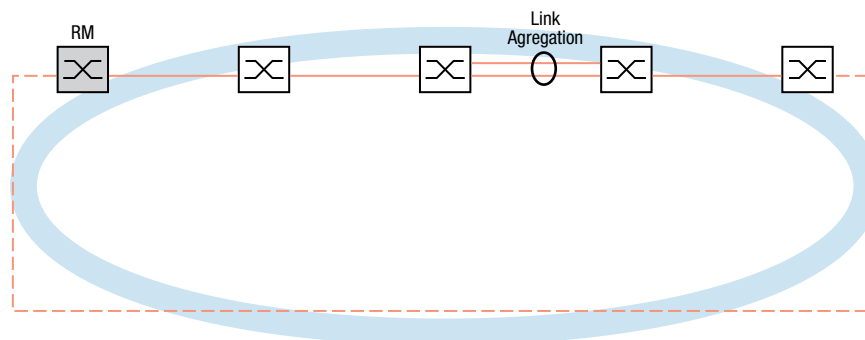
Abb. 35: Link-Aggregation über eine einzelne Verbindung eines MRP-Rings
