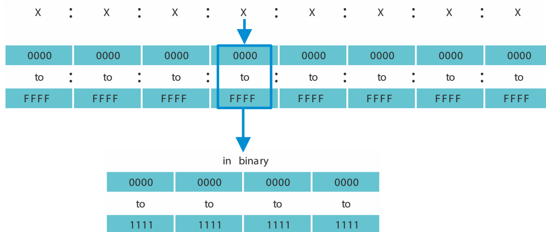
Abb. 8: Darstellung der IPv6-Adresse
