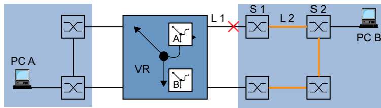
Abb. 77: Überwachen einer Leitung mit Interface-Tracking
