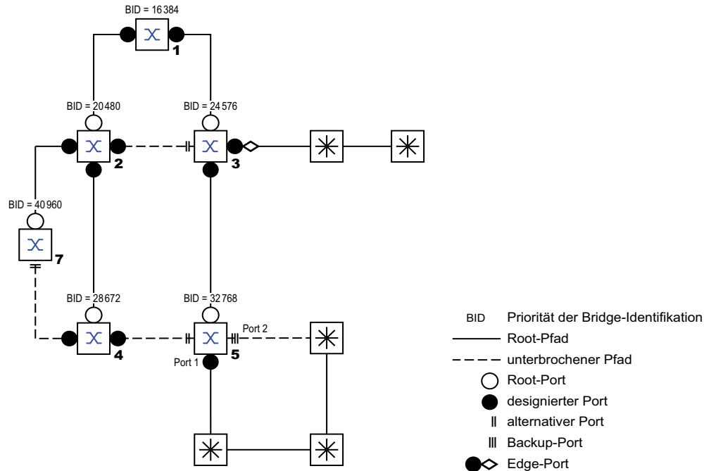
Abb. 50: Port-Rollen-Zuweisung
