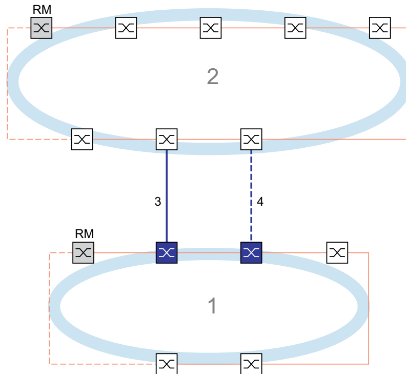
Abb. 61: Beispiel für die 2-Switch-Kopplung 1: Ring 2: Backbone 3: Hauptleitung 4: Redundante Leitung
