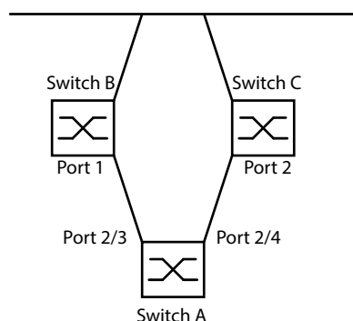
Abb. 52: Link-Backup Beispiel-Netzwerk
