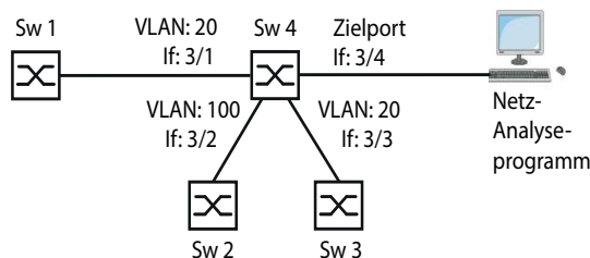
Abb. 80: Anwendungsbeispiel für ein VLAN-Mirroring -Setup
