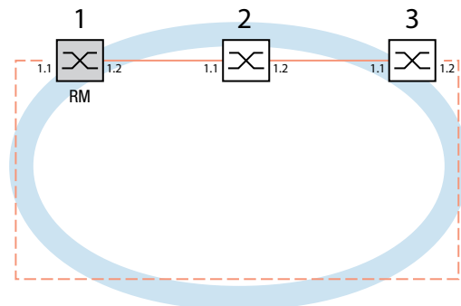
Abb. 34: Beispiel für einen MRP-Ring RM = Ring-Manager — Hauptleitung - - - redundante Leitung
