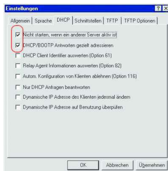
Abb. 100: DHCP-Einstellung
