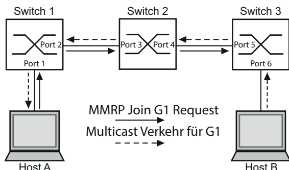
Abb. 92: MMRP -Netz für MAC-Adressen-Registrierung
