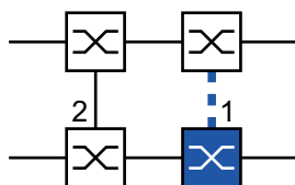
Abb. 71: 2-Switch-Kopplung, Standby-Gerät 1: Kopplungs-Port 2: Partner-Kopplungs-Port
