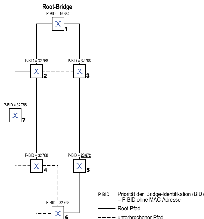
Abb. 48: Beispiel eines Netzplans für die Manipulation des Root-Pfads
