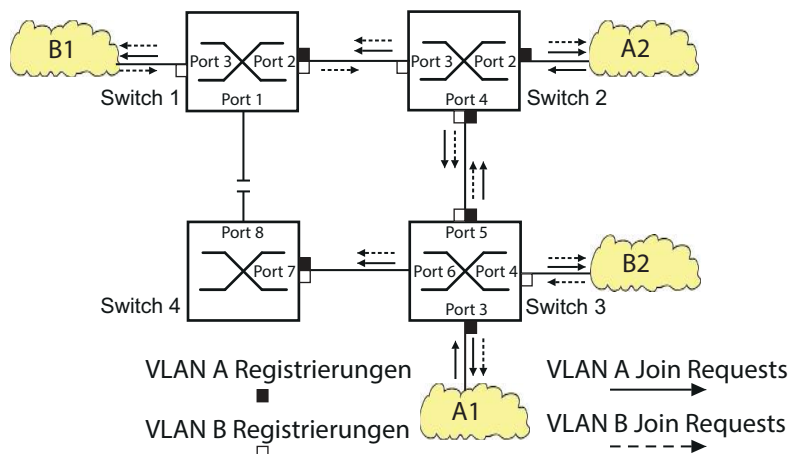
Abb. 94: MVRP-Beispiel-Netz für VLAN-Registrierung
