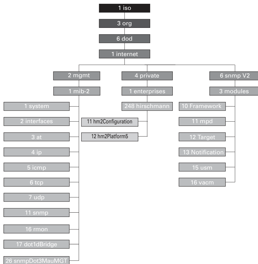
Abb. 118: Baumstruktur der Hirschmann-MIB
