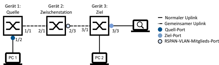
Abb. 91: RSPAN in einer Linien-Topologie, ohne einen Reflektor-Port (mit gemeinsamen Uplinks)
