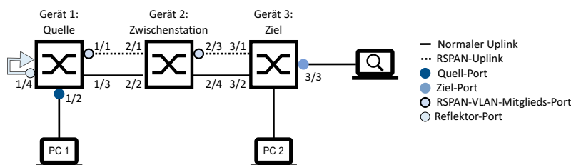
Abb. 88: RSPAN in einer Linien-Topologie, mittels eines Reflektor-Ports (mit separaten Uplinks)
