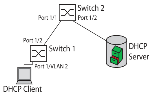
Abb. 92: Beispiel: DHCP-Schicht-2-Netz
