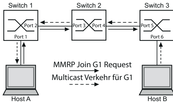
Abb. 93: MMRP -Netz für MAC-Adressen-Registrierung
