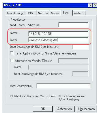
Abb. 104: Konfigurationsdatei auf dem tftp-Server
