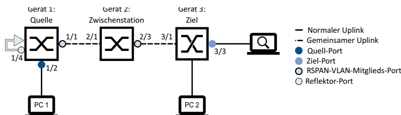
Abb. 89: RSPAN in einer Linien-Topologie, mittels eines Reflektor-Ports (mit gemeinsamen Uplinks)
