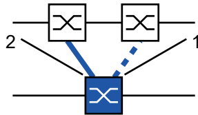
Abb. 67: 1-Switch-Kopplung 1: Kopplungs-Port 2: Partner-Kopplungs-Port
