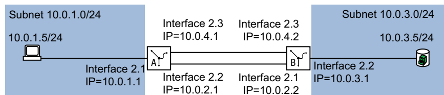
Abb. 86: Redundante statische Route
