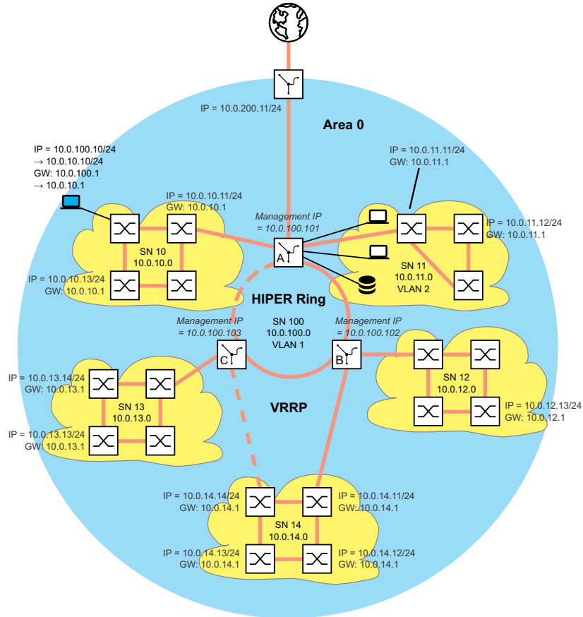
Abb. 107: Netzplan mit Management-IP-Adressen
