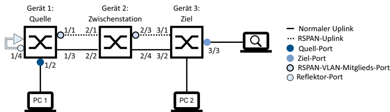
Abb. 122: RSPAN in einer Linien-Topologie, mittels Reflektor-Port (mit separaten Uplinks)
