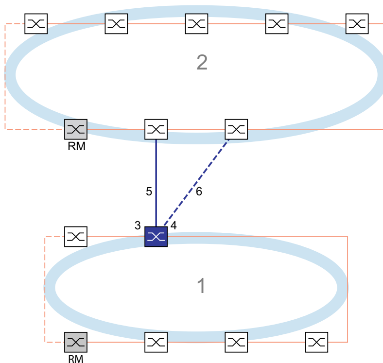
Abb. 66: Beispiel für die 1-Switch-Kopplung
