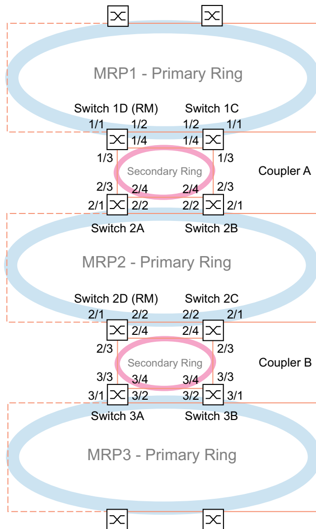
Abb. 75: Redundant Coupling Protocol-Zugtopologie: - Ports x/1 und x/2 sind MRP -Ring-Ports - Ports x/3 sind äußere RCP -Ports - Ports x/4 sind innere RCP -Ports
