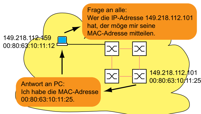
Abb. 78: ARP-Anfrage und -Antwort
