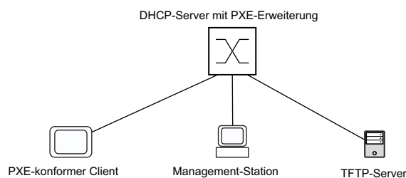
Abb. 126: Einfacher Aufbau eines Preboot eXecution Environment (PXE)-Setups
