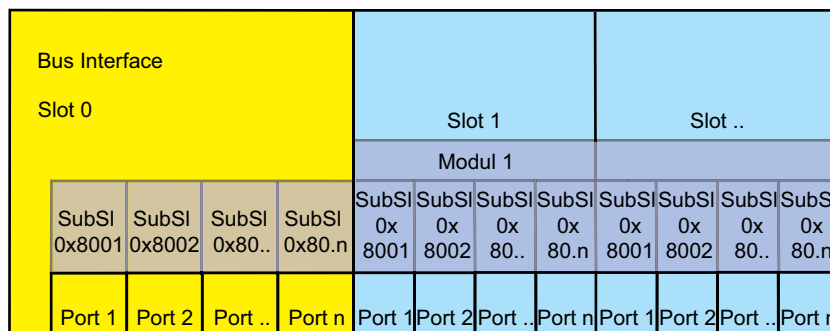
Abb. 139: Kombigerät
