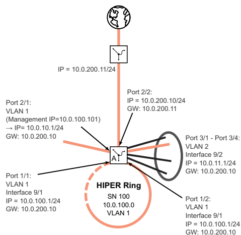
Abb. 108: IP-Parameter für Schicht-3-Gerät A
