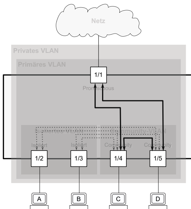
Abb. 28: Kommunikationsfluss der Community-Ports
