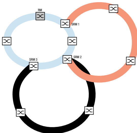
Abb. 54: Sonderfall: Ein Sub-Ring-Manager-Gerät verwaltet 2 Sub-Ringe (2 Instanzen). Das Sub-Ring-Manager-Gerät ist in der Lage, bis zu 20 Instanzen zu verwalten.
