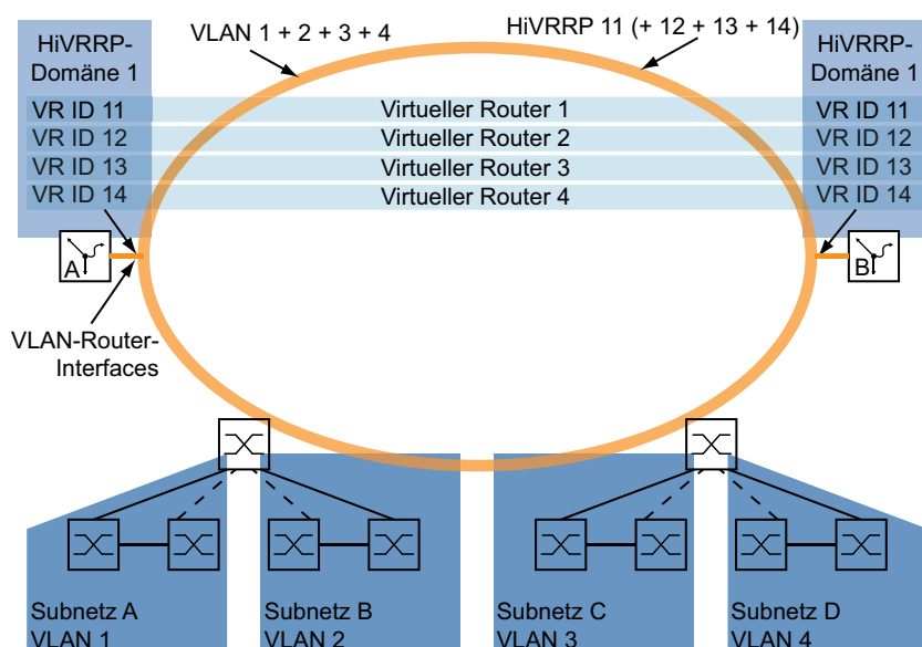
Abb. 91: Beispiel für die Anwendung einer HiVRRP-Domäne
