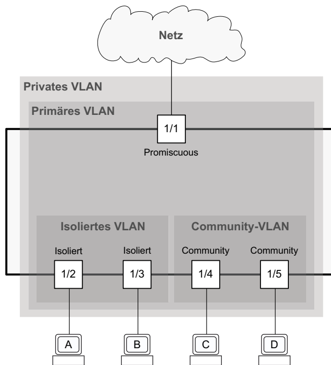
Abb. 26: Aufbau eines privaten VLANs
