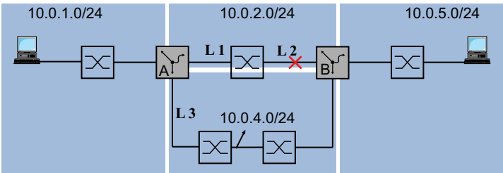
Abb. 112: Beispiel für statisches Route-Tracking
