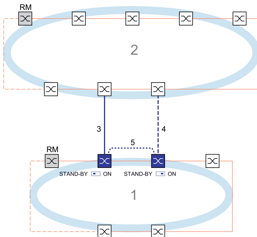
Abb. 71: Beispiel für die 2-Switch-Kopplung mit Steuerleitung
