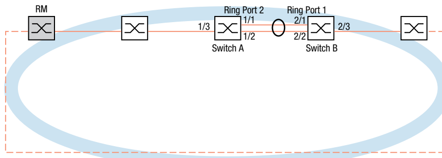
Abb. 39: Anwendungsbeispiel für ein MRP-über-LAG-Setup
