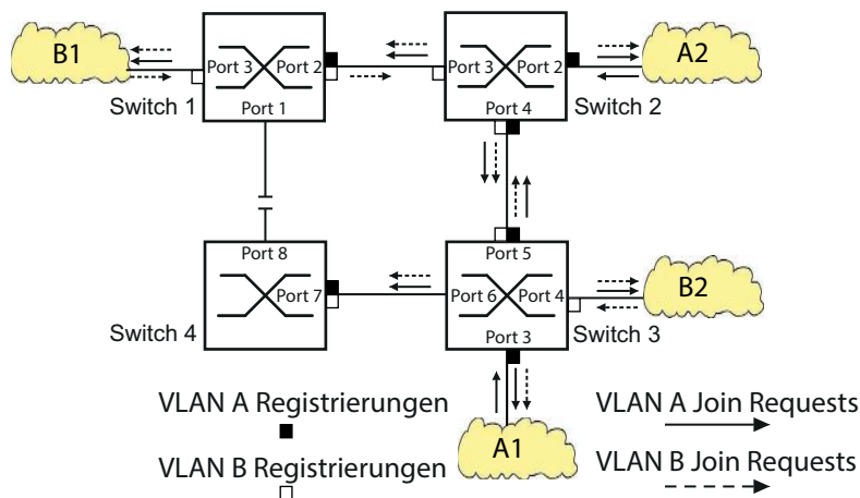
Abb. 129: MVRP -Beispiel-Netz für VLAN-Registrierung
