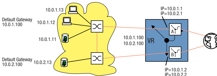
Abb. 93: Virtueller Router mit Multinetting
