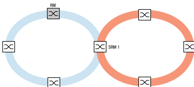
Abb. 55: Sonderfall: Ein Sub-Ring-Manager-Gerät verwaltet beide Enden eines Sub-Rings an unterschiedlichen Ports (Single-Sub-Ring-Manager).
