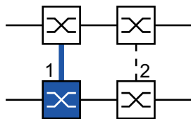
Abb. 69: 2-Switch-Kopplung, primäres Gerät 1: Kopplungs-Port 2: Partner-Kopplungs-Port
