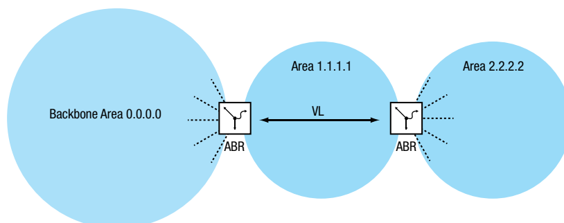
Abb. 99: Anbinden einer entfernten Area an die Backbone Area durch eine virtuelle Verbindung (VL)
