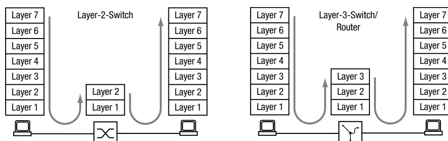
Abb. 76: Datentransport durch einen Switch und einen Router in den Schichten des OSI-Referenzmodells
