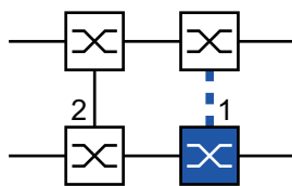
Abb. 70: 2-Switch-Kopplung, Standby-Gerät 1: Kopplungs-Port 2: Partner-Kopplungs-Port
