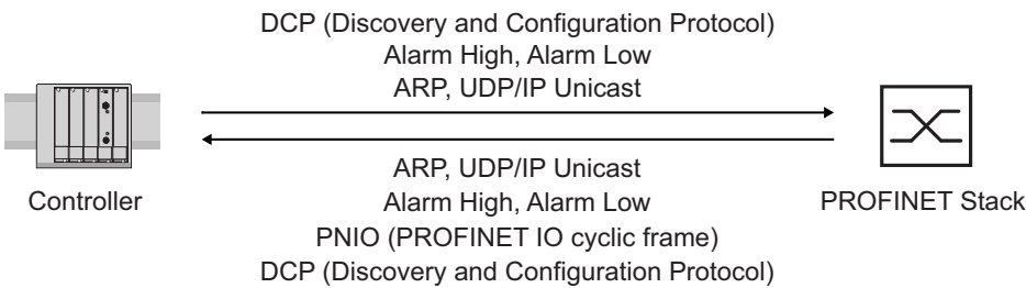
Abb. 136: Kommunikation zwischen Controller und dem Gerät
