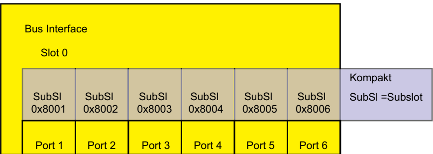
Abb. 137: Kompaktes Gerät
