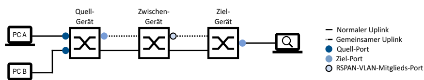
Abb. 118: Beispiel für eine Linien-Topologie, ohne Reflektor-Port (mit separaten Uplinks)
