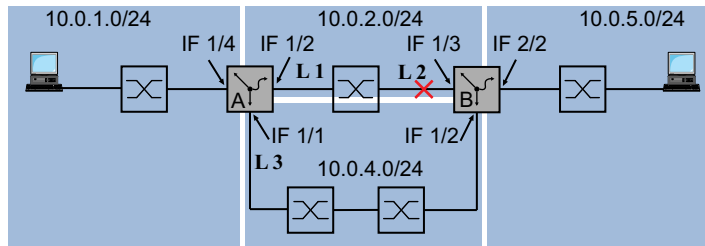
Abb. 113: Statisches Route-Tracking konfigurieren
