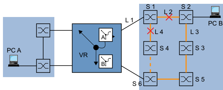
Abb. 111: Überwachen der Erreichbarkeit eines Geräts in einem redundanten Ring
