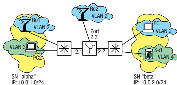
Abb. 103: Anwendungsbeispiel für ein Protokoll-basiertes VLAN
