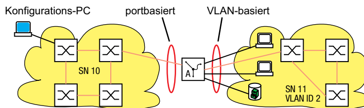
Abb. 82: Statische Routen: Beispiel für eine Verbindung zwischen zwei Fertigungszellen.
