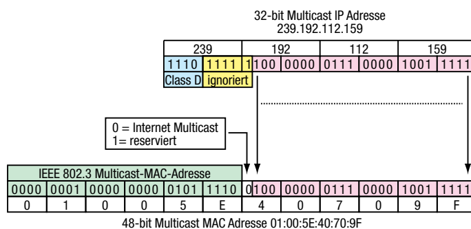
Abb. 105: Umsetzung der IP-Adresse in die MAC-Adresse
