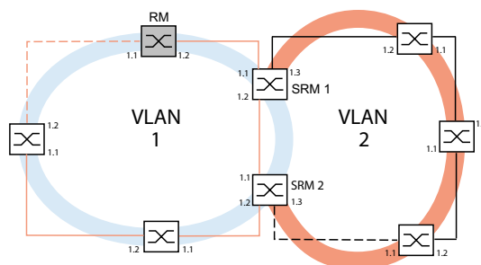
Abb. 56: Beispiel für eine Sub-Ring-Struktur mit VLANs orangefarbene Linie= Mitglieder des Hauptrings in VLAN 1 schwarze Linie= Mitglieder des Sub-Rings in VLAN 2 orange gestrichelte Linie= unterbrochenes Segment im Hauptring schwarz gestrichelte Linie= unterbrochenes Segment im Sub-Ring SRM = Sub-Ring-Manager RM = Ring-Manager
