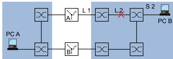
Abb. 110: Überwachen einer Leitung mit Ping-Tracking
