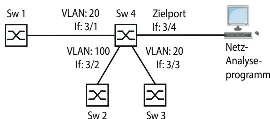
Abb. 116: Anwendungsbeispiel für ein VLAN-Mirroring-Setup
