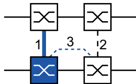
Abb. 72: 2-Switch-Kopplung mit Steuerleitung, primäres Gerät
