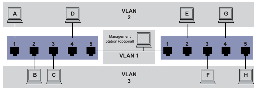
Abb. 29: Beispiel für eine komplexere VLAN-Konfiguration
