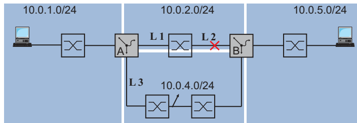
Abb. 90: Beispiel für statisches Route-Tracking
