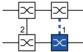
Abb. 65: 2-Switch-Kopplung, Standby-Gerät 1: Kopplungs-Port 2: Partner-Kopplungs-Port
