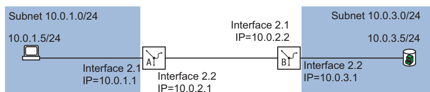
Abb. 88: Statisches Routing
