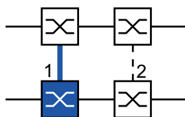
Abb. 72: 2-Switch-Kopplung, primäres Gerät 1: Kopplungs-Port 2: Partner-Kopplungs-Port
