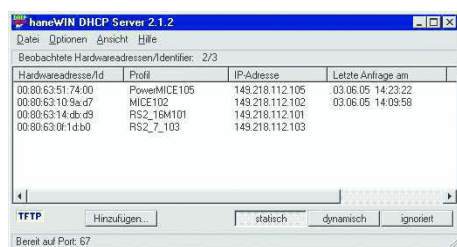
Abb. 56: DHCP-Server mit Einträgen
