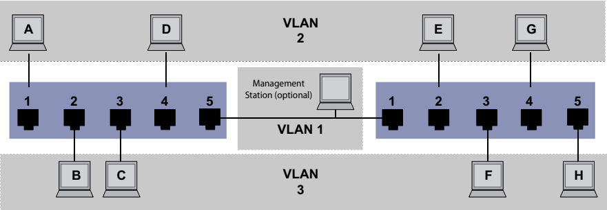
Abb. 20: Beispiel für eine komplexere VLAN-Konfiguration
