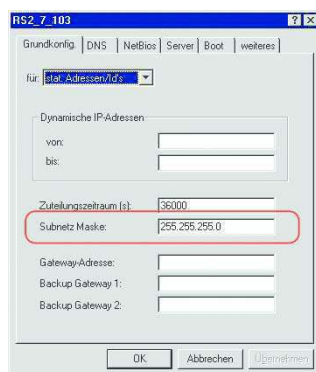
Abb. 50: Netzmaske im Konfigurationsprofil
