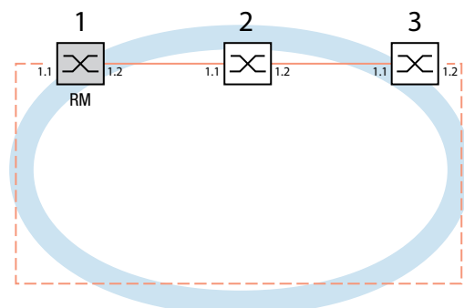
Abb. 26: Beispiel für einen MRP-Ring RM = Ring-Manager — Hauptleitung - - - redundante Leitung
