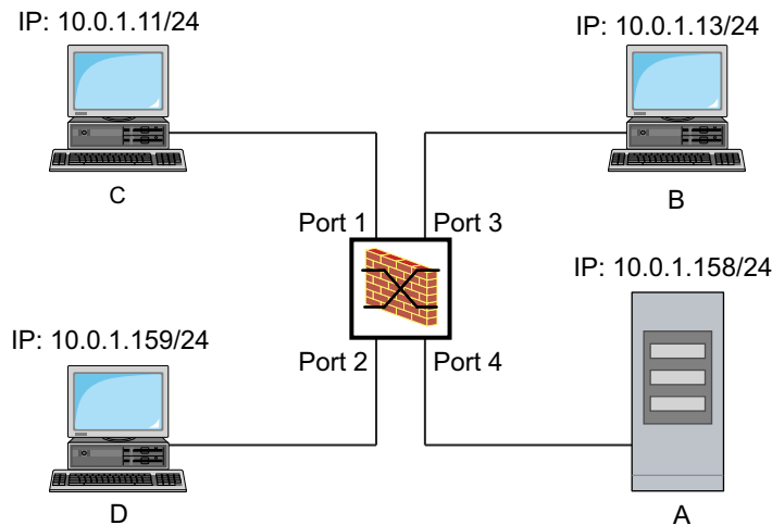
Abb. 15: Anwendungsbeispiel für eine IP-ACL
