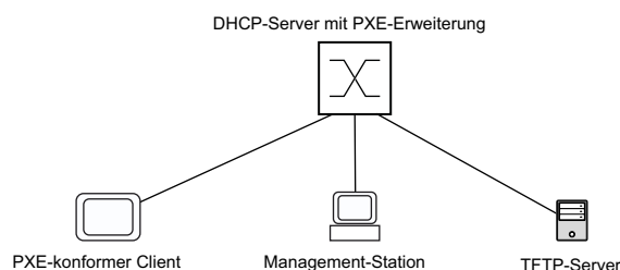
Abb. 40: Einfacher Aufbau eines Preboot eXecution Environment (PXE)-Setups
