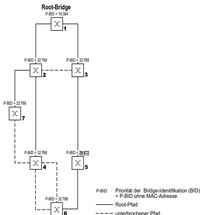
Abb. 34: Beispiel eines Netzplans für die Manipulation des Root-Pfads
