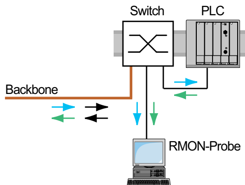
Abb. 39: Anwendungsbeispiel für ein Port-Mirroring-Setup
