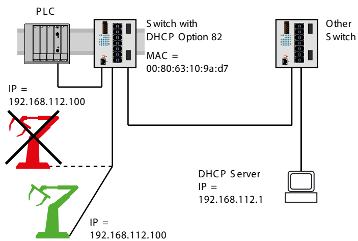
Abb. 62: Anwendungsbeispiel für den Einsatz von Option 82
