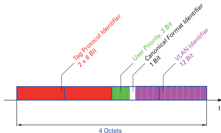
Abb. 17: Aufbau des VLAN-Tag
