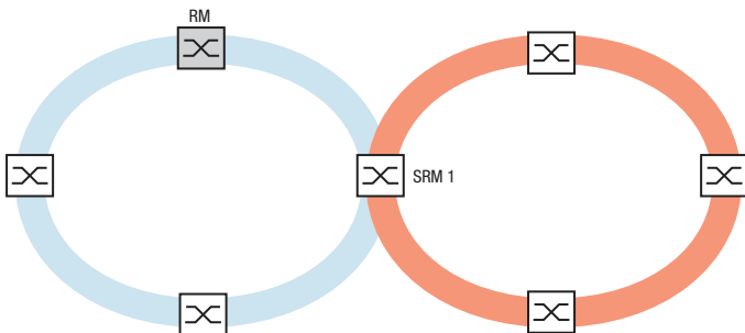
Abb. 48: Sonderfall: Ein Subring-Manager verwaltet beide Enden eines Subrings an unterschiedlichen Ports (Single-Subring-Manager).
