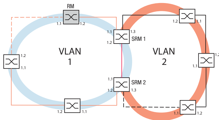
Abb. 49: Beispiel für eine Subring-Struktur orangefarbene Linie = Mitglieder des Hauptrings in VLAN 1 schwarze Linie = Mitglieder des Subrings in VLAN 2 orange gestrichelte Linie = unterbrochenes Segment im Hauptring schwarz gestrichelte Linie = unterbrochenes Segment im Subring rote Linie = redundante Verbindung, Mitglied in VLAN 1 SRM = Subring-Manager RM = Ring-Manager
