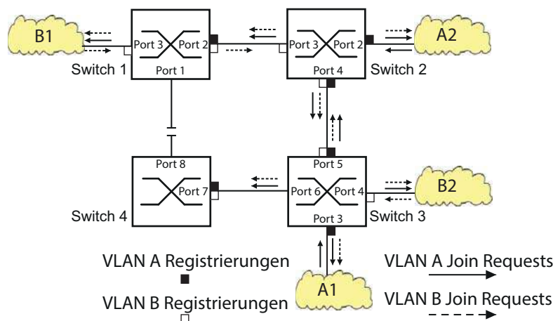
Abb. 53: MVRP -Beispiel-Netz für VLAN-Registrierung
