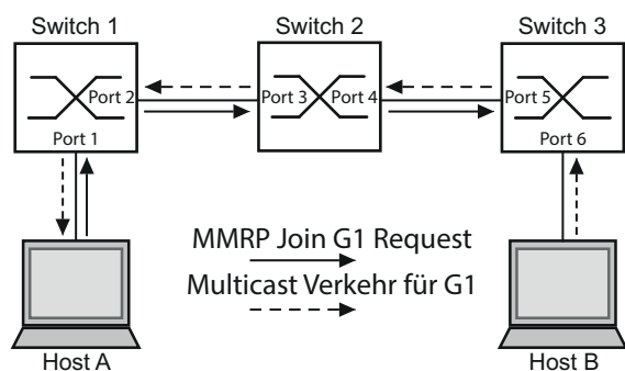
Abb. 52: MMRP -Netz für MAC-Adressen-Registrierung
