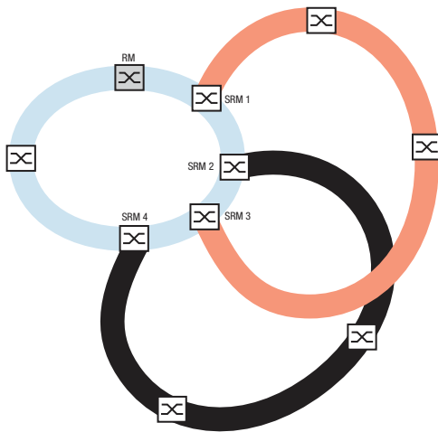
Abb. 46: Beispiel für eine überlappende Subring-Struktur
