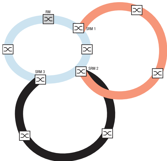
Abb. 47: Sonderfall: Ein Subring-Manager verwaltet 2 Subringe (2 Instanzen). Der Subring-Manager ist in der Lage, bis zu 2 Instanzen zu verwalten.
