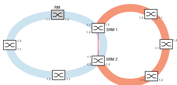
Abb. 45: Beispiel für eine Subring-Struktur blauer Ring = Hauptring oranger Ring = Subring rote Linie = redundante Verbindung SRM = Subring-Manager RM = Ring-Manager
