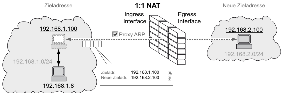
Abb. 43: Funktionsprinzip der Funktion 1:1-NAT
