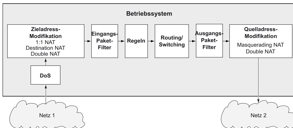
Abb. 42: Bearbeitungsreihenfolge der Datenpakete im Gerät
