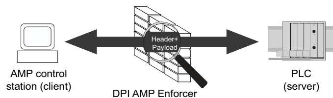
Abb. 24: Inspektion der Datenpakete
