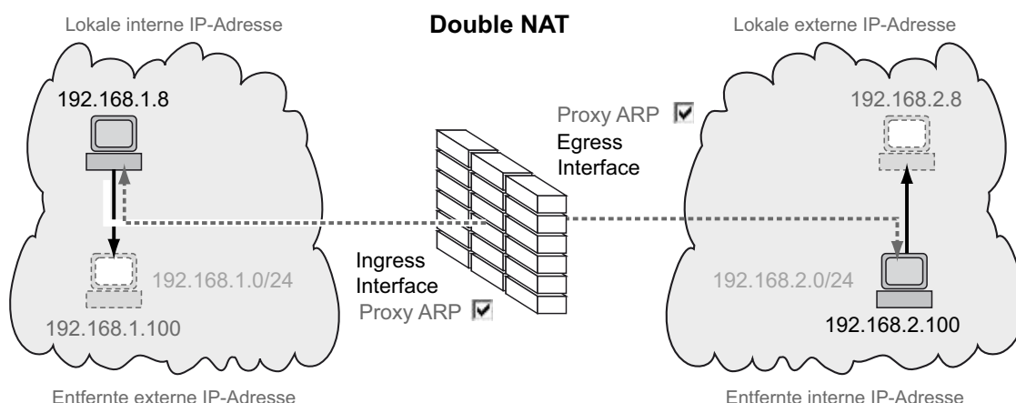
Abb. 47: Funktionsprinzip der Funktion Double-NAT
