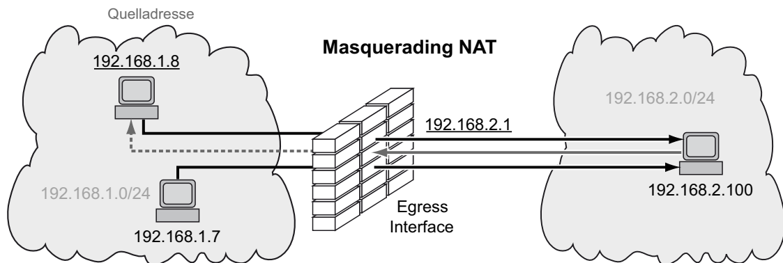
Abb. 46: Funktionsprinzip der Funktion Masquerading-NAT
