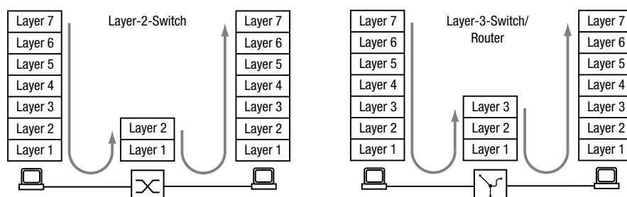
Abb. 31: Datentransport durch einen Switch und einen Router in den Schichten des OSI-Referenzmodells
