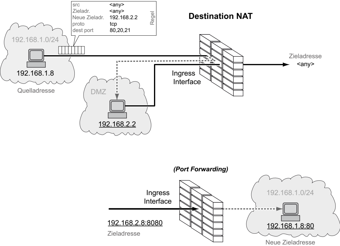
Abb. 45: Funktionsprinzip der Funktion Destination-NAT
