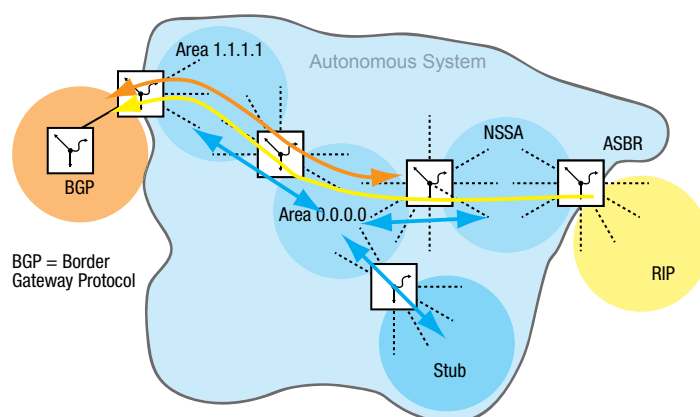
Abb. 54: LSA-Verteilung in die Area-Typen
