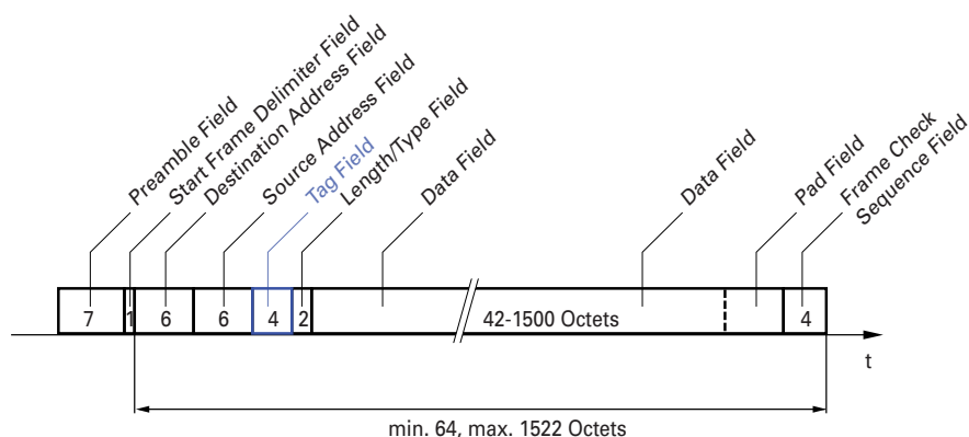
Abb. 26: Ethernet-Datenpaket mit Tag
