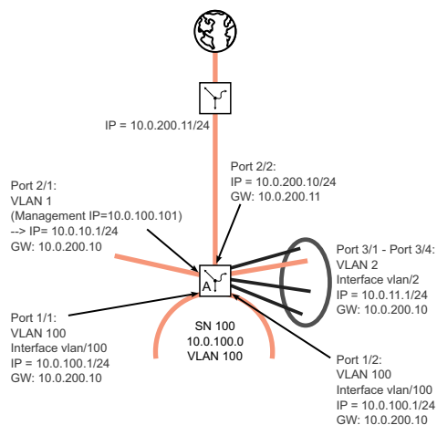
Abb. 61: IP-Parameter für Schicht-3-Gerät A
