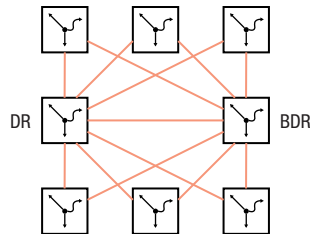
Abb. 57: LSA-Verteilung mit Designated-Router und Backup-Designated-Router
