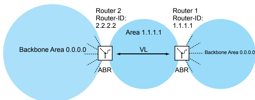
Abb. 56: Erweiterung der Backbone-Area durch eine virtuelle Verbindung (VL)
