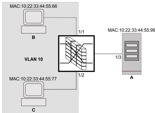
Abb. 19: Anwendungsbeispiel für Paketfilter auf Grundlage von MAC-Adressen
