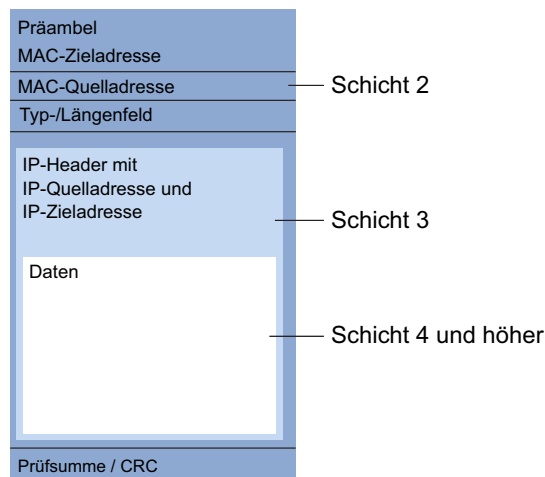
Abb. 34: Aufbau eines Datenpaketes aus Sicht des ISO/OSI-Referenzmodells
