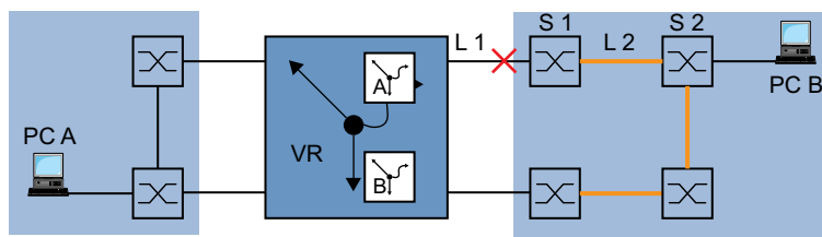
Abb. 62: Überwachen einer Leitung mit Interface-Tracking
