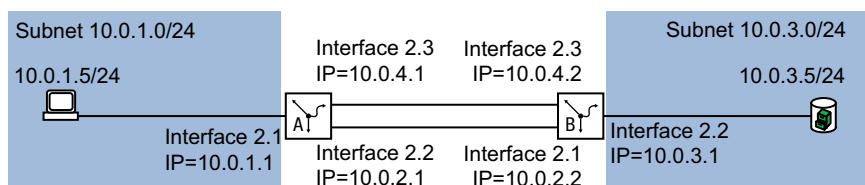
Abb. 41: Redundante statische Route
