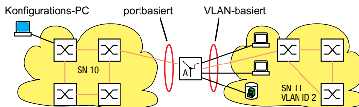
Abb. 37: Statische Routen: Beispiel für eine Verbindung zwischen zwei Fertigungszellen.
