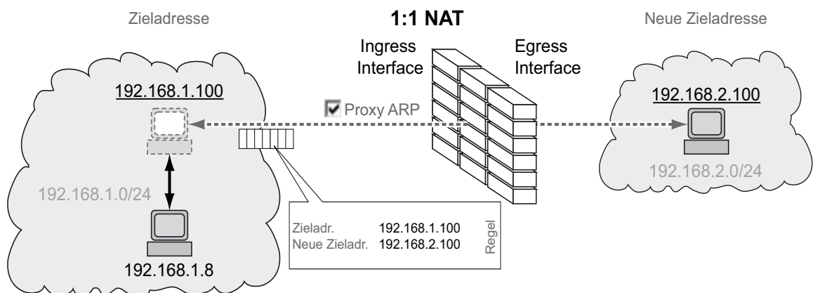
Abb. 3: Funktionsprinzip der Funktion 1:1-NAT
