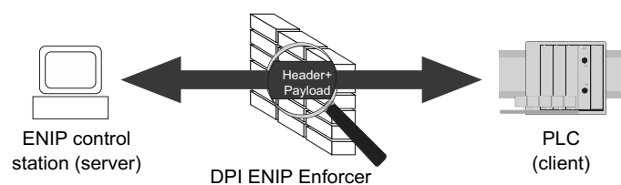
Abb. 25: Inspektion der Datenpakete
