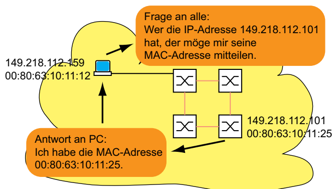
Abb. 33: ARP-Anfrage und -Antwort
