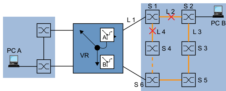
Abb. 64: Überwachen der Erreichbarkeit eines Geräts in einem redundanten Ring
