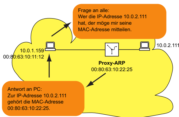
Abb. 35: Funktion Proxy-ARP
