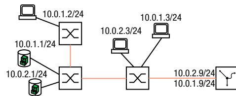
Abb. 36: Beispiel für Multinetting
