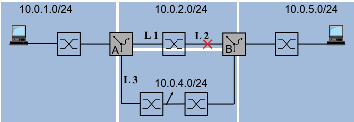
Abb. 65: Beispiel für statisches Route-Tracking
