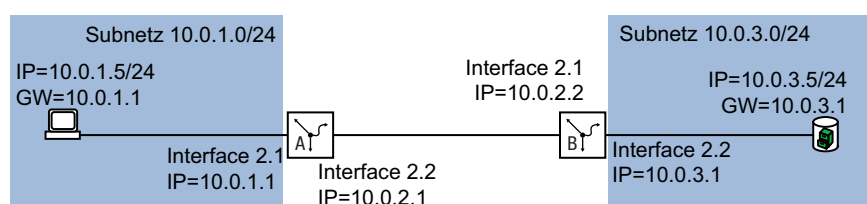
Abb. 58: Anwendungsbeispiel für ein OSPF-Setup
