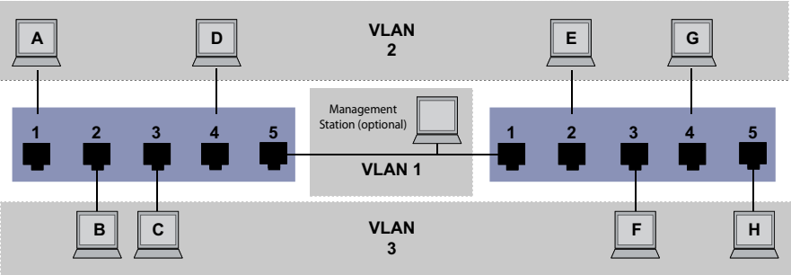
Abb. 30: Beispiel für eine komplexere VLAN-Konfiguration
