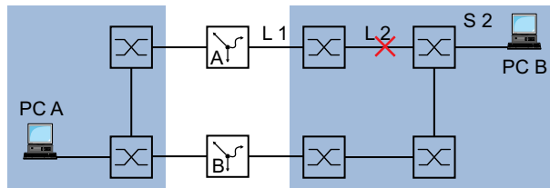
Abb. 63: Überwachen einer Leitung mit Ping-Tracking
