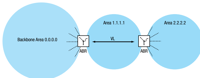
Abb. 55: Anbinden einer entfernten Area an die Backbone Area durch eine virtuelle Verbindung (VL)
