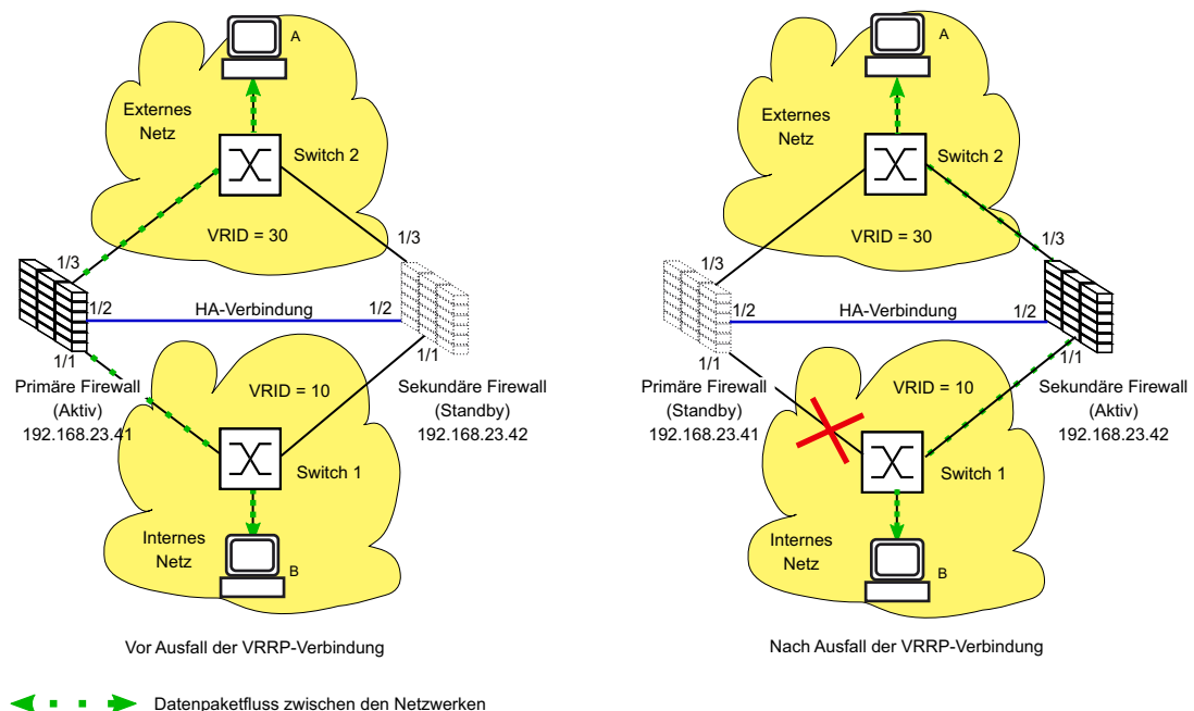
Abb. 52: Lauf der Datenpakete vor und nach dem Ausfall der internen VRRP-Verbindung
