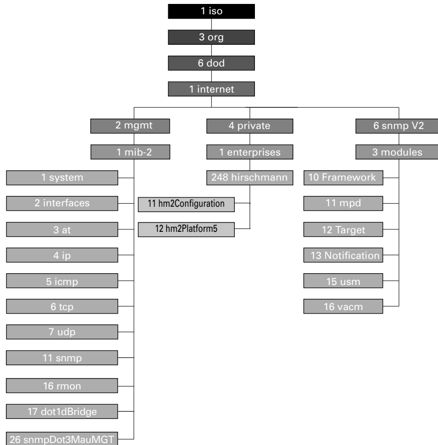
Abb. 67: Baumstruktur der Hirschmann-MIB
