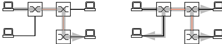
Abb. 32: MAC-Datenvermittlung: Unicast-Datenpaket (links) und Broadcast-Datenpaket (rechts)
