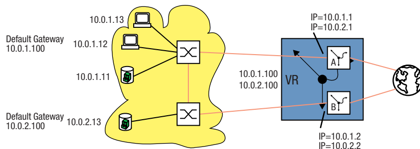
Abb. 51: Virtueller Router mit Multinetting
