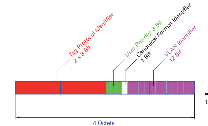
Abb. 27: Aufbau des VLAN-Tag
