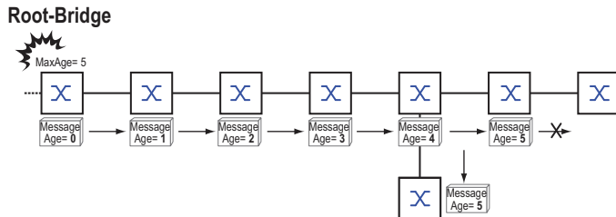
Abb. 37: Übertragung einer STP-BPDU in Abhängigkeit von MaxAge
