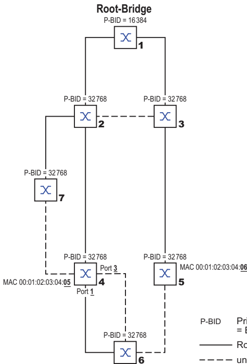
Abb. 39: Beispiel für die Bestimmung des Root-Pfads
