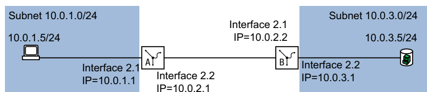
Abb. 42: Statisches Routing
