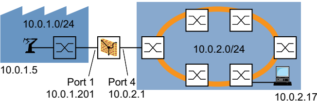
Abb. 18: Anwendungsbeispiel für ein Paketfilter-Setup
