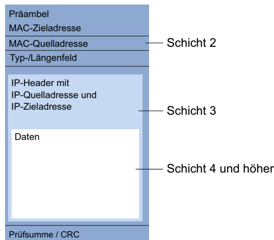
Abb. 36: Aufbau eines Datenpaketes aus Sicht des ISO/OSI-Referenzmodells
