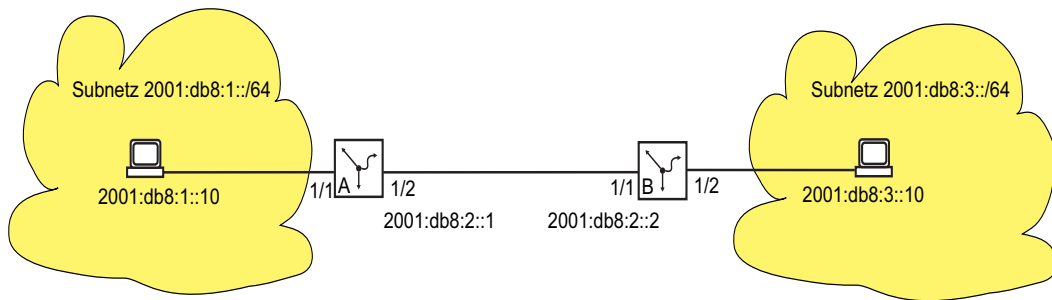
Abb. 45: Statisches Routing
