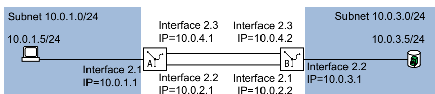
Abb. 43: Redundante statische Route
