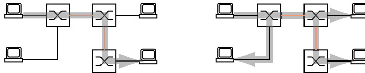
Abb. 34: MAC-Datenvermittlung: Unicast-Datenpaket (links) und Broadcast-Datenpaket (rechts)
