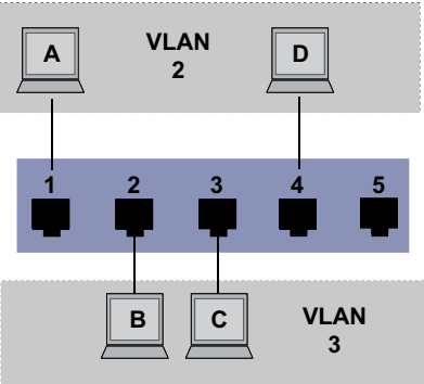
Abb. 31: Beispiel für ein einfaches Port-basiertes VLAN
