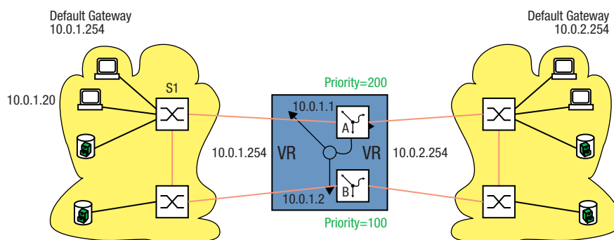
Abb. 55: Virtueller Router mit Lastverteilung
