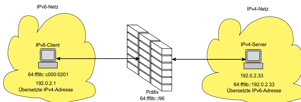
Abb. 52: Funktionsprinzip der Funktion NAT64
