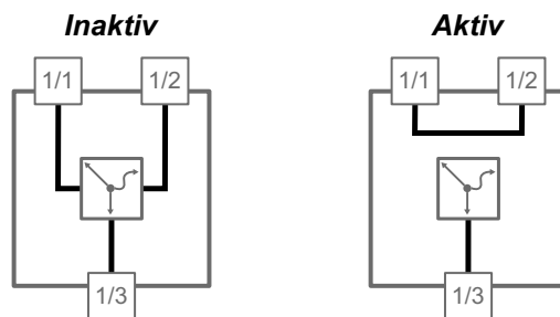
Abb. 16: Zustände des Hardware-LAN-Bypasses
