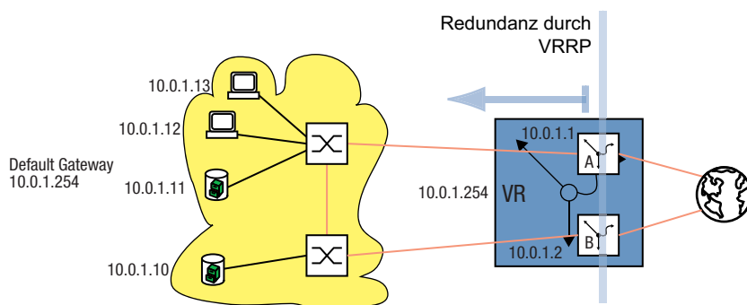
Abb. 53: Darstellung des virtuellen Routers
