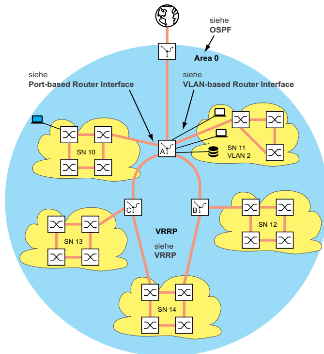
Abb. 64: Netzplan
