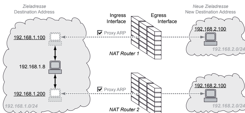
Abb. 48: Identische Produktionszellen mit Leitreechner verbinden (Anwendungsbeispiel)
