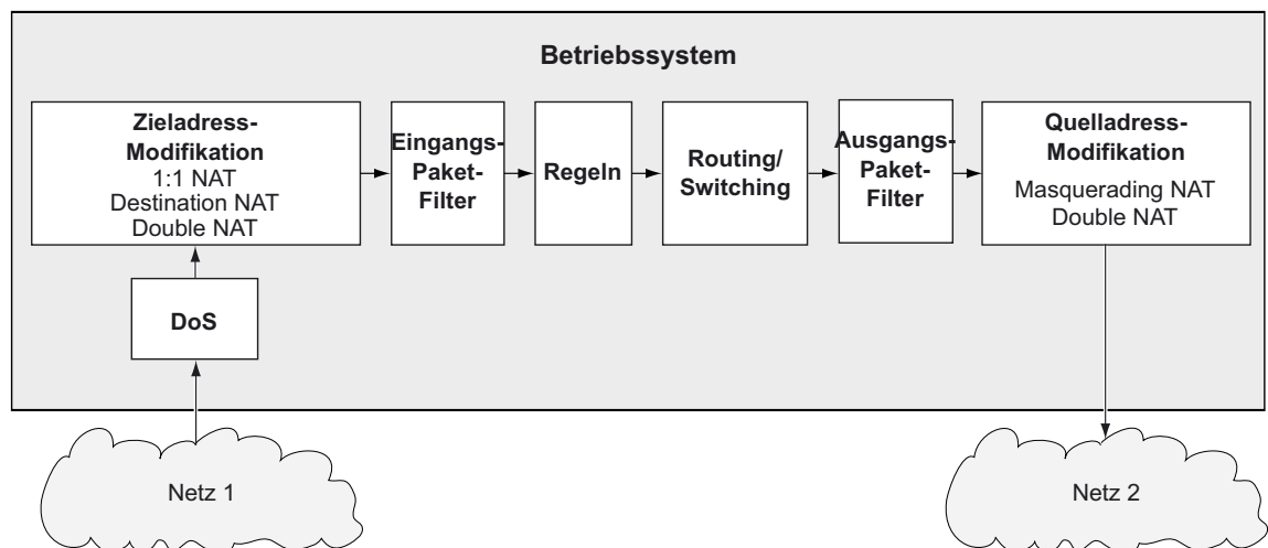
Abb. 17: Bearbeitungsreihenfolge der Datenpakete im Gerät
