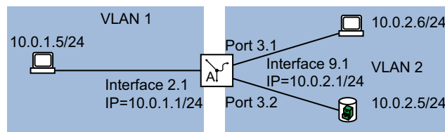
Abb. 41: VLAN-basiertes Router-Interface
