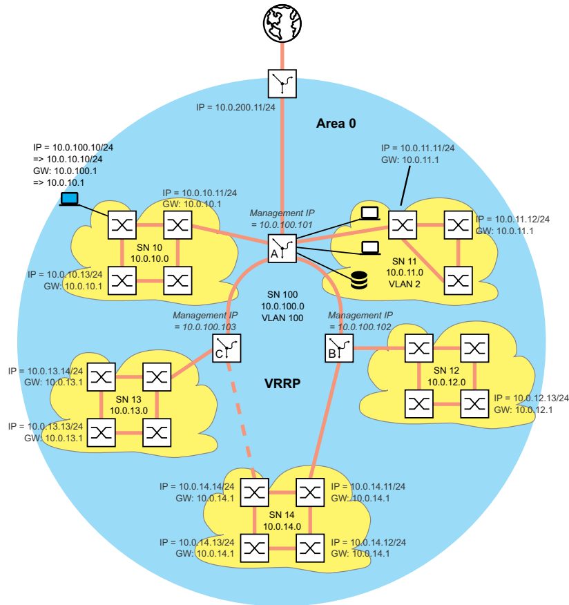
Abb. 65: Netzplan mit Management-IP-Adressen
