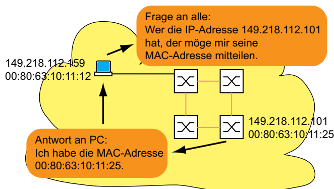
Abb. 35: ARP-Anfrage und -Antwort
