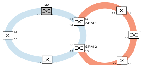
Abb. 48: Beispiel für eine Sub-Ring-Struktur blauer Ring = Hauptring oranger Ring = Sub-Ring SRM = Sub-Ring-Manager RM = Ring-Manager
