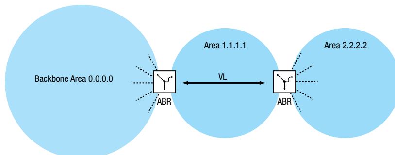
Abb. 95: Anbinden einer entfernten Area an die Backbone Area durch eine virtuelle Verbindung (VL)
