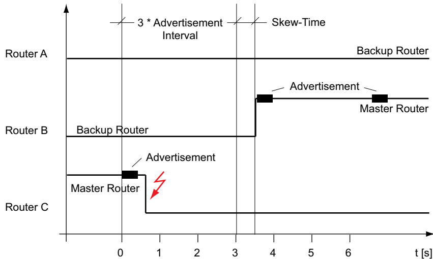
Abb. 85: Umschaltzeiten Master-Router <-> Backup-Router nach RFC 2338 VRRP-Priorität Router A = 64 VRRP-Priorität Router B = 128 VRRP-Priorität Router C = 254
