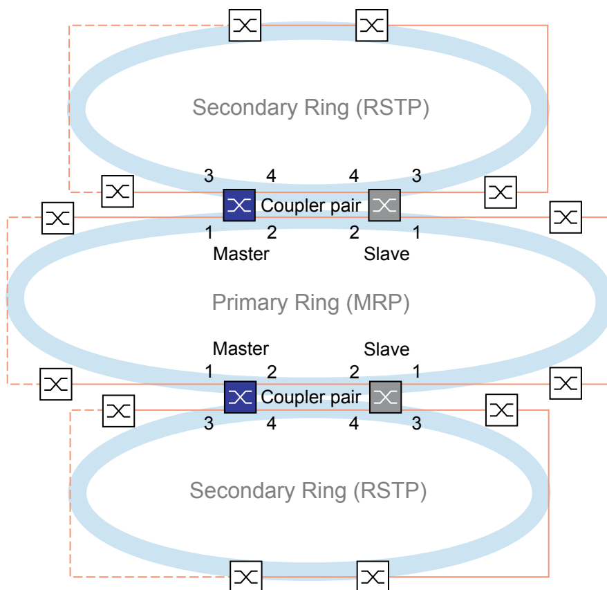
Abb. 70: Beispiel für eine redundante Zwei-Switch-Kopplung (2 Kopplerpaare) 1: Äußerer Kopplungs-Port im Primär-Ring 2: Innerer Kopplungs-Port im Primär-Ring 3: Äußerer Kopplungs-Port im Sekundär-Ring 4: Innerer Kopplungs-Port im Sekundär-Ring
