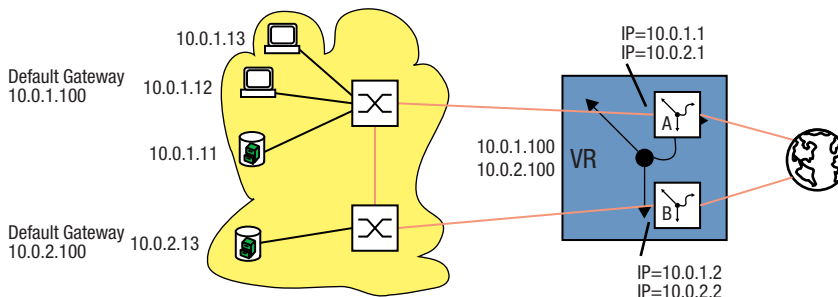
Abb. 89: Virtueller Router mit Multinetting
