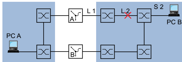
Abb. 106: Überwachen einer Leitung mit Ping-Tracking
