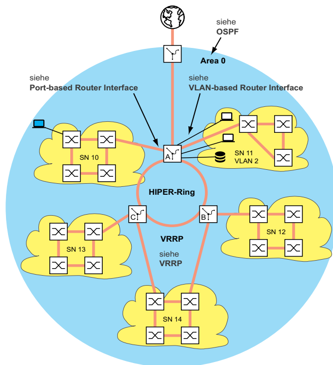
Abb. 102: Netzplan
