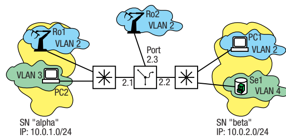
Abb. 99: Anwendungsbeispiel für ein Protokoll-basiertes VLAN
