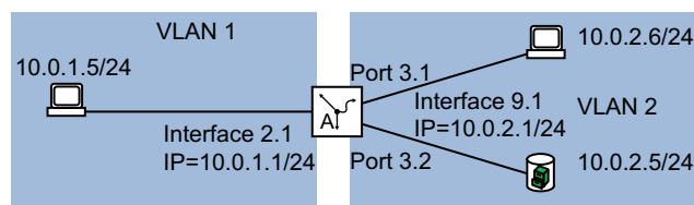
Abb. 80: VLAN-basiertes Router-Interface
