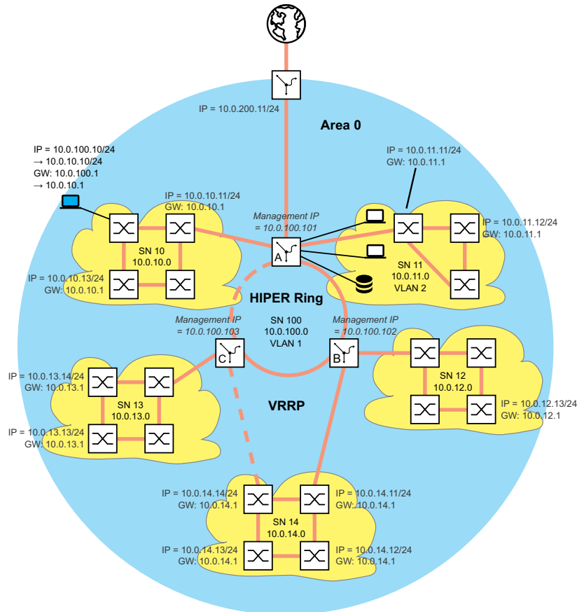
Abb. 103: Netzplan mit Management-IP-Adressen
