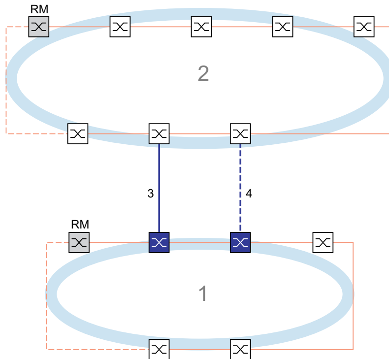
Abb. 56: Beispiel für die 2-Switch-Kopplung 1: Ring 2: Backbone 3: Hauptleitung 4: Redundante Leitung
