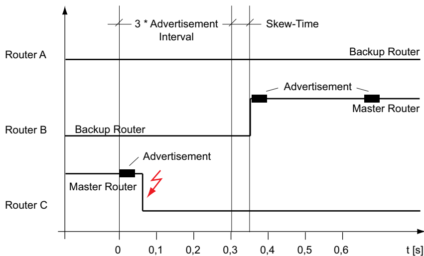
Abb. 86: Umschaltzeiten Master-Router <-> Backup-Router nach HiVRRP
