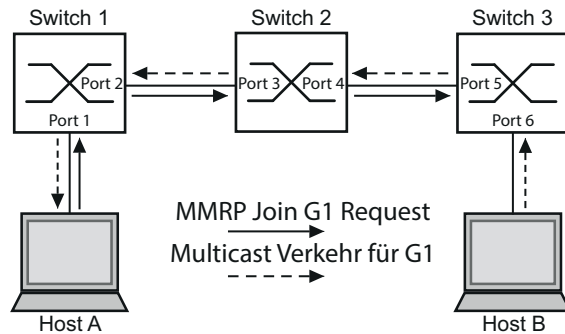
Abb. 124: MMRP -Netz für MAC-Adressen-Registrierung
