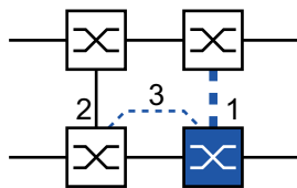
Abb. 61: 2-Switch-Kopplung mit Steuerleitung, Standby-Gerät
