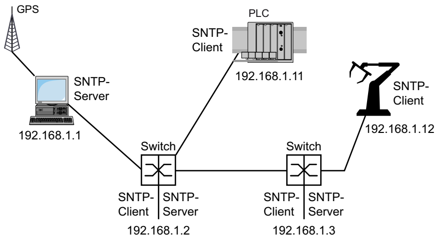
Abb. 16: Beispiel für SNTP-Kaskade
