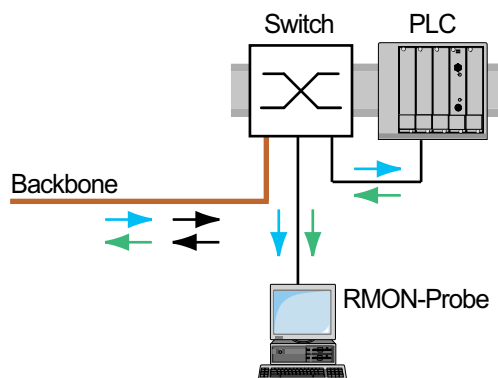
Abb. 111: Anwendungsbeispiel für ein Port-Mirroring-Setup
