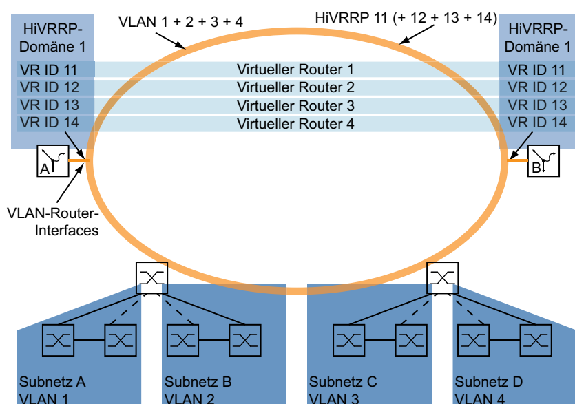
Abb. 87: Beispiel für die Anwendung einer HiVRRP-Domäne
