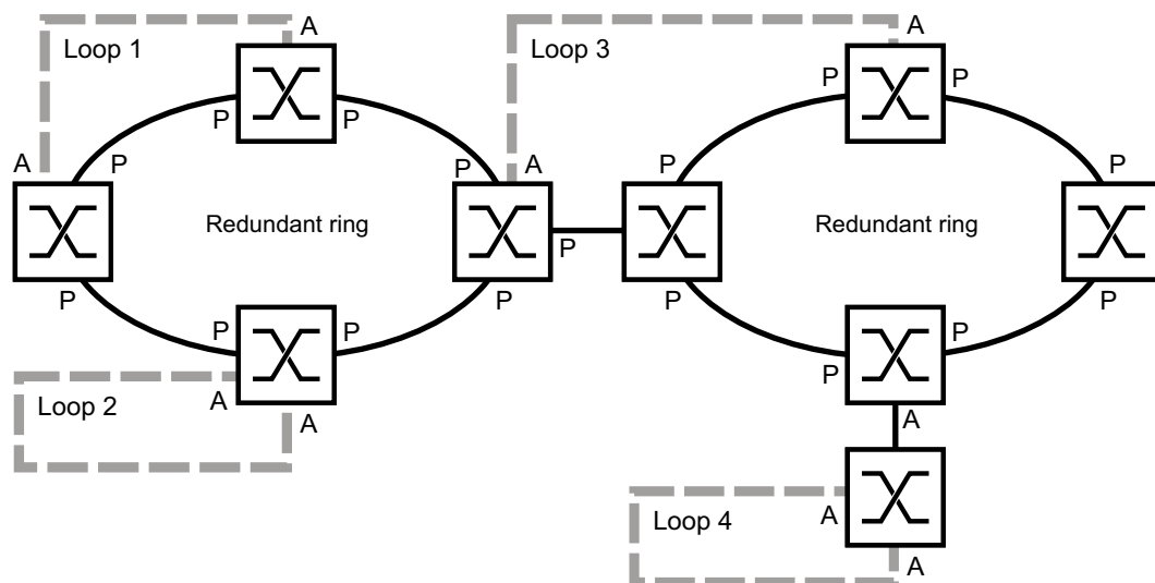
Abb. 110: Beispiele für unbeabsichtigte Schicht-2-Loops
