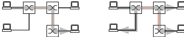
Abb. 73: MAC-Datenvermittlung: Unicast-Datenpaket (links) und Broadcast-Datenpaket (rechts)
