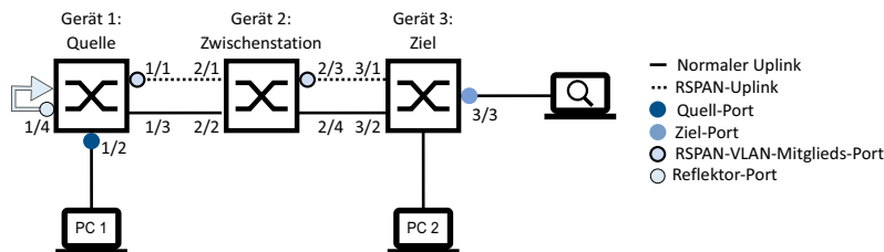
Abb. 118: RSPAN in einer Linien-Topologie, mittels Reflektor-Port (mit separaten Uplinks)
