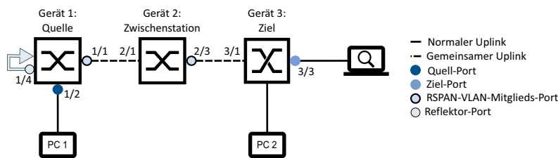
Abb. 119: RSPAN in einer Linien-Topologie, mittels Reflektor-Port (mit gemeinsamen Uplinks)
