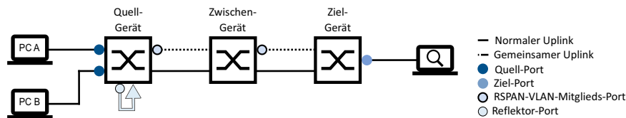
Abb. 113: Beispiel für eine Linien-Topologie mit einem Reflektor-Port (mit separaten Uplinks)
