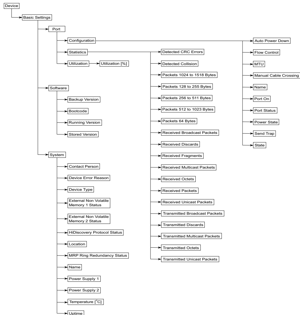
Abb. 127: OPC UA-Informationsmodell
