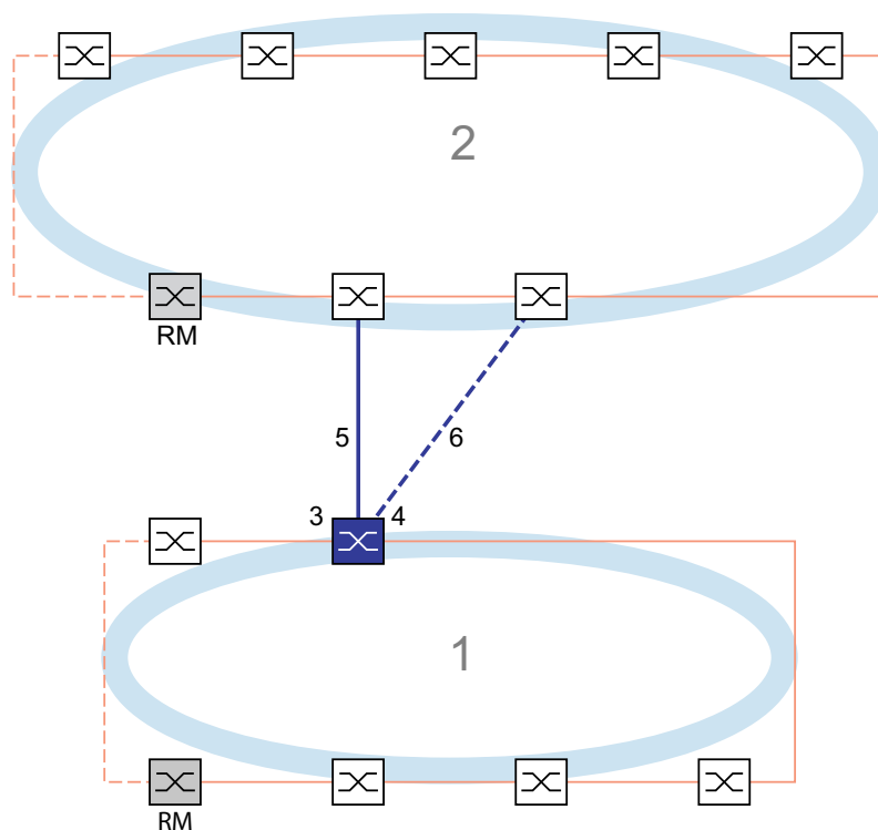
Abb. 55: Beispiel für die 1-Switch-Kopplung
