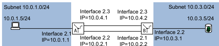
Abb. 82: Redundante statische Route
