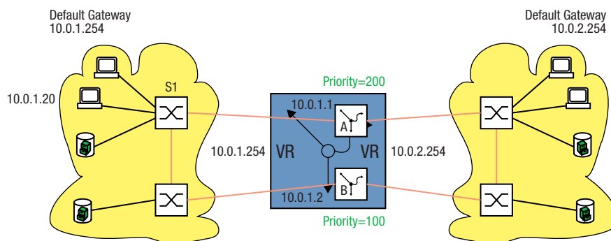
Abb. 88: Virtueller Router mit Lastverteilung
