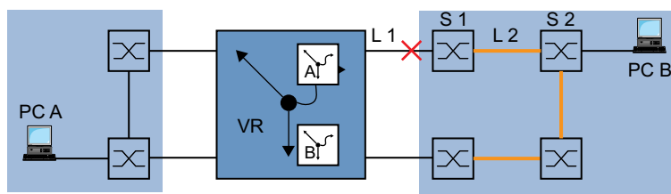
Abb. 105: Überwachen einer Leitung mit Interface-Tracking
