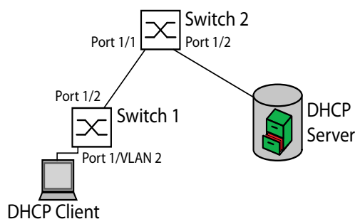
Abb. 123: Beispiel: DHCP-Schicht-2-Netz
