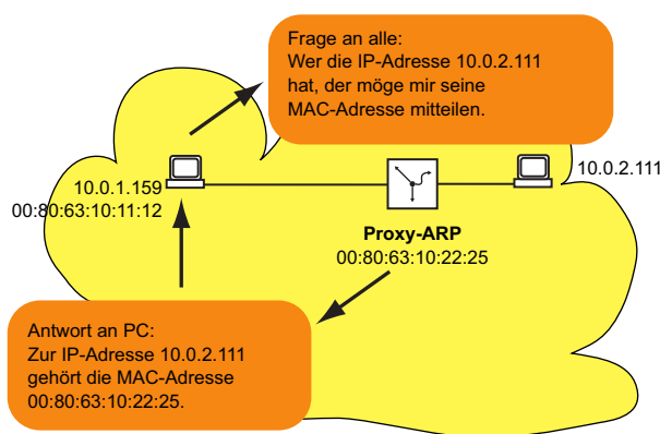
Abb. 76: Funktion Proxy-ARP
