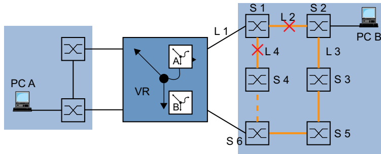
Abb. 107: Überwachen der Erreichbarkeit eines Geräts in einem redundanten Ring
