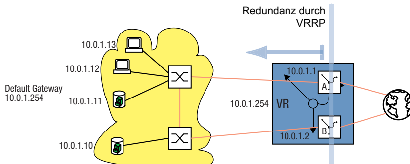
Abb. 83: Darstellung des virtuellen Routers
