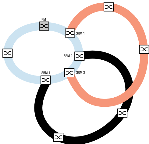
Abb. 48: Beispiel für eine überlappende Sub-Ring-Struktur
