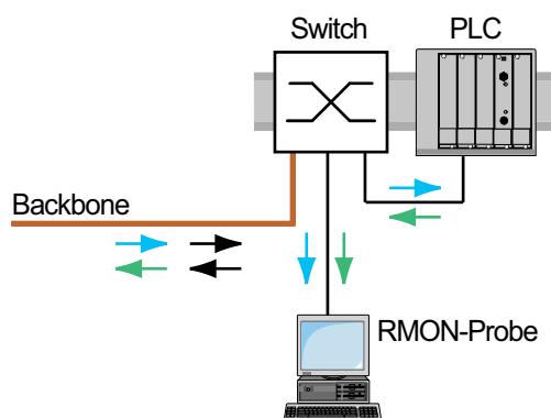
Abb. 73: Anwendungsbeispiel für ein Port-Mirroring-Setup
