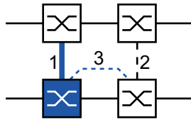
Abb. 59: 2-Switch-Kopplung mit Steuerleitung, primäres Gerät
