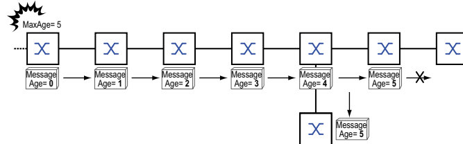
Abb. 39: Übertragung einer STP-BPDU abhängig von MaxAge
