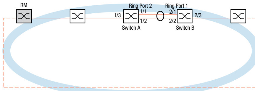
Abb. 34: Anwendungsbeispiel für ein MRP-über-LAG-Setup
