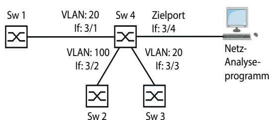
Abb. 74: Anwendungsbeispiel für ein VLAN-Mirroring -Setup
