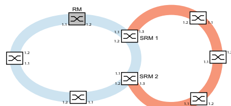
Abb. 47: Beispiel für eine Sub-Ring-Struktur blauer Ring = Hauptring oranger Ring = Sub-Ring SRM = Sub-Ring-Manager RM = Ring-Manager
