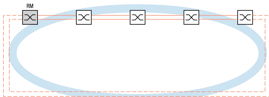
Abb. 32: Link-Aggregation für den gesamten MRP-Ring
