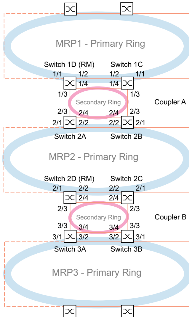
Abb. 70: Redundant Coupling Protocol-Zugtopologie: - Ports x/1 und x/2 sind MRP -Ring-Ports - Ports x/3 sind äußere RCP -Ports - Ports x/4 sind innere RCP -Ports
