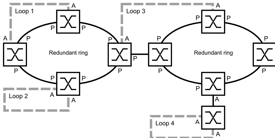
Abb. 72: Beispiele für unbeabsichtigte Schicht-2-Loops
