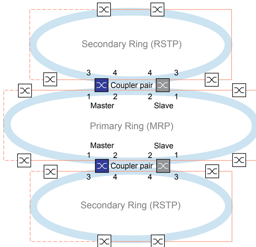
Abb. 69: Beispiel für eine redundante Zwei-Switch-Kopplung (2 Kopplerpaare)
