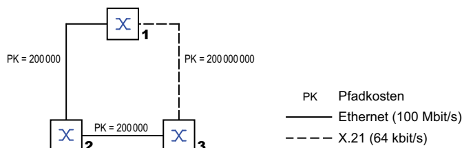
Abb. 36: Pfadkosten
