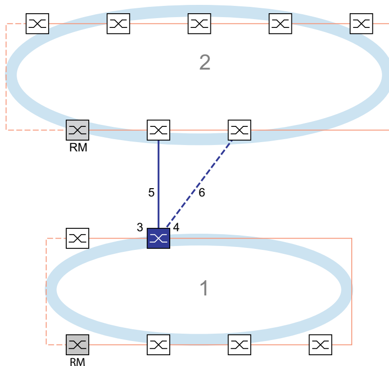
Abb. 54: Beispiel für die 1-Switch-Kopplung
