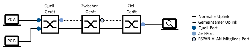
Abb. 76: Beispiel für eine Linien-Topologie, ohne Reflektor-Port (mit separaten Uplinks)
