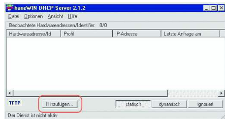
Abb. 62: Statische Adressen hinzufügen
