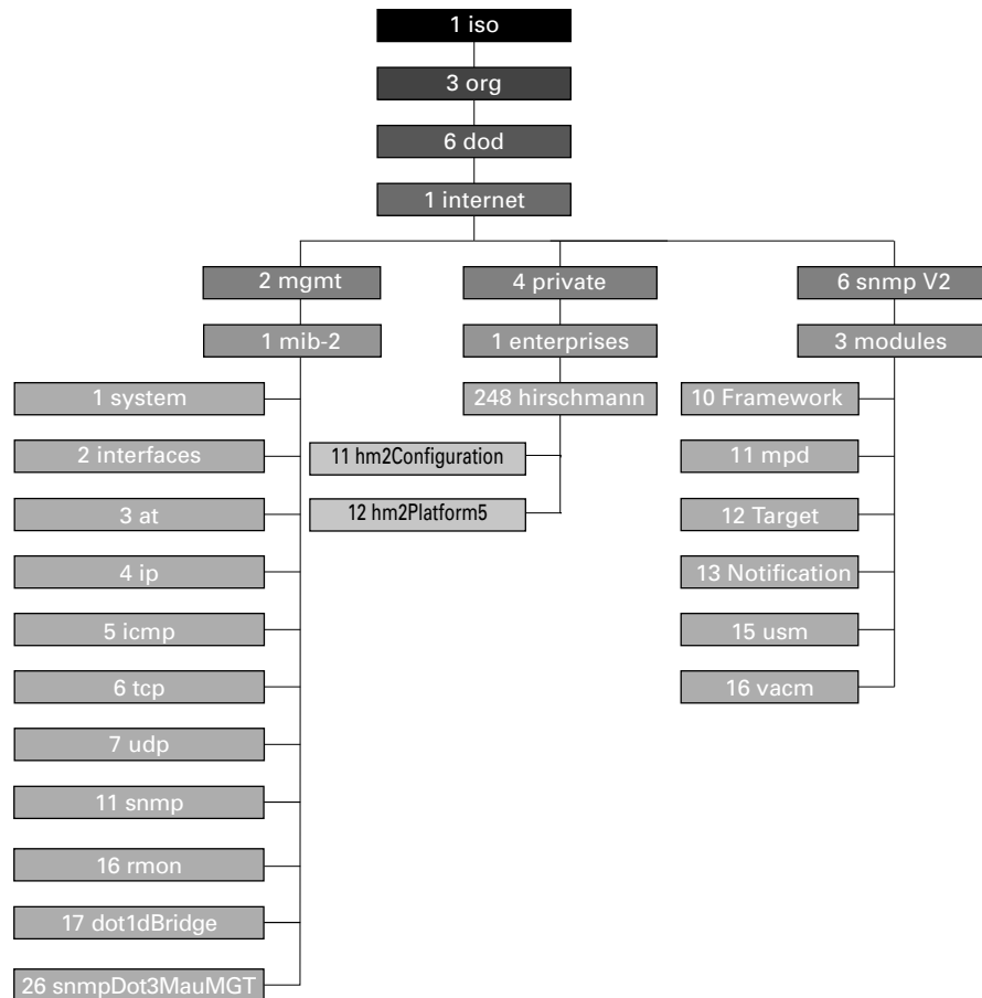
Abb. 71: Baumstruktur der Hirschmann-MIB
