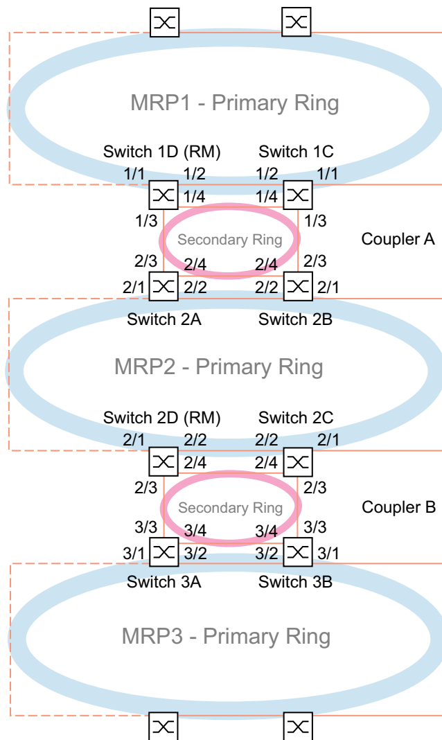
Abb. 73: Redundant Coupling Protocol-Zugtopologie: - Ports x/1 und x/2 sind MRP -Ring-Ports - Ports x/3 sind äußere RCP -Ports - Ports x/4 sind äußere RCP -Ports
