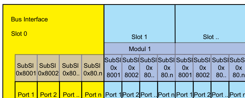
Abb. 96: Kombigerät
