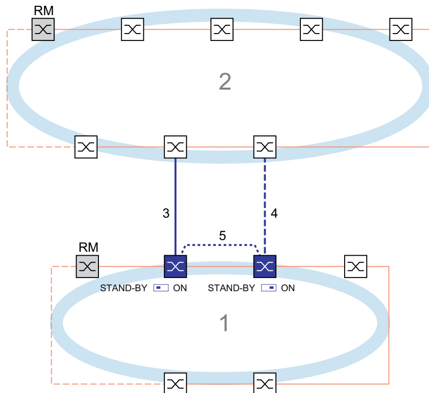
Abb. 69: Beispiel für die 2-Switch-Kopplung mit Steuerleitung 1: Ring 2: Backbone 3: Hauptleitung 4: Redundante Leitung 5: Steuerleitung
