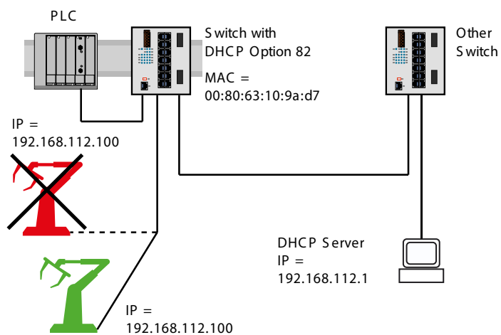
Abb. 112: Anwendungsbeispiel für den Einsatz von Option 82
