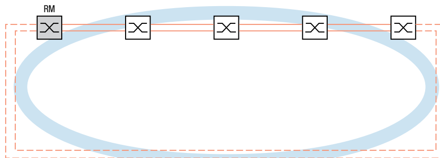
Abb. 35: Link-Aggregation für den gesamten MRP-Ring
