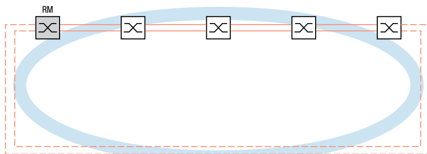
Abb. 34: Link-Aggregation für den gesamten MRP-Ring
