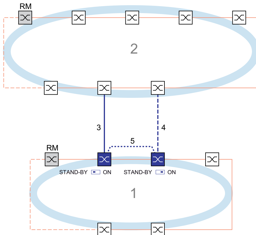
Abb. 68: Beispiel für die 2-Switch-Kopplung mit Steuerleitung 1: Ring 2: Backbone 3: Hauptleitung 4: Redundante Leitung 5: Steuerleitung
