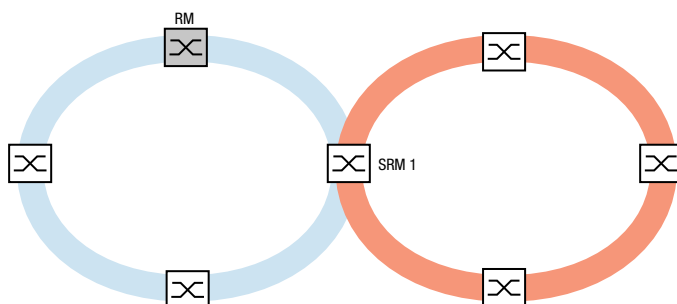
Abb. 52: Sonderfall: Ein Sub-Ring-Manager-Gerät verwaltet beide Enden eines Sub-Rings an unterschiedlichen Ports (Single-Sub-Ring-Manager).
