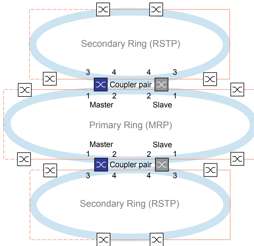
Abb. 71: Beispiel für eine redundante Zwei-Switch-Kopplung (2 Kopplerpaare)
