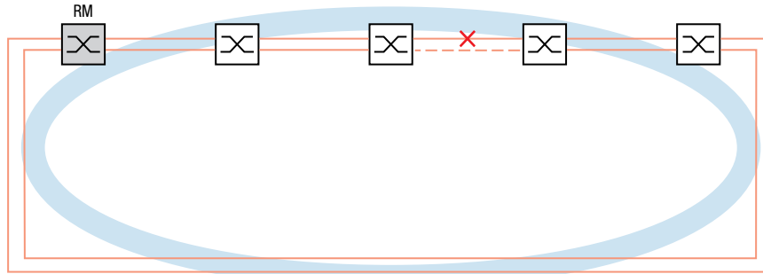
Abb. 35: Unterbrechung einer Verbindung in einem MRP-Ring
