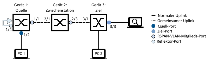
Abb. 83: RSPAN in einer Linien-Topologie, mittels Reflektor-Port (mit gemeinsamen Uplinks)
