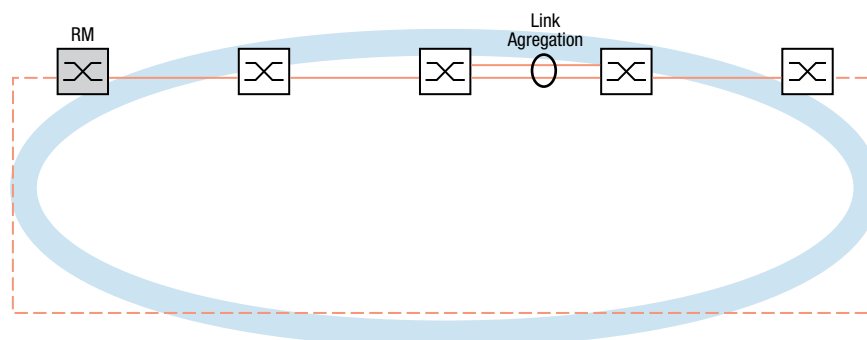
Abb. 33: Link-Aggregation über eine einzelne Verbindung eines MRP-Rings
