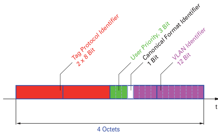
Abb. 18: Aufbau des VLAN-Tag
