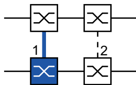
Abb. 66: 2-Switch-Kopplung, primäres Gerät 1: Kopplungs-Port 2: Partner-Kopplungs-Port
