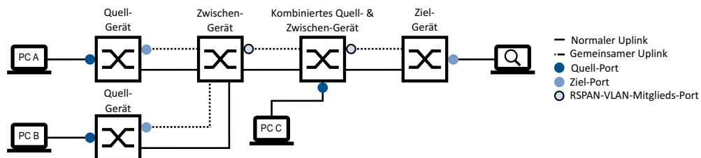
Abb. 80: Beispiel für eine komplexe Baum-Topologie, ohne Reflektor-Ports (mit separaten Uplinks)
