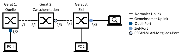
Abb. 85: RSPAN in einer Linien-Topologie, ohne einen Reflektor-Port (mit gemeinsamen Uplinks)
