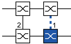
Abb. 59: 2-Switch-Kopplung, Standby-Gerät 1: Kopplungs-Port 2: Partner-Kopplungs-Port
