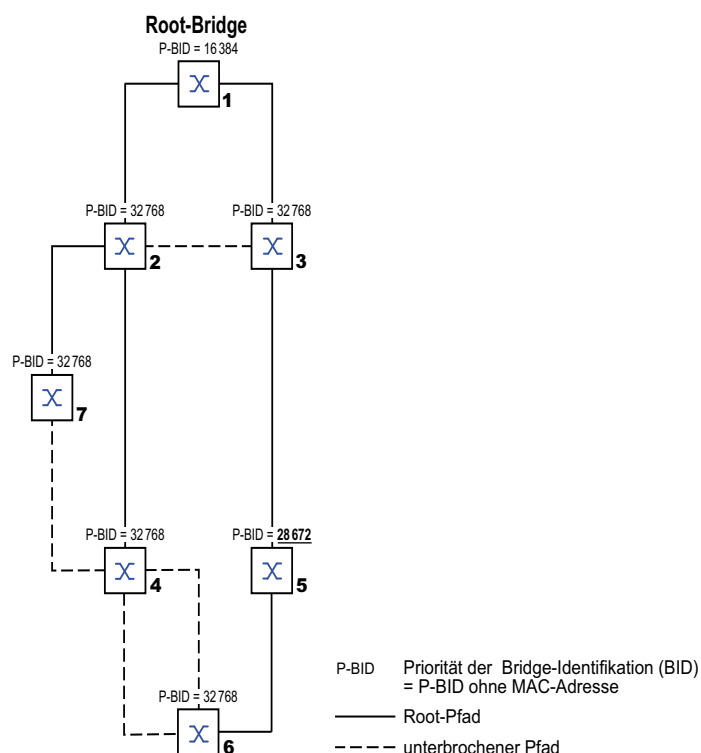
Abb. 44: Beispiel eines Netzplans für die Manipulation des Root-Pfads
