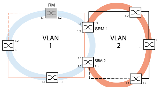
Abb. 53: Beispiel für eine Sub-Ring-Struktur mit VLANs orangefarbene Linie= Mitglieder des Hauptrings in VLAN 1 schwarze Linie= Mitglieder des Sub-Rings in VLAN 2 orange gestrichelte Linie= unterbrochenes Segment im Hauptring schwarz gestrichelte Linie= unterbrochenes Segment im Sub-Ring SRM = Sub-Ring-Manager RM = Ring-Manager
