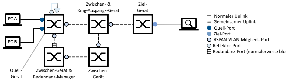
Abb. 81: Beispiel für eine einfache Ring-Topologie auf der Grundlage eines bestehenden redundanten Rings (mit gemeinsamen Links)
