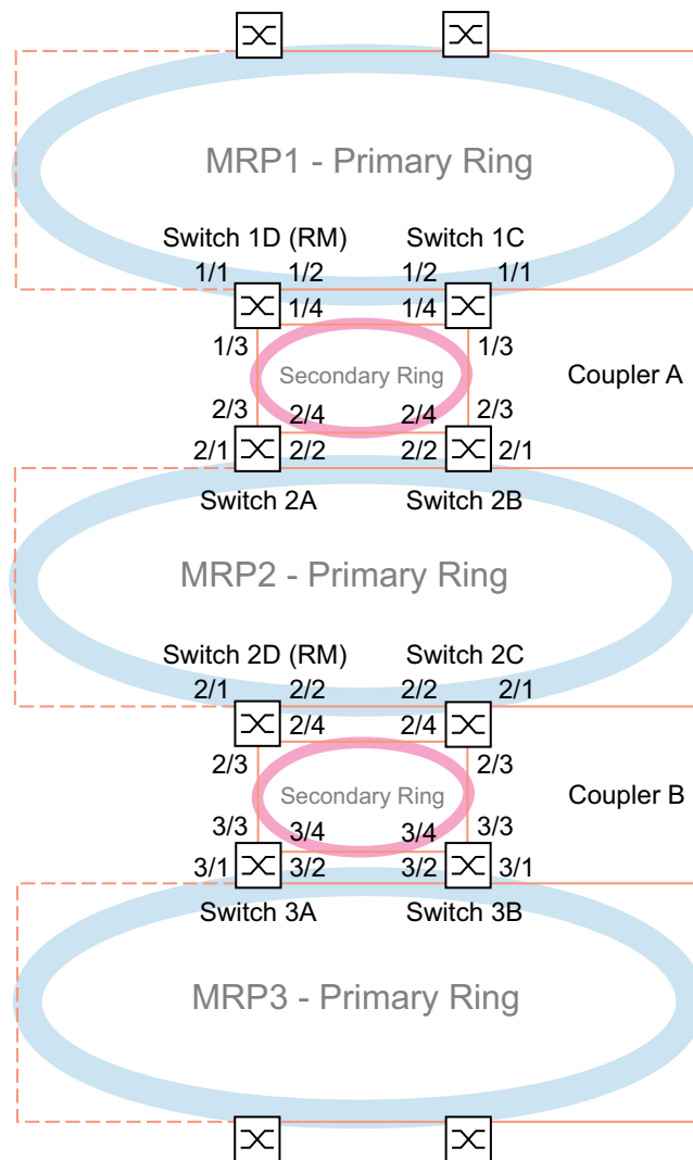
Abb. 72: Redundant Coupling Protocol-Zugtopologie: - Ports x/1 und x/2 sind MRP -Ring-Ports - Ports x/3 sind äußere RCP -Ports - Ports x/4 sind innere RCP -Ports
