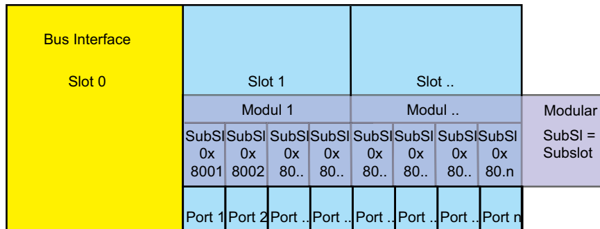
Abb. 68: Modulares Gerät
