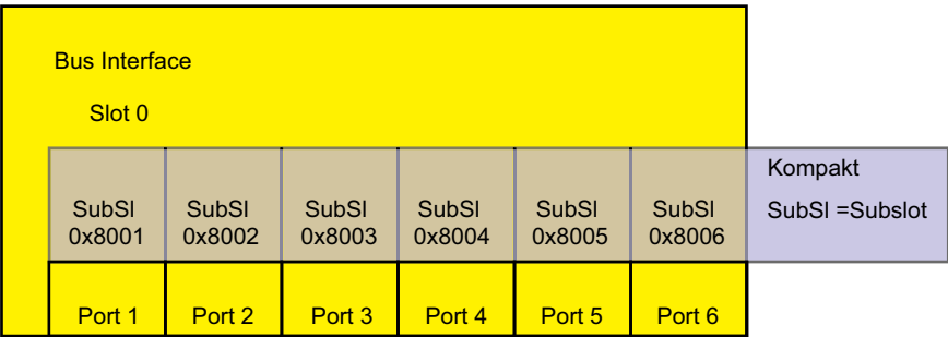
Abb. 67: Kompaktes Gerät
