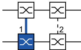
Abb. 51: 2-Switch-Kopplung, primäres Gerät 1: Kopplungs-Port 2: Partner-Kopplungs-Port
