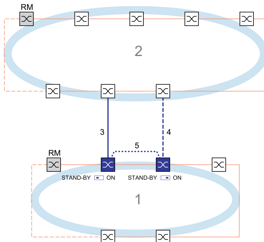
Abb. 45: Beispiel für die 2-Switch-Kopplung mit Steuerleitung 1: Ring 2: Backbone 3: Hauptleitung 4: Redundante Leitung 5: Steuerleitung
