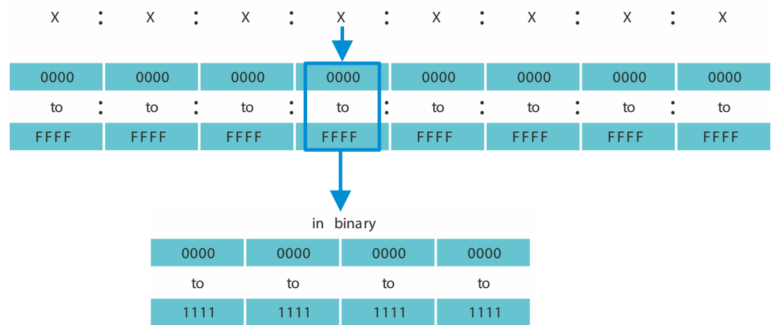
Abb. 8: Darstellung der IPv6-Adresse
