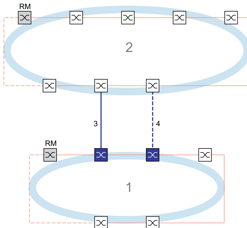
Abb. 42: Beispiel für die 2-Switch-Kopplung 1: Ring 2: Backbone 3: Hauptleitung 4: Redundante Leitung
