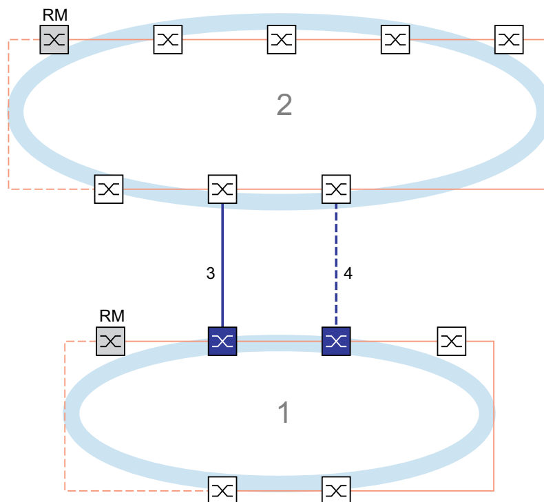
Abb. 50: Beispiel für die 2-Switch-Kopplung 1: Ring 2: Backbone 3: Hauptleitung 4: Redundante Leitung
