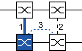
Abb. 46: 2-Switch-Kopplung mit Steuerleitung, primäres Gerät 1: Kopplungs-Port 2: Partner-Kopplungs-Port 3: Steuerleitung
