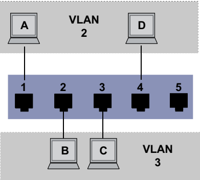
Abb. 21: Beispiel für ein einfaches Port-basiertes VLAN
