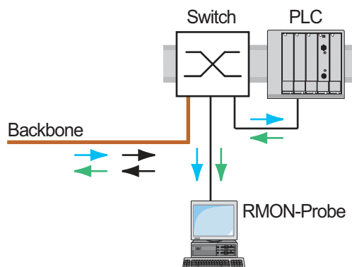
Abb. 60: Anwendungsbeispiel für ein Port-Mirroring-Setup
