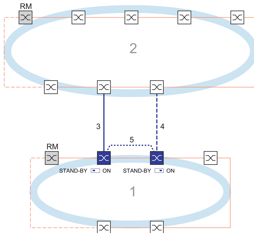
Abb. 57: Beispiel für die 2-Switch-Kopplung mit Steuerleitung 1: Ring 2: Backbone 3: Hauptleitung 4: Redundante Leitung 5: Steuerleitung
