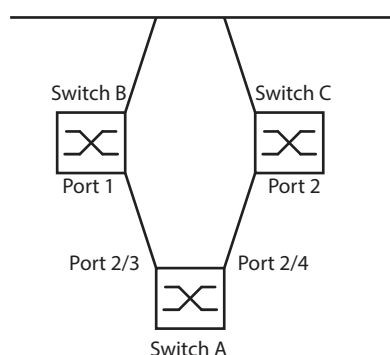
Abb. 44: Link-Backup Beispiel-Netzwerk
