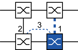
Abb. 51: 2-Switch-Kopplung mit Steuerleitung, Standby-Gerät 1: Kopplungs-Port 2: Partner-Kopplungs-Port 3: Steuerleitung
