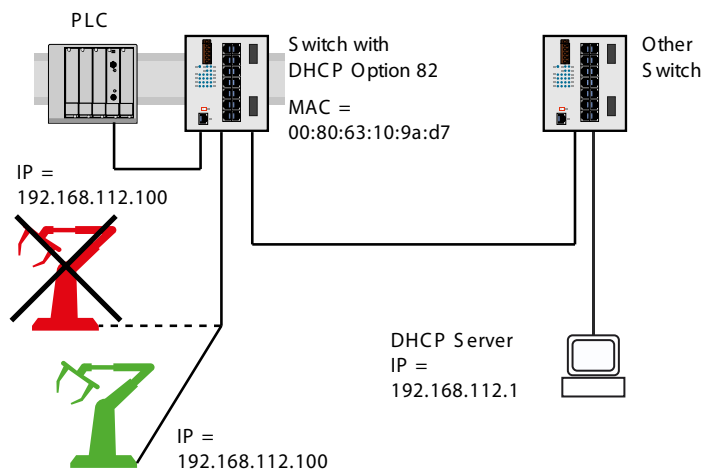
Abb. 88: Anwendungsbeispiel für den Einsatz von Option 82
