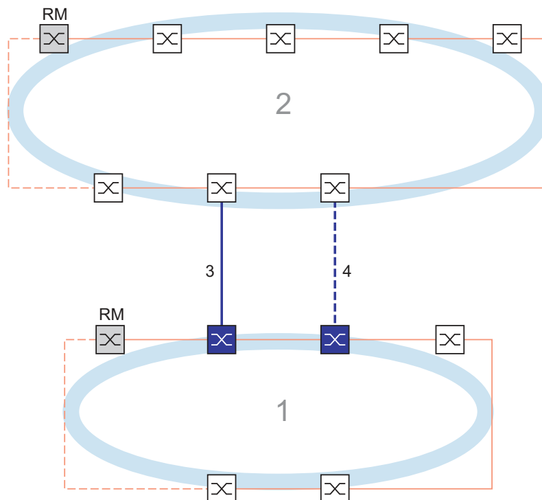
Abb. 54: Beispiel für die 2-Switch-Kopplung
