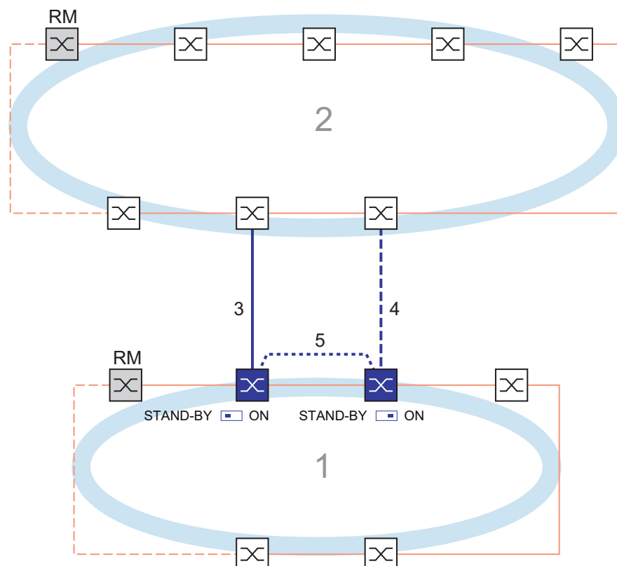
Abb. 49: Beispiel für die 2-Switch-Kopplung mit Steuerleitung 1: Ring 2: Backbone 3: Hauptleitung 4: Redundante Leitung 5: Steuerleitung
