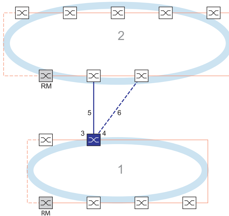
Abb. 45: Beispiel für die 1-Switch-Kopplung
