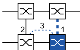
Abb. 59: 2-Switch-Kopplung mit Steuerleitung, Standby-Gerät
