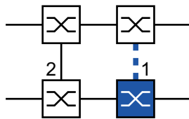
Abb. 56: 2-Switch-Kopplung, Standby-Gerät 1: Kopplungs-Port 2: Partner-Kopplungs-Port
