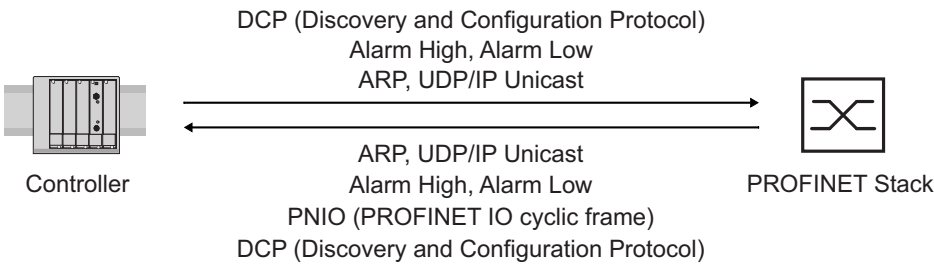
Abb. 69: Kommunikation zwischen Controller und dem Gerät
