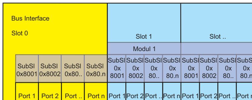
Abb. 72: Kombigerät
