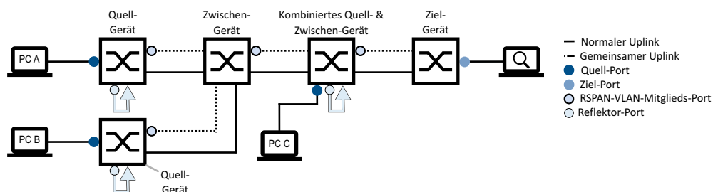
Abb. 78: Beispiel für eine komplexe Baum-Topologie mit Reflektor-Ports (mit separaten Uplinks)
