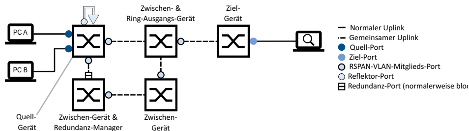
Abb. 79: Beispiel für eine einfache Ring-Topologie auf der Grundlage eines bestehenden redundanten Rings (mit gemeinsamen Links)
