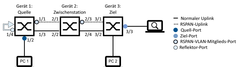
Abb. 80: RSPAN in einer Linien-Topologie, mittels Reflektor-Port (mit separaten Uplinks)
