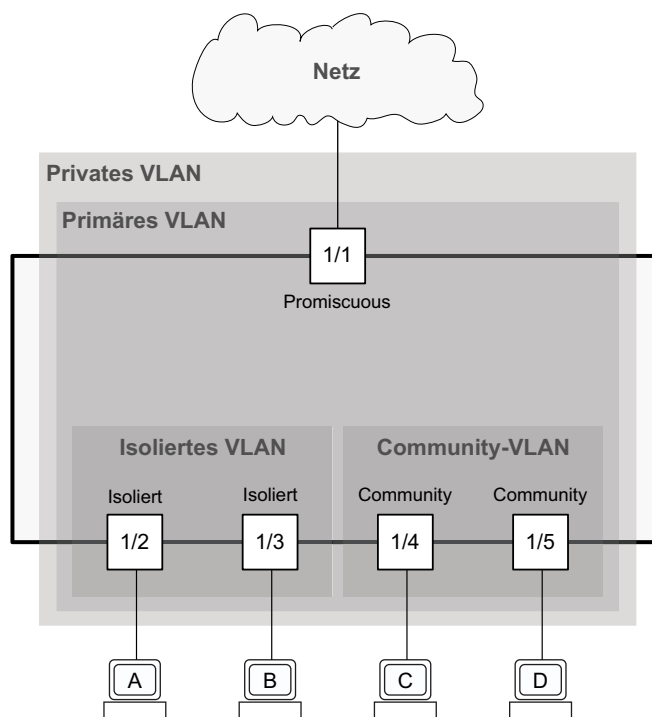
Abb. 24: Aufbau eines privaten VLANs
