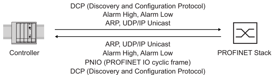
Abb. 93: Kommunikation zwischen Controller und dem Gerät
