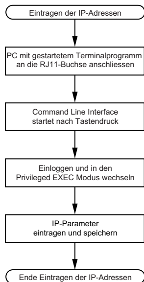
Abb. 10: Ablaufdiagramm Eintragen der IP-Adressen
