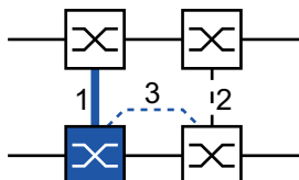
Abb. 70: 2-Switch-Kopplung mit Steuerleitung, primäres Gerät
