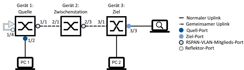
Abb. 81: RSPAN in einer Linien-Topologie, mittels Reflektor-Port (mit gemeinsamen Uplinks)
