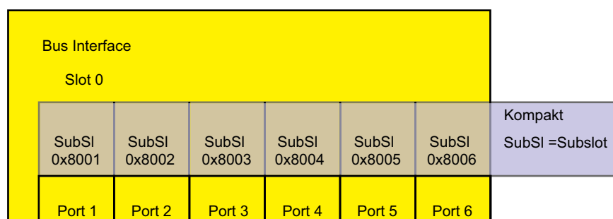
Abb. 94: Kompaktes Gerät
