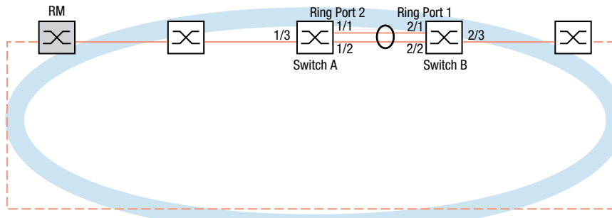
Abb. 37: Anwendungsbeispiel für ein MRP-über-LAG-Setup
