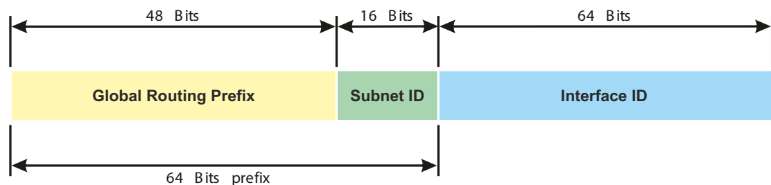
Abb. 9: Allgemeines Format der IPv6-Global-Unicast-Adresse
