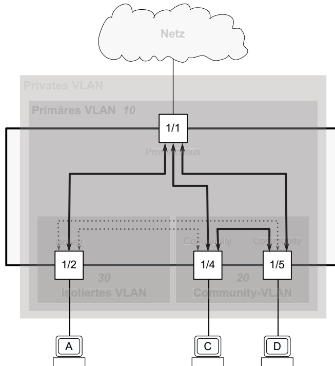
Abb. 27: Beispiel für ein privates VLAN
