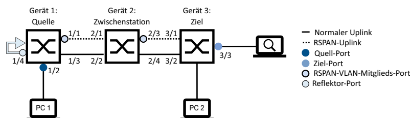
Abb. 80: RSPAN in einer Linien-Topologie, mittels eines Reflektor-Ports (mit separaten Uplinks)
