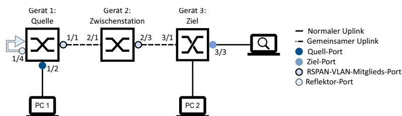
Abb. 81: RSPAN in einer Linien-Topologie, mittels eines Reflektor-Ports (mit gemeinsamen Uplinks)
