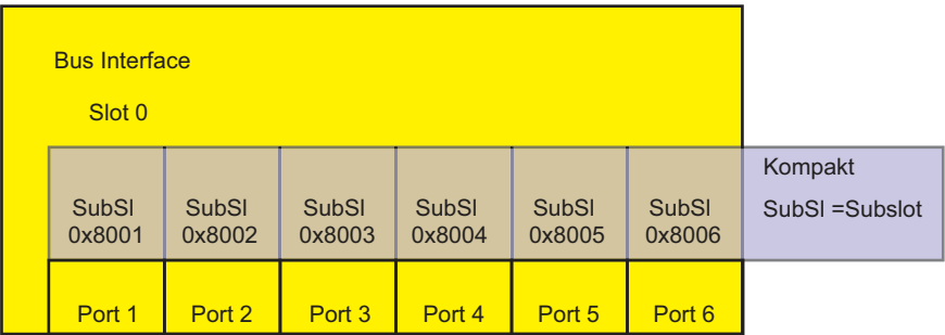
Abb. 91: Kompaktes Gerät
