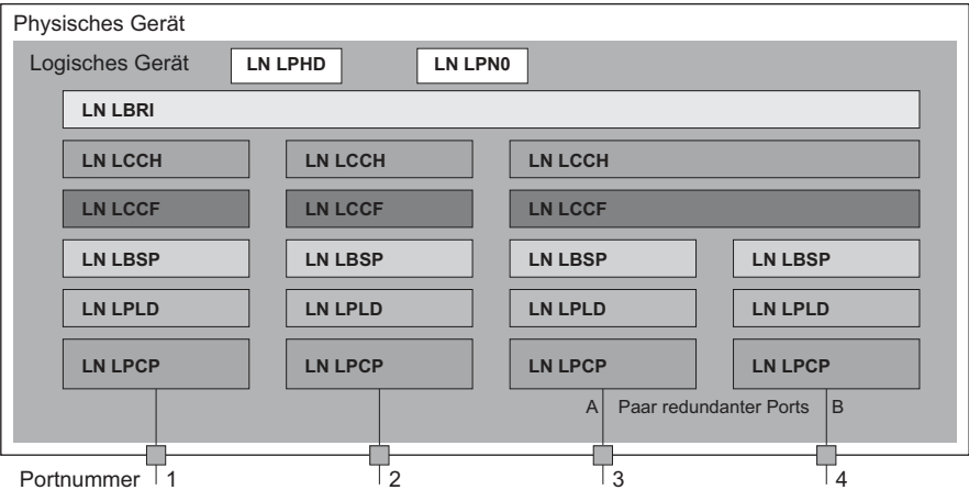
Abb. 86: Bridge-Modell nach Technical Report IEC 61850 90-4
