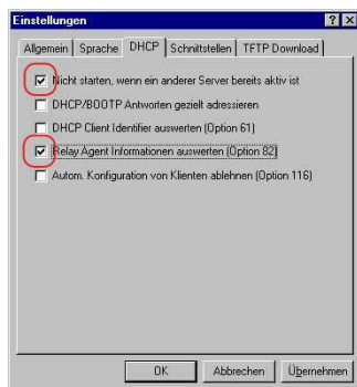
Abb. 107: DHCP-Einstellung
