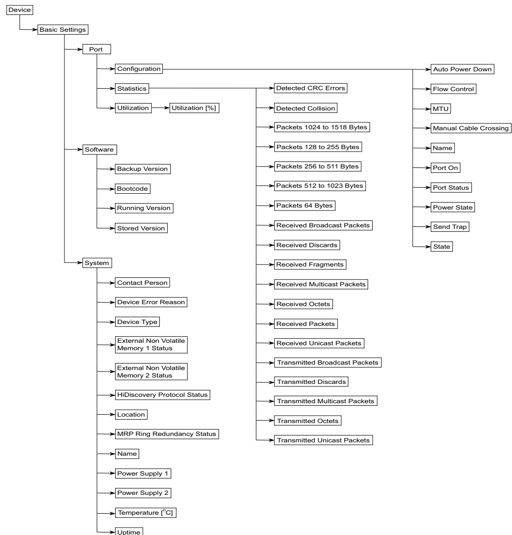
Abb. 97: OPC UA-Informationsmodell
