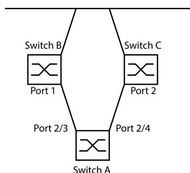
Abb. 50: Link-Backup Beispiel-Netzwerk
