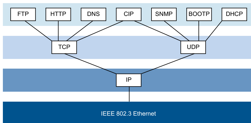
Abb. 96: IEEE 802.3 EtherNet/IP
