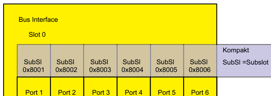
Abb. 100: Kompaktes Gerät
