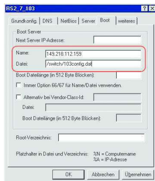
Abb. 107: Konfigurationsdatei auf dem tftp-Server
