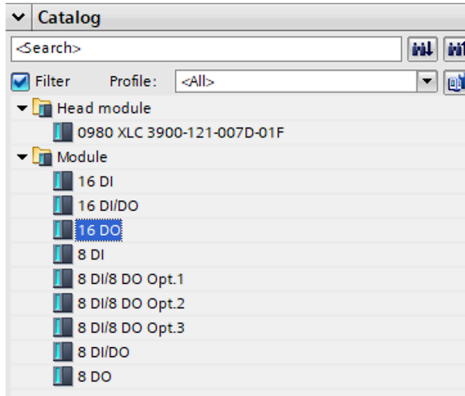
Abb. 20: I/O-Kanalkonfiguration
