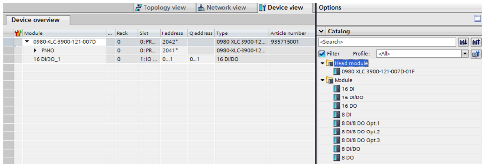
Abb. 17: Voreinstellung der Kanäle
