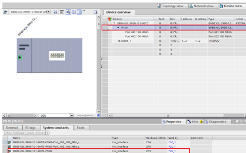
Abb. 26: TIA Portal® Hardware-Identifizierung des PROFINET-Interface für I&M 0-3 RDREC/WRREC
