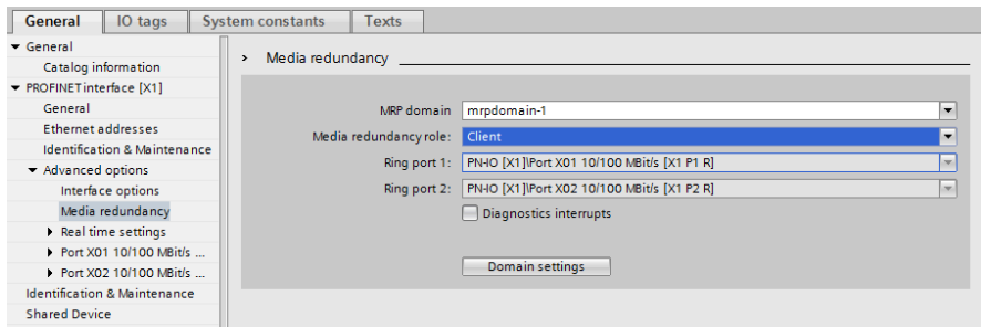
Abb. 24: Beispiel für die Einrichtung eines MRP-Clients im TIA Portal®
