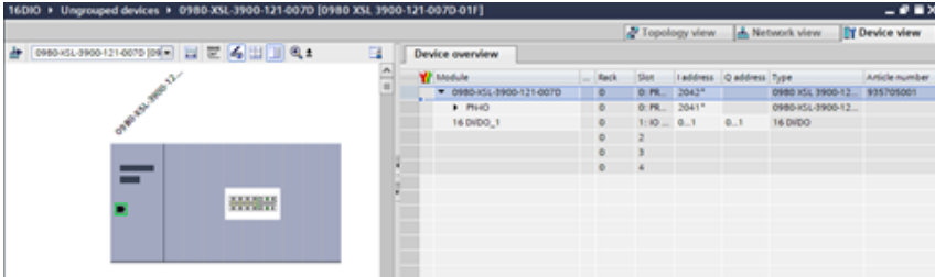
Abb. 12: Gerät konfigurieren
