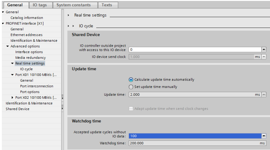
Abb. 25: Beispiel für die Einrichtung der Watchdog-Zeitüberwachung im TIA Portal® für die Nutzung von MRP
