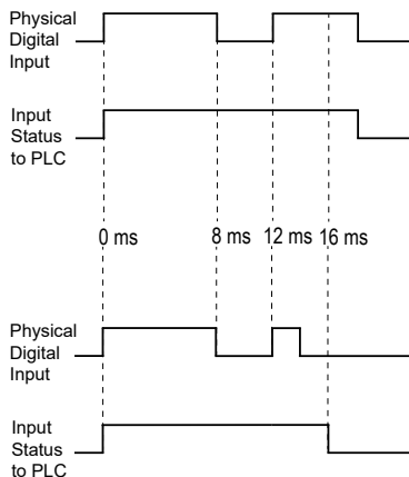
Figure 22: DI Extension
