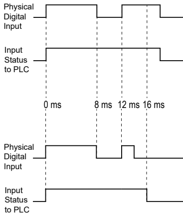
Abb. 9: DI Extension
