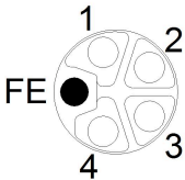
Abb. 7: Schemazeichnung M12 L-Kodierung (Buchse X04 für Power Out)
