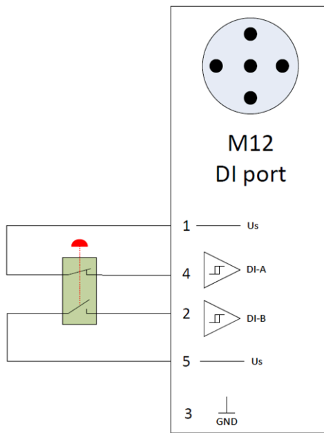
Abb. 63: Internes F-DI Blockdiagramm
