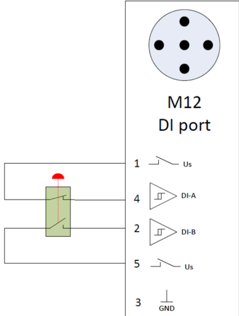
Abb. 68: Internes F-DI Blockdiagramm
