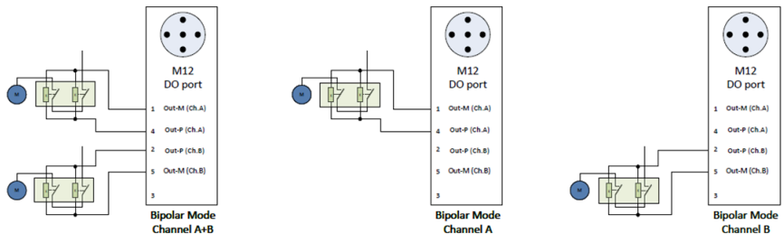
Abb. 7: Zulässige Anwendungsfälle für den bipolaren Modus
