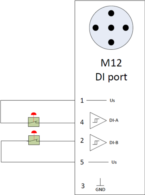
Abb. 62: Internes F-DI Blockdiagramm
