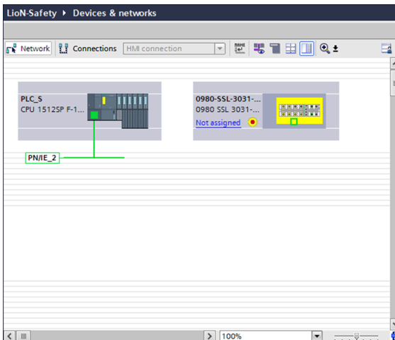
Abb. 10: Netzwerksicht
