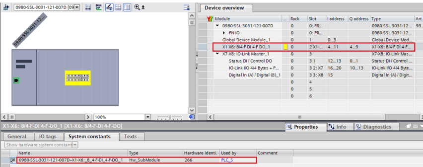
Abb. 50: Hardware-Identifizierung des Safety-Moduls für I&M 4 RDREC
