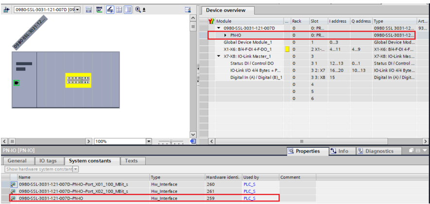
Abb. 49: TIA Portal® Hardware-Identifizierung des PROFINET-Interfaces für I&M 0-3 RDREC/WRREC
