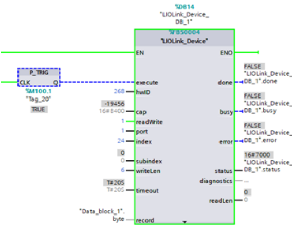
Abb. 33: "Write"-Beispiel FB50004
