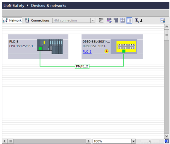
Abb. 11: Gerät zuweisen
