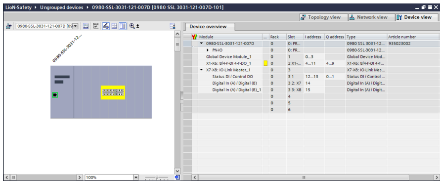
Abb. 12: Gerät konfigurieren
