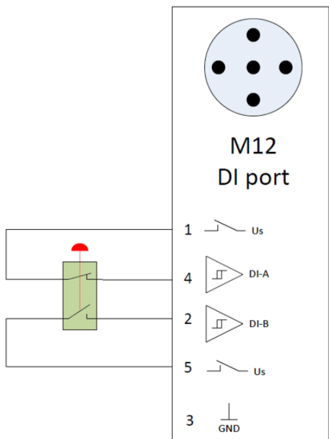
Abb. 17: Internes SDI Blockdiagramm
