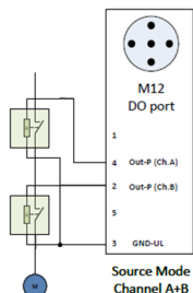
Abb. 8: Zulässiger Anwendungsfall für den Source-Modus
