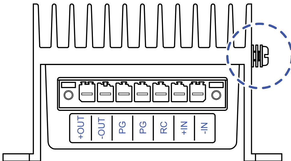
Abb. 3: Erden: Position der Erdungsschraube am Gerät (Gerätevorderseite)
