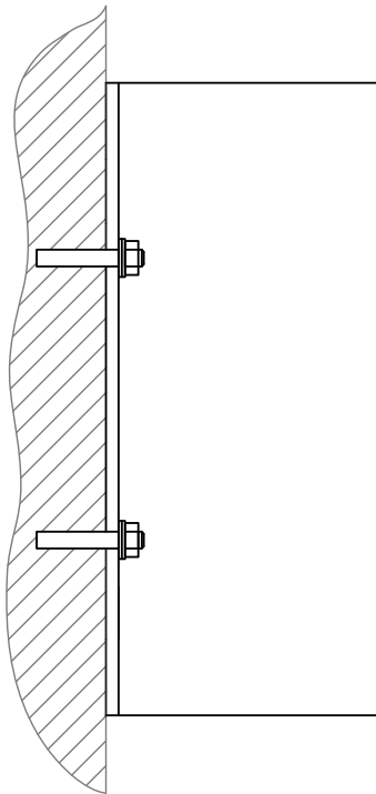
Abb. 2: Gerät montieren und erden: Vertikale Montage auf eine ebene Fläche (Seitenansicht)
