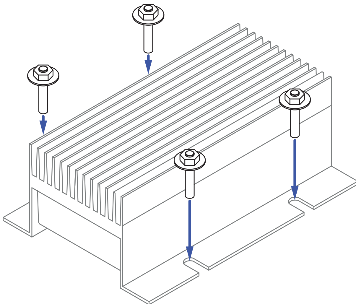
Abb. 1: Gerät montieren und erden: Montage auf eine ebene Fläche
