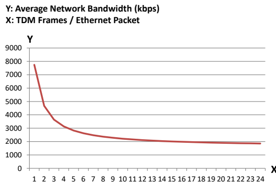
Figure 16 CESoPSN Bandwidth
