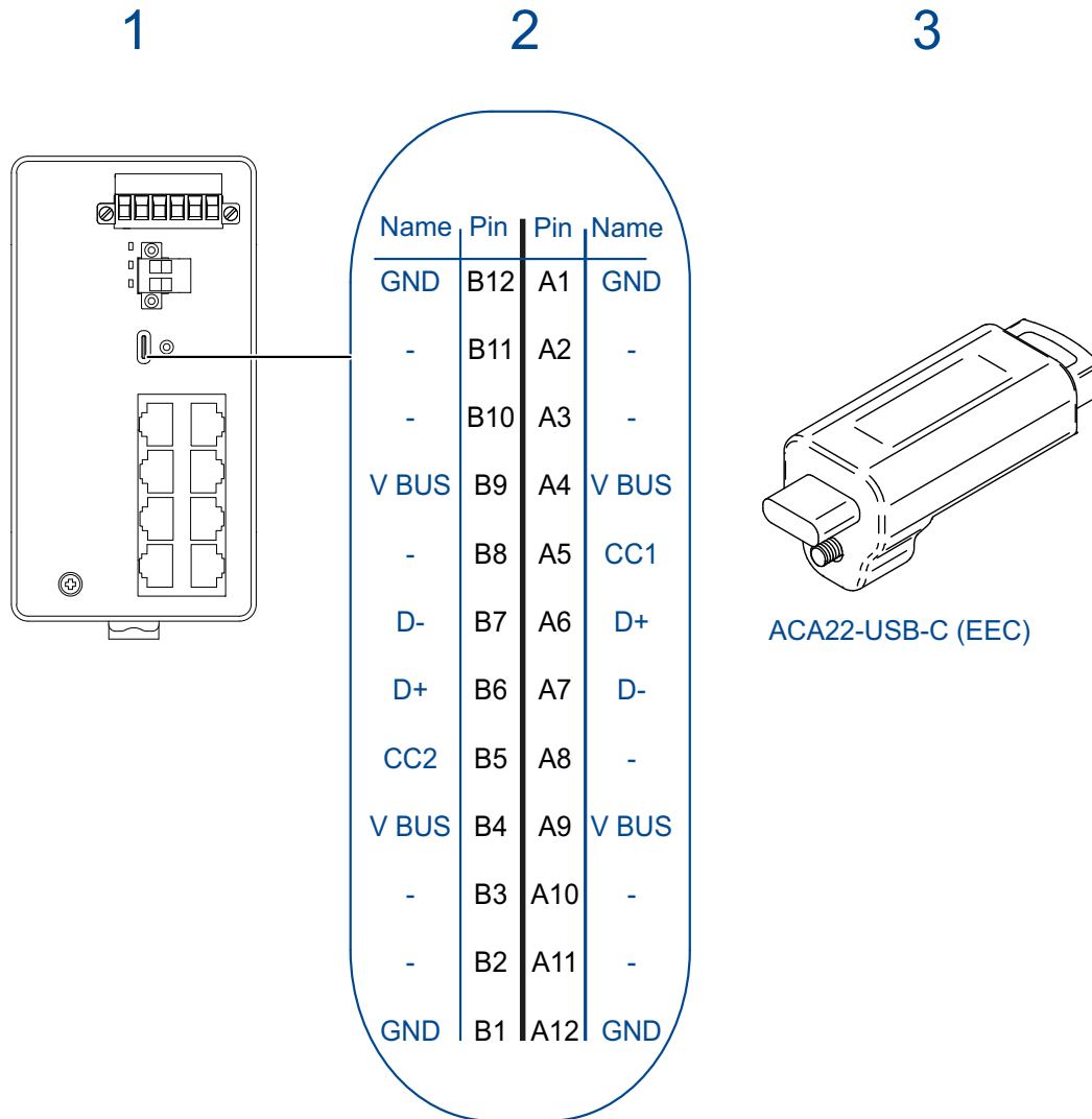
Abb. 6: (1) Position der USB-C-Schnittstelle am Gerät, (2) Pinbelegung der USB-C-Schnittstelle, (3) Ansicht des ACA22-USB-C (EEC).
