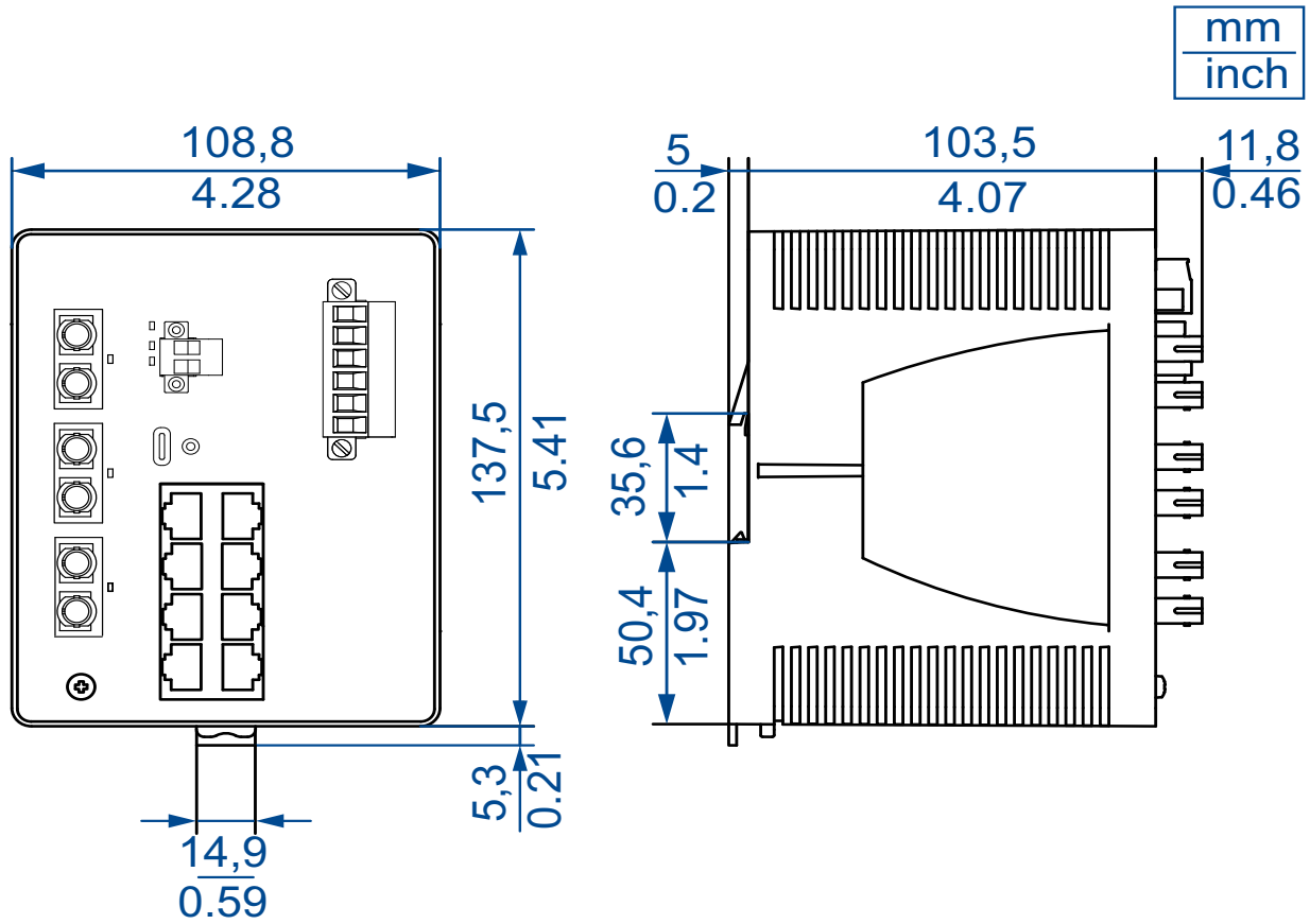
Abb. 25: Gerätevarianten im breiten Kunststoffgehäuse
