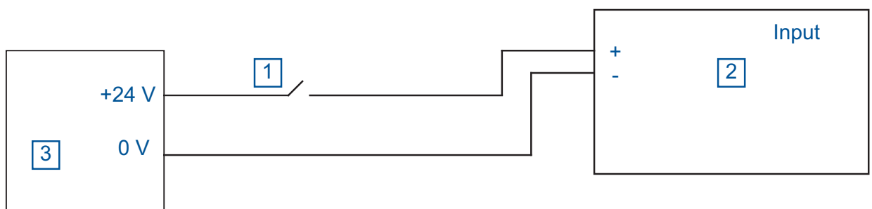
Abb. 20: Anschluss eines Sensors (2-Pol) mit gesonderter Spannungsversorgung 1 - Schalter (2-Pol-Sensor) 2 - BRS-Familie 3 - Gesonderte Spannungsversorgung für Sensor
