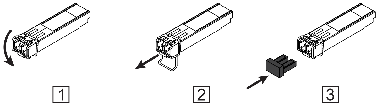
Abb. 21: SFP-Transceiver demontieren: Demontagereihenfolge
