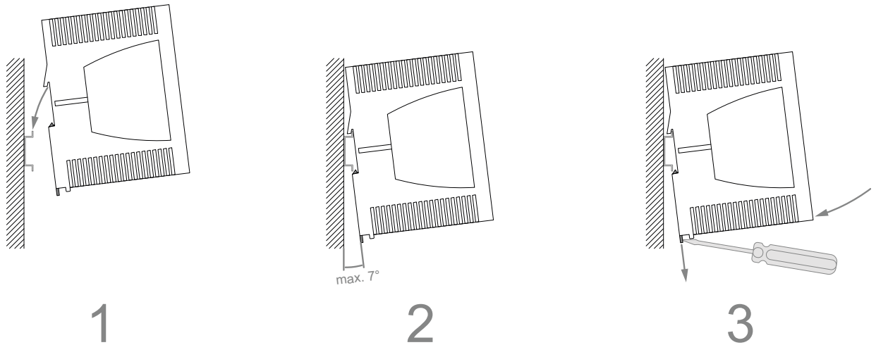
Abb. 10: Montage auf die Hutschiene
