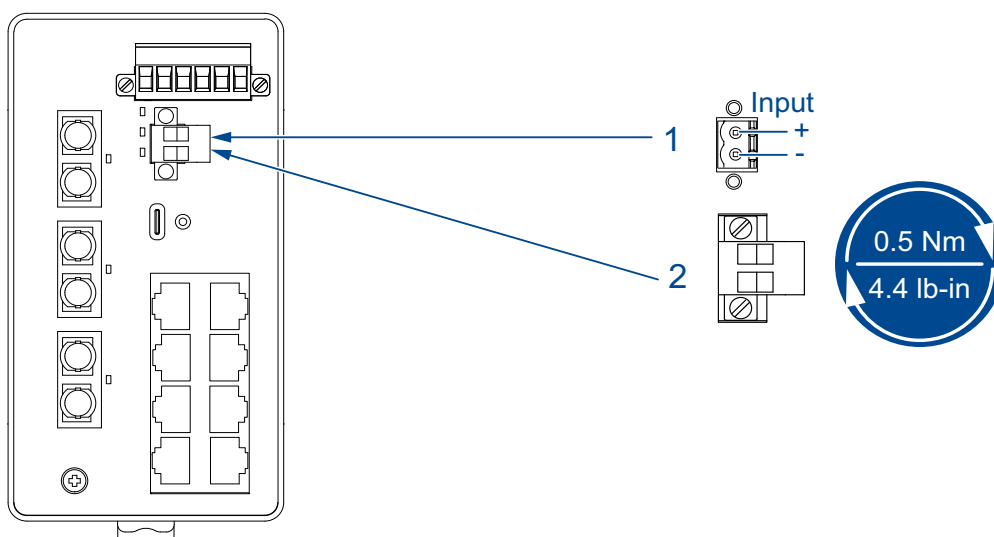
Abb. 18: (1) Anschluss am Gerät, (2) Klemmblock montiert am Gerät (Vorderansicht), Anzugsdrehmoment.
