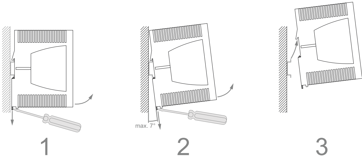
Abb. 22: Demontage von der Hutschiene
