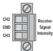
Fig.13: Sorties de tension analogiques – Affectation des broches sur le bornier à 3 pôles
