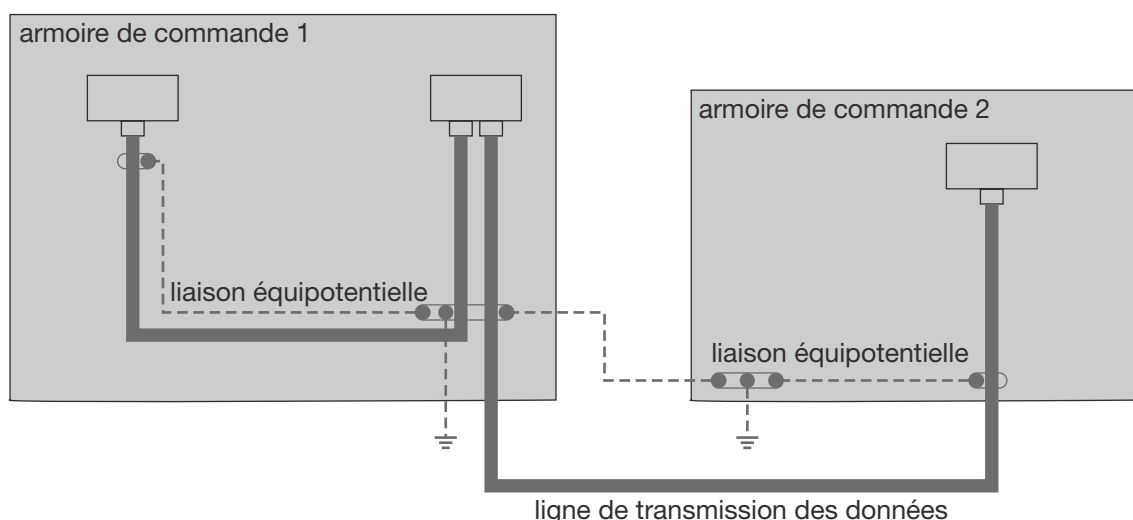
Fig. 6: Pose de câbles à l'intérieur de bâtiments
