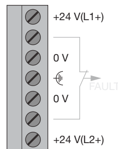
Abb. 14: Betriebsspannungsversorgung – Anschlussbelegung an der 7poligen Schraub-Klemmleiste
