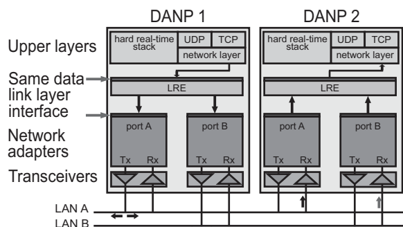
Abb. 35: Ablauf PRP/LRE
