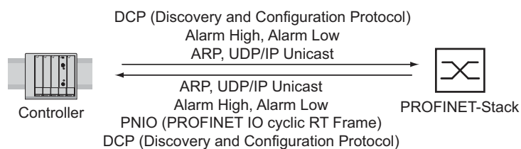
Abb. 61: Kommunikation zwischen Controller und dem Gerät
