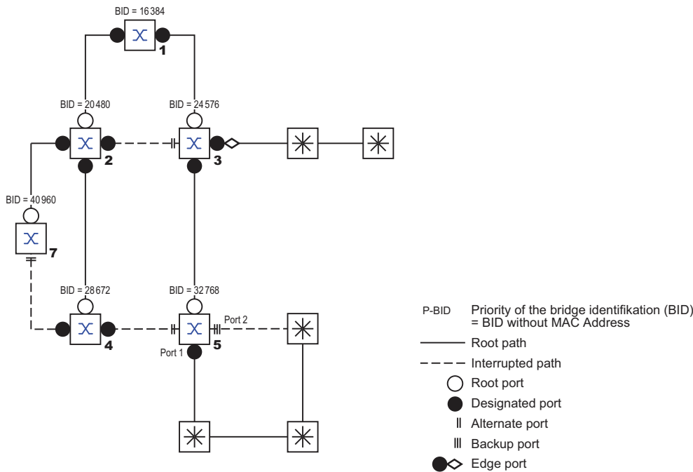
Abb. 50: Port-Rollen-Zuweisung
