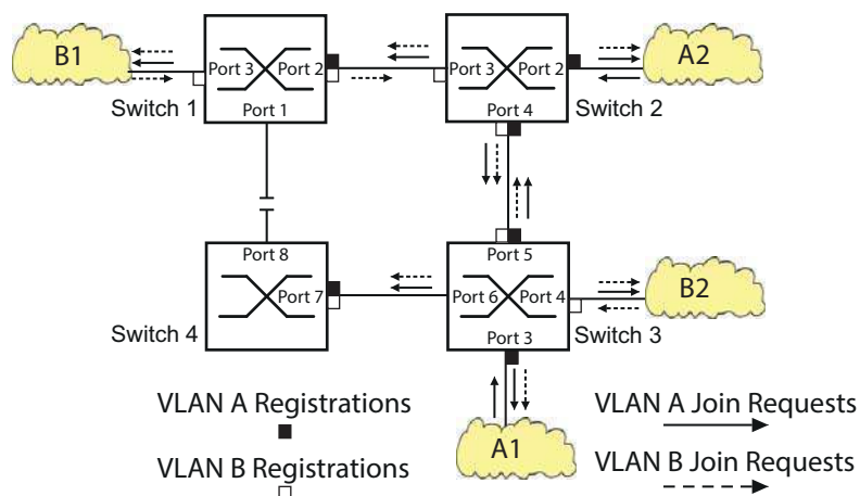
Abb. 55: MVRP-Beispiel-Netz für VLAN-Registrierung
