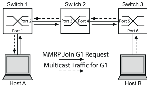
Abb. 54: MMRP -Netz für MAC-Adressen-Registrierung
