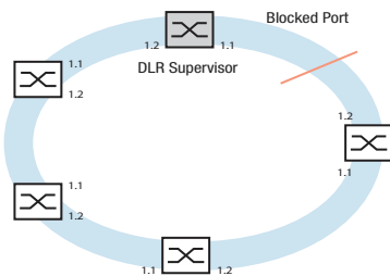
Abb. 31: DLR-Netz mit Ring-Teilnehmern
