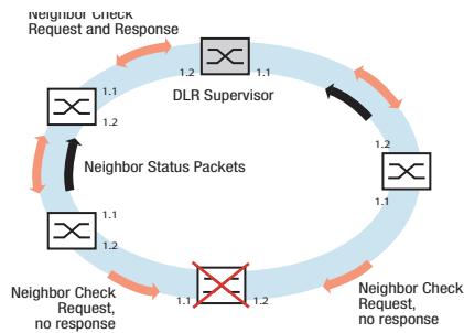
Abb. 33: Neighbor-Check-Prozess
