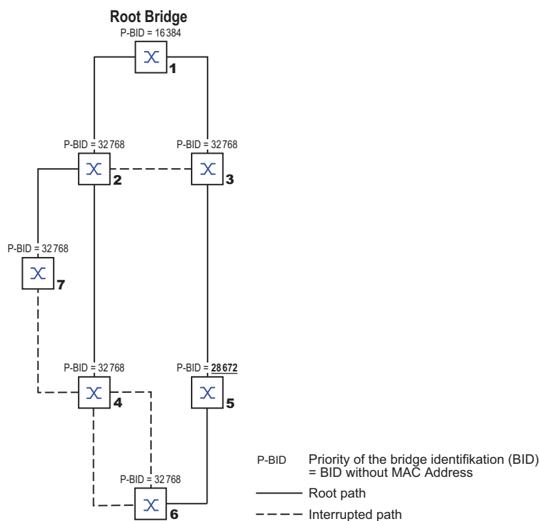
Abb. 48: Beispiel für die Manipulation des Root-Pfads
