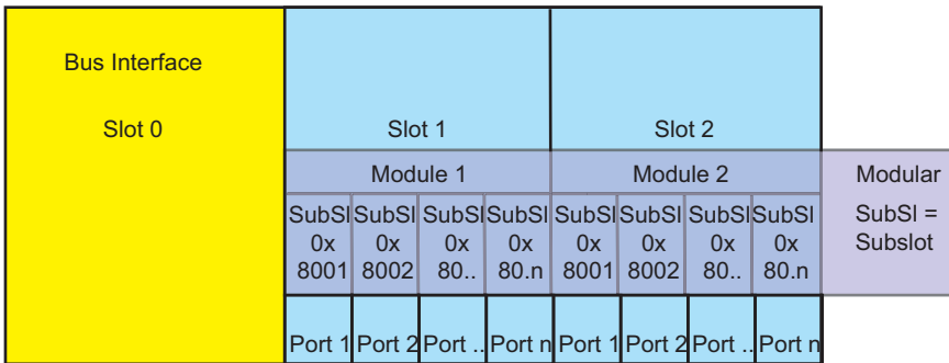
Abb. 63: Modulares Gerät
