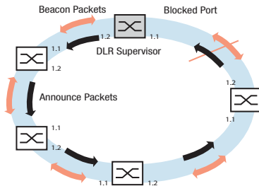
Abb. 32: Beacon- und Announce-Pakete
