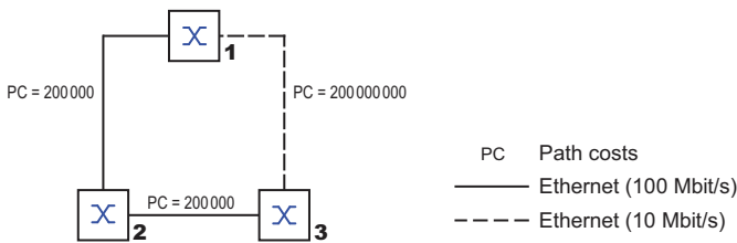
Abb. 42: Pfadkosten
