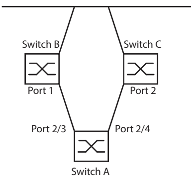
Abb. 52: Link-Backup Beispiel-Netzwerk
