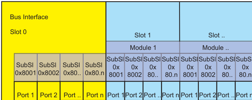
Abb. 64: Kombigerät
