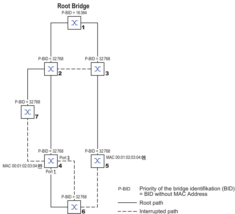
Abb. 47: Beispiel für die Bestimmung des Root-Pfads
