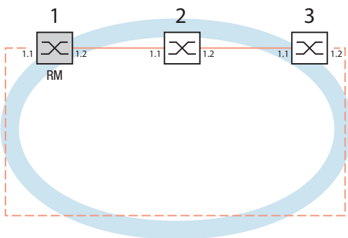
Abb. 30: Beispiel eines MRP-Rings RM = Ring-Manager — Hauptleitung - - - redundante Leitung
