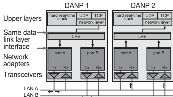
Abb. 35: Ablauf PRP/LRE
