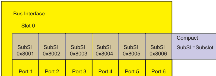
Abb. 62: Kompaktes Gerät
