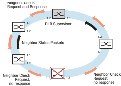
Abb. 33: Neighbor-Check-Prozess
