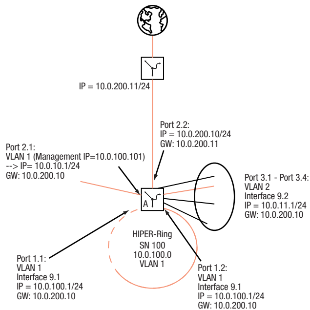
Abb. 113: IP-Parameter für Schicht-3-Gerät A
