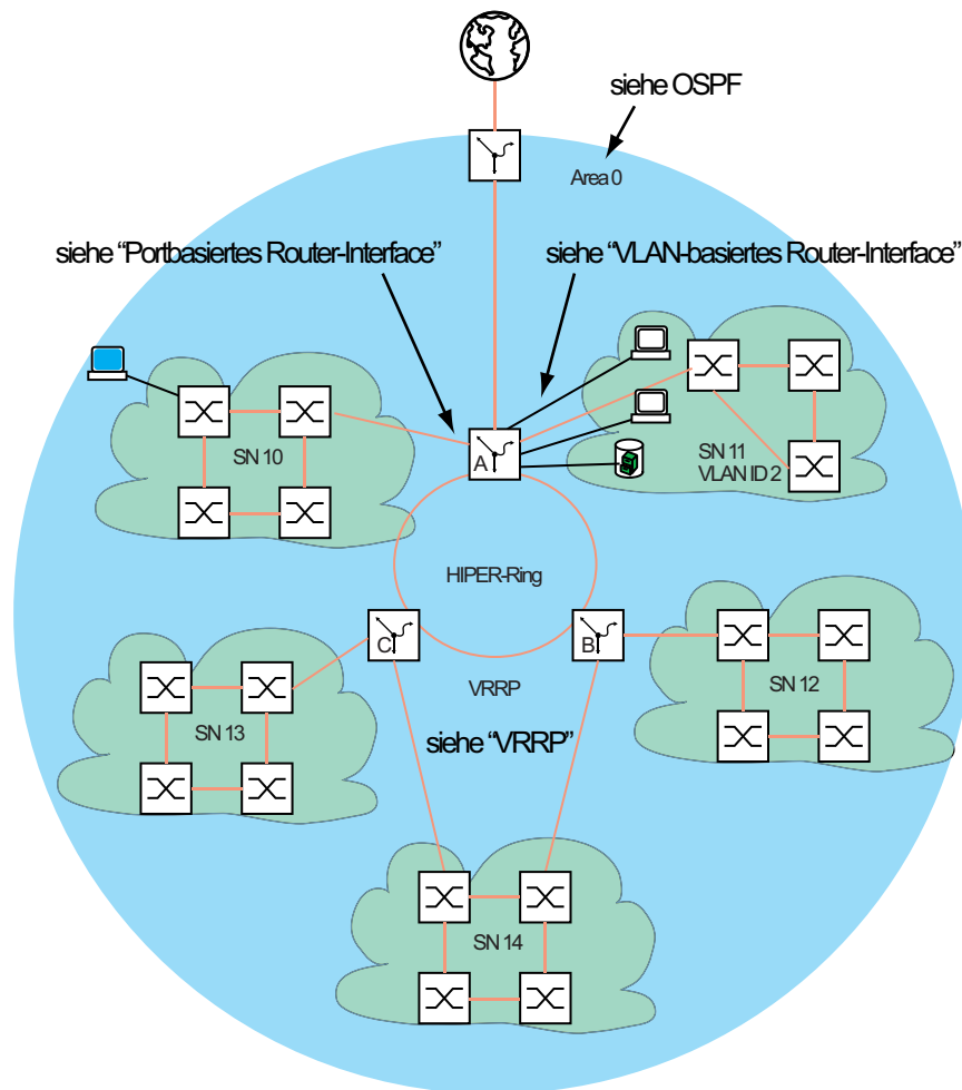
Abb. 111: Netzplan
