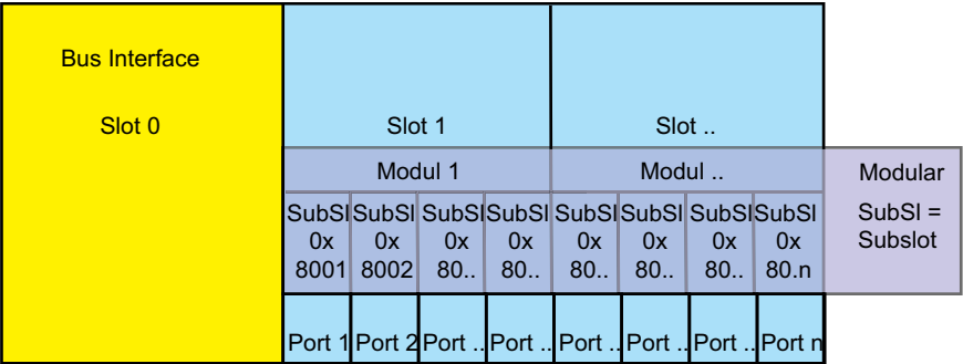
Abb. 127: Modulares Gerät
