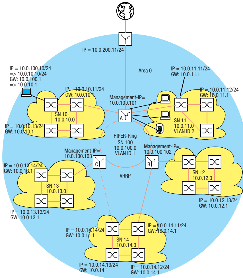
Abb. 112: Netzplan mit Management-IP-Adressen
