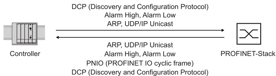
Abb. 125: Kommunikation zwischen Controller und dem Gerät
