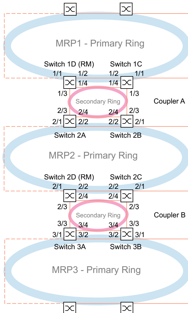
Abb. 74: Redundant Coupling Protocol-Zugtopologie:
