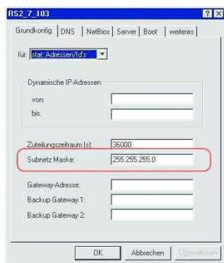
Abb. 133: Netzmaske im Konfigurationsprofil
