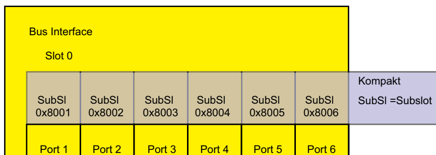
Abb. 126: Kompaktes Gerät
