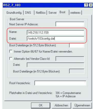
Abb. 134: Konfigurationsdatei auf dem tftp-Server
