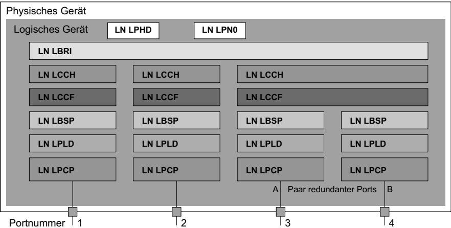
Abb. 121: Bridge-Modell nach Technical Report IEC 61850 90-4
