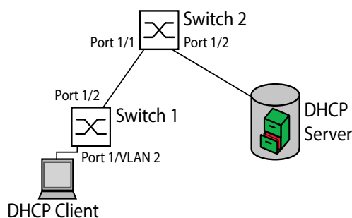
Abb. 117: Beispiel: DHCP-Schicht-2-Netz
