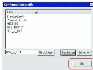
Abb. 135: Konfigurationsprofile verwalten
