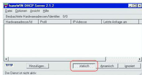
Abb. 136: Statische Adresseingabe
