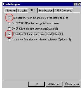
Abb. 141: DHCP-Einstellung
