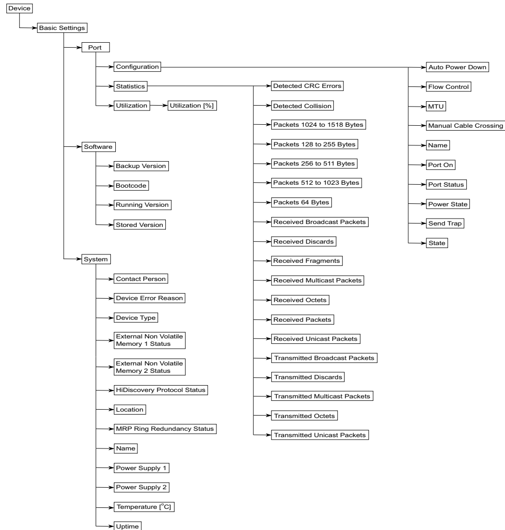
Abb. 129: OPC UA-Informationsmodell
