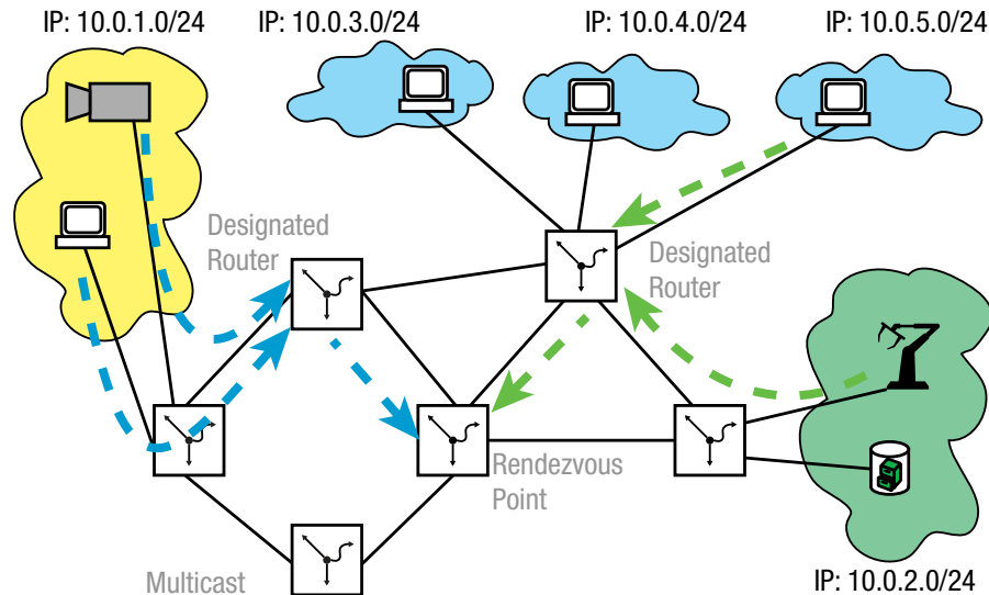
Abb. 116: Designated-Router leiten Nachrichten von Multicast-Quellen und Multicast-Teilnehmern an den Rendezvous-Point weiter
