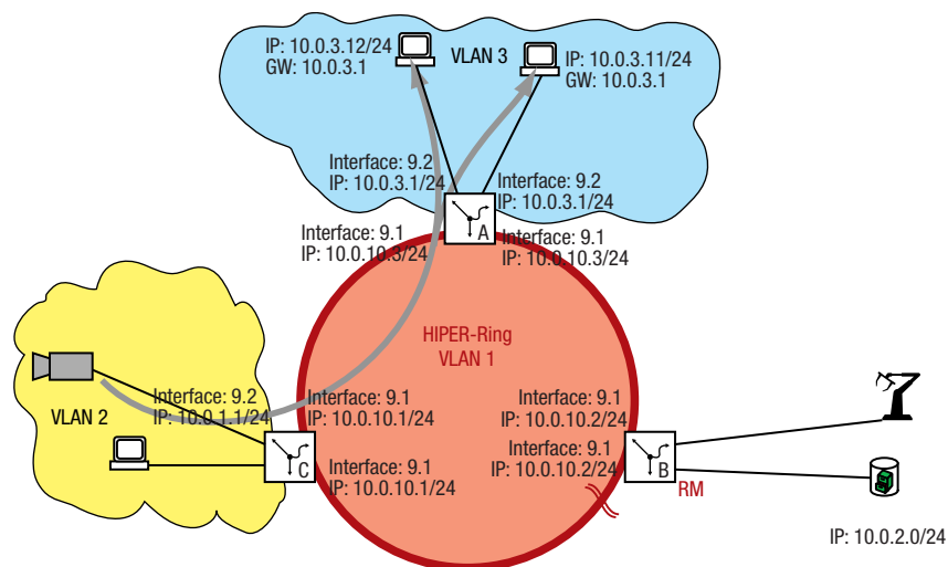
Abb. 120: Multicast-Beispielkonfiguration mit HIPER-Ring
