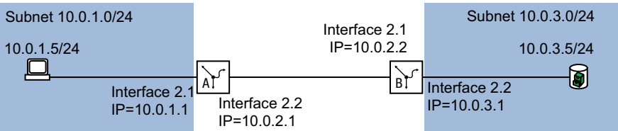
Abb. 84: Statisches Routing
