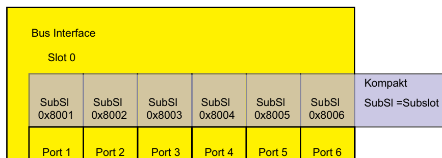
Abb. 137: Kompaktes Gerät
