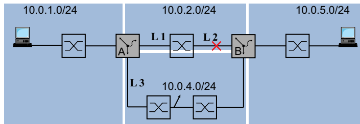
Abb. 86: Beispiel für statisches Route-Tracking
