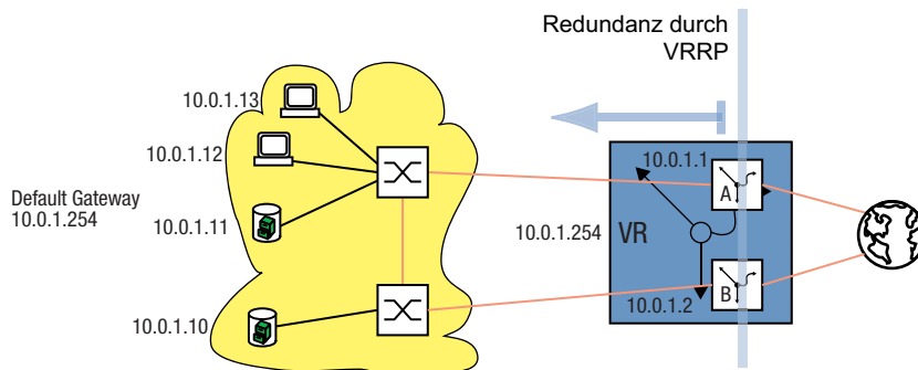
Abb. 92: Darstellung des virtuellen Routers
