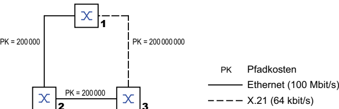
Abb. 41: Pfadkosten
