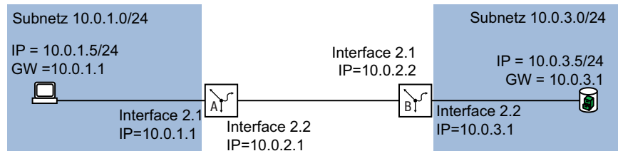
Abb. 101: Beispiel für die Konfiguration von RIP
