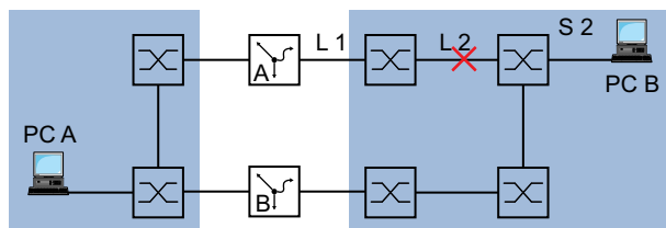
Abb. 89: Überwachen einer Leitung mit Ping-Tracking
