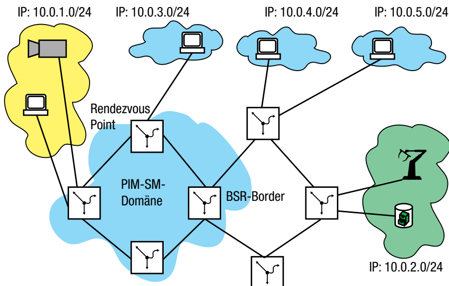
Abb. 117: Als BSR-Border-Router konfigurierte Router verwerfen Bootstrap-Nachrichten und begrenzen die PIM-SM-Domäne.
