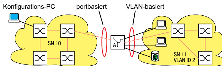
Abb. 81: Statische Routen: Beispiel für eine Verbindung zwischen zwei Fertigungszellen.
