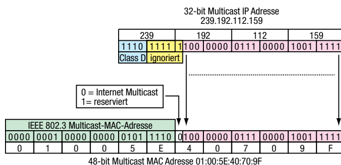
Abb. 110: Umsetzung der IP-Adresse in die MAC-Adresse
