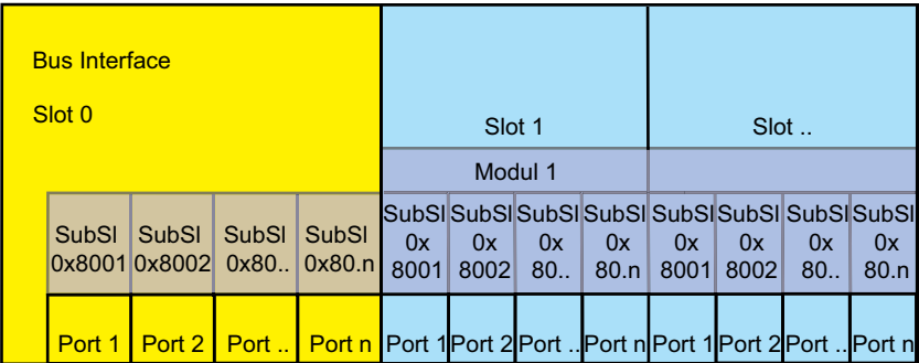
Abb. 139: Kombigerät
