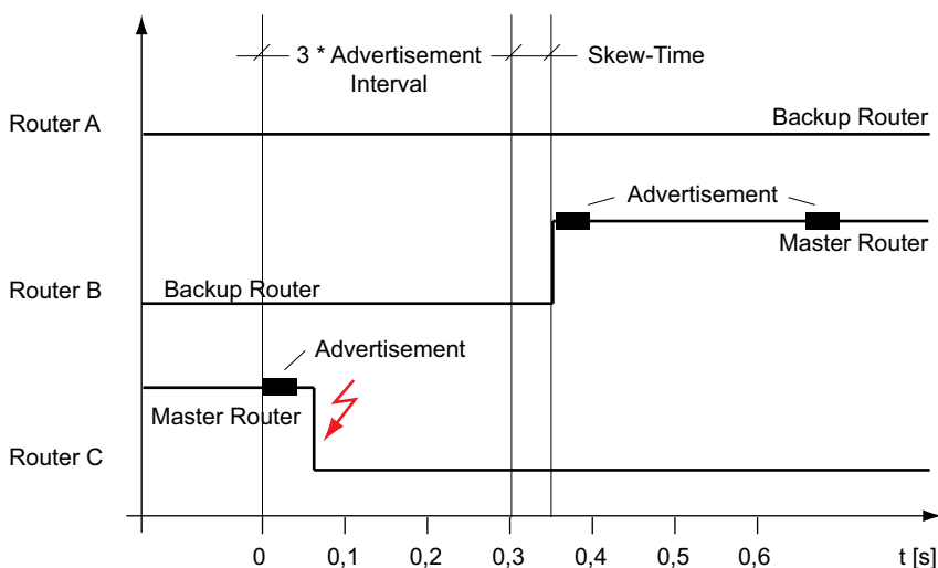
Abb. 95: Umschaltzeiten Master-Router <-> Backup-Router nach HiVRRP
