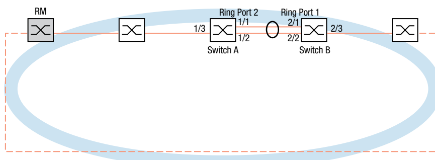
Abb. 39: Beispielkonfiguration für MRP-over-LAG
