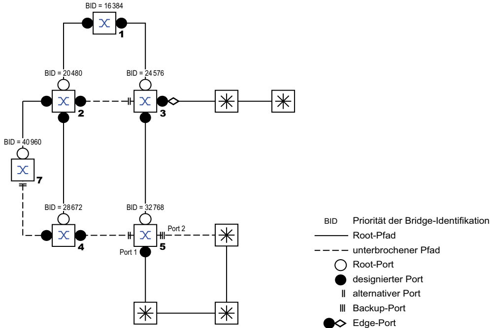
Abb. 49: Port-Rollen-Zuweisung
