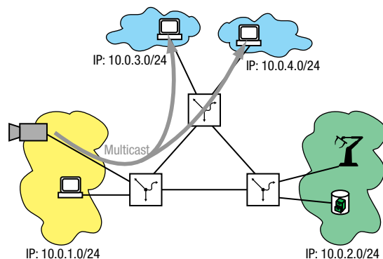
Abb. 109: Beispiel für eine Multicast-Anwendung
