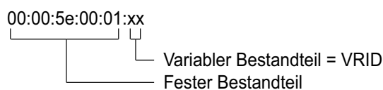
Abb. 93: Virtuelle MAC-Adresse
