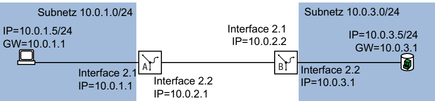
Abb. 107: Beispiel für die Konfiguration von OSPF
