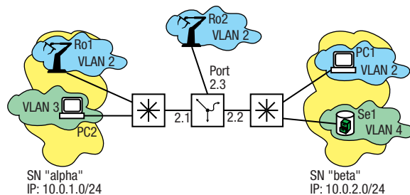
Abb. 108: Beispiel für ein Protokoll-basiertes VLAN
