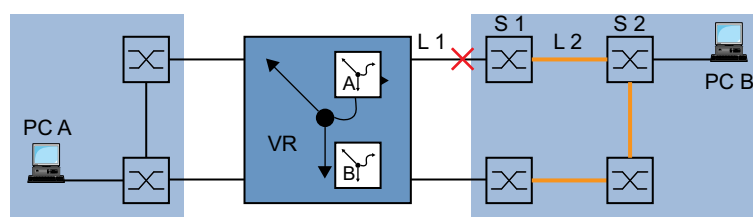
Abb. 88: Überwachen einer Leitung mit Interface-Tracking
