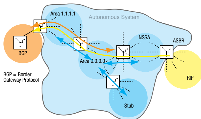
Abb. 103: LSA-Verteilung in die Area-Typen
