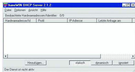
Abb. 141: Startfenster des Programms hanewIN DHCP Server
