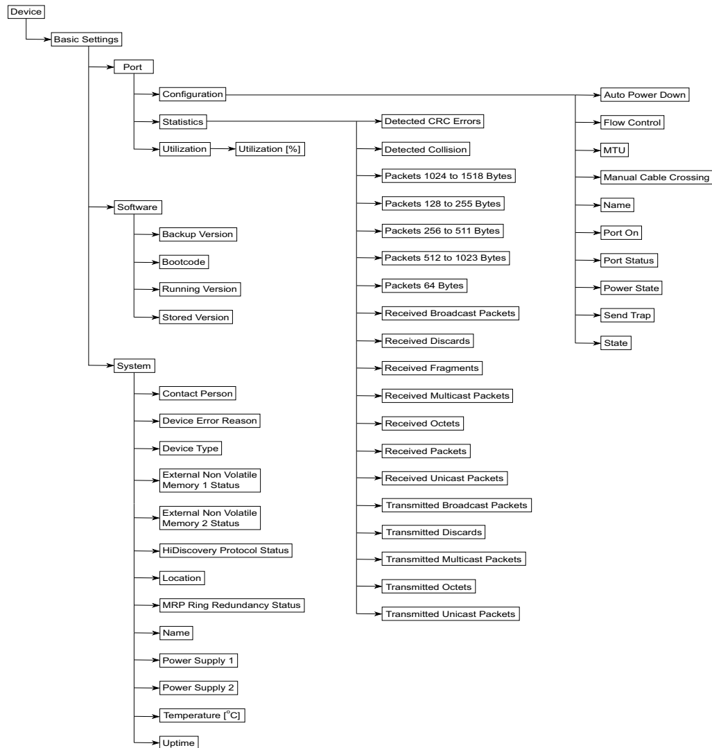
Abb. 140: OPC UA-Informationsmodell
