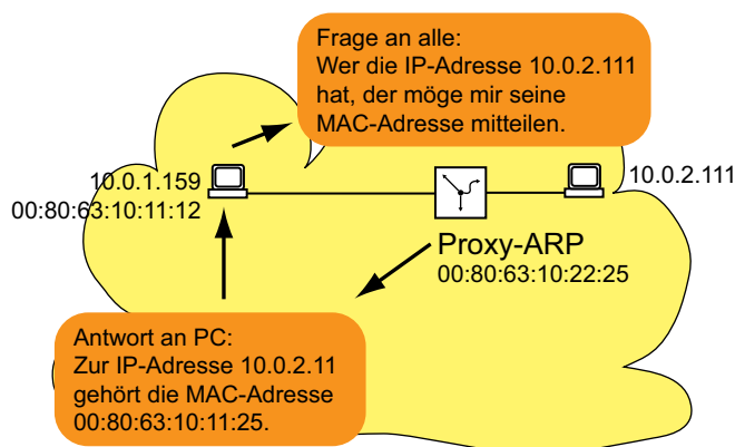
Abb. 79: Funktion Proxy-ARP
