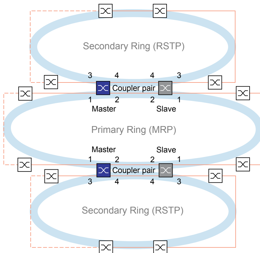
Abb. 73: Beispiel einer redundanten 2-Switch-Kopplung (2 Kopplerpaare)
