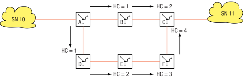
Abb. 99: Zählen des Hop Count
