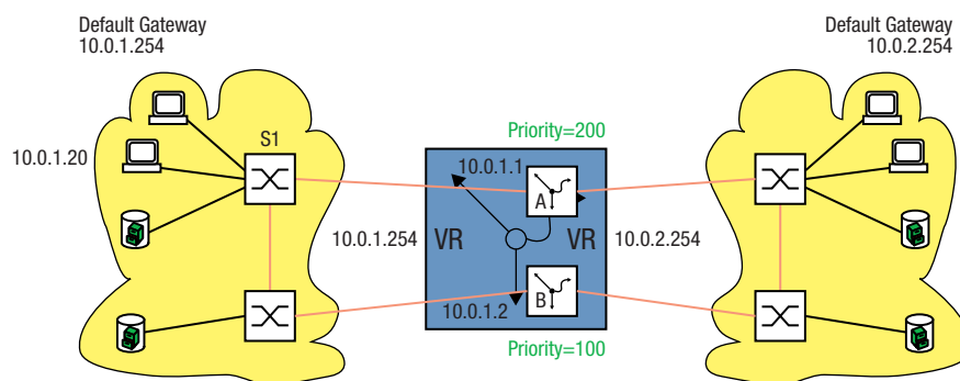
Abb. 97: Virtueller Router mit Lastverteilung
