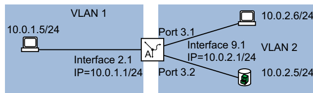
Abb. 83: VLAN-basiertes Router-Interface
