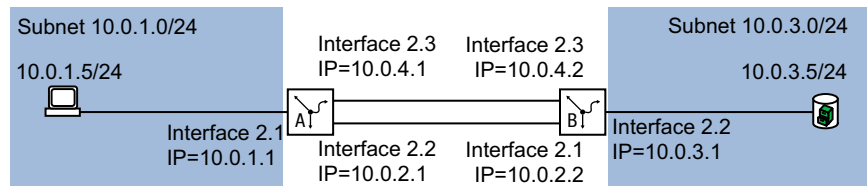
Abb. 85: Redundante statische Route
