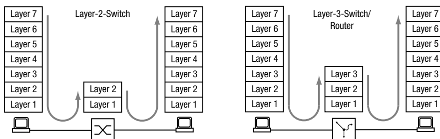
Abb. 75: Datentransport durch einen Switch und einen Router in den Schichten des OSI-Referenzmodells
