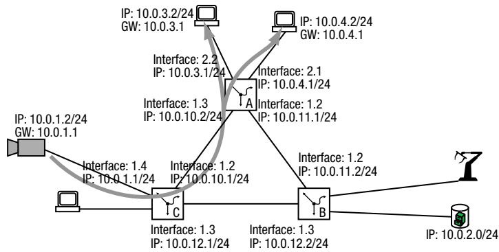
Abb. 119: Multicast-Beispielkonfiguration
