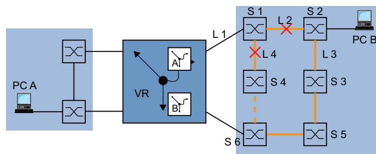
Abb. 91: Überwachen der Erreichbarkeit eines Geräts in einem redundanten Ring
