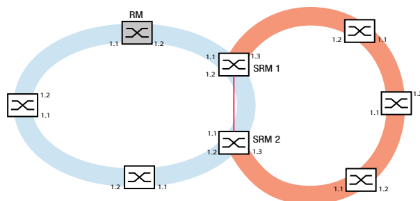
Abb. 52: Beispiel für eine Subring-Struktur blauer Ring = Hauptring oranger Ring = Subring rote Linie = redundante Verbindung des Subrings SRM = Subring-Manager RM = Ring-Manager
