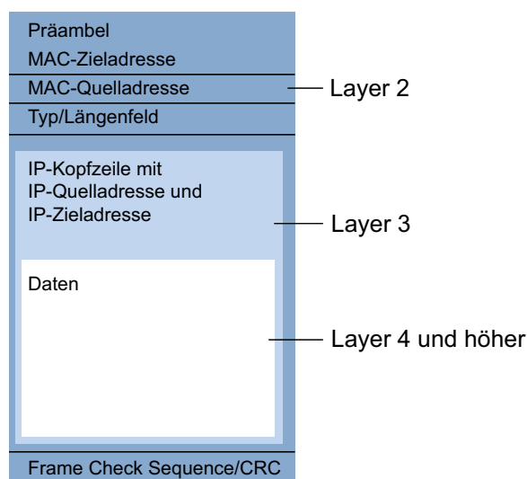
Abb. 78: Aufbau eines Datenpaketes aus Sicht des ISO/OSI-Referenzmodells
