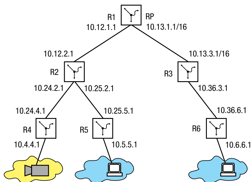
Abb. 118: Beispielkonfiguration für PIM-SM
