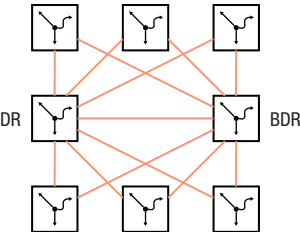
Abb. 106: LSA-Verteilung mit Designated-Router und Backup-Designated-Router
