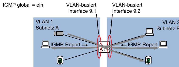
Abb. 121: Registrierter Multicast-Datenstrom auf dem VLAN-Router-Interface
