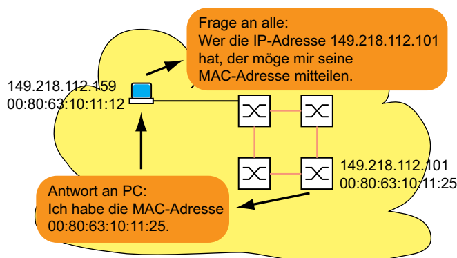
Abb. 77: ARP-Anfrage und -Antwort
