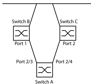
Abb. 51: Link-Backup Beispiel-Netzwerk
