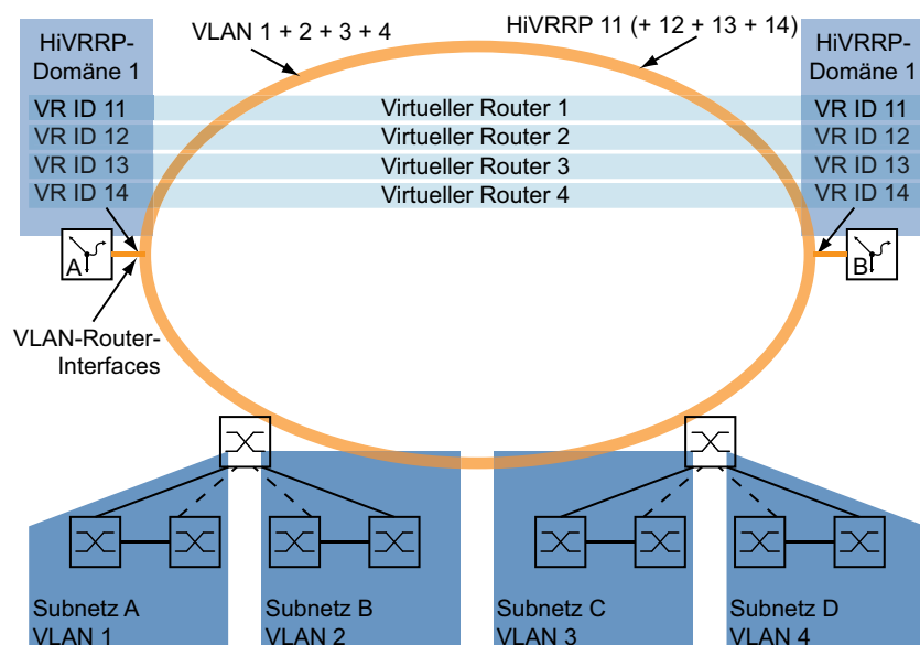
Abb. 96: Beispiel für die Anwendung einer HiVRRP-Domäne
