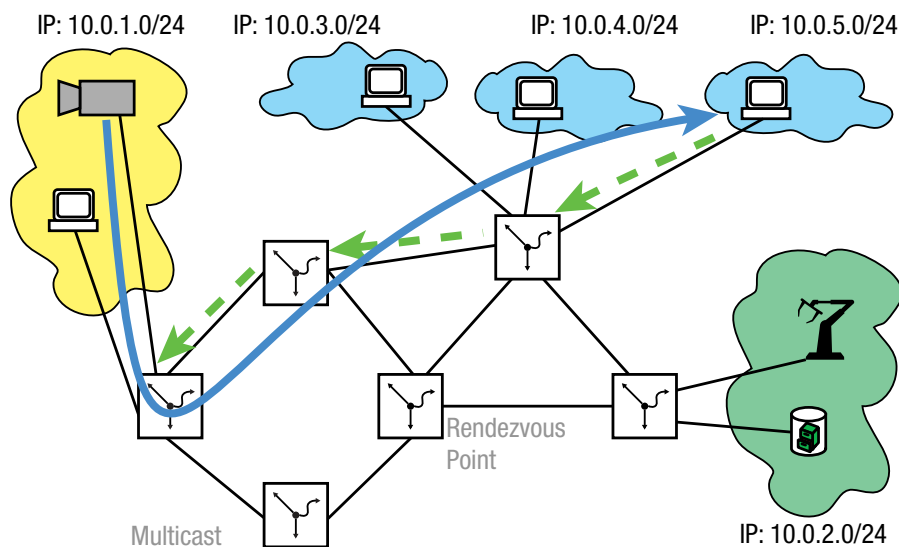
Abb. 115: Topologiewechsel vom RPT auf den direkten Pfad (SPT)
