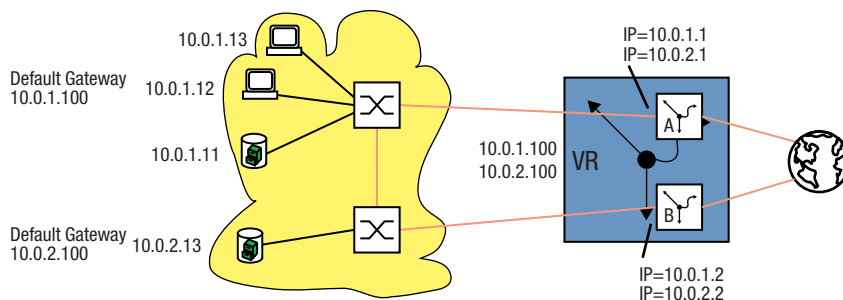
Abb. 98: Virtueller Router mit Multinetting
