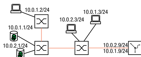
Abb. 80: Beispiel für Multinetting
