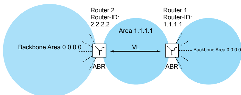
Abb. 105: Erweiterung der Backbone-Area durch eine virtuelle Verbindung (VL)
