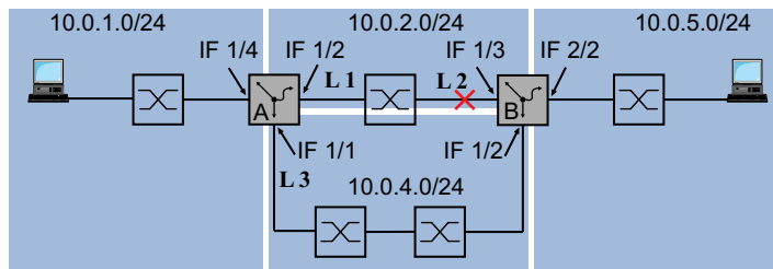
Abb. 87: Statisches Route-Tracking konfigurieren
