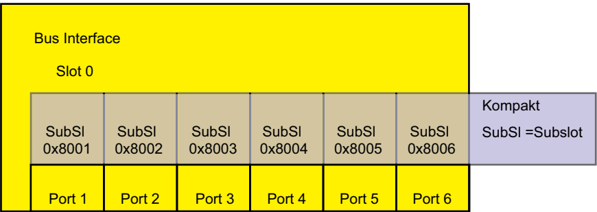
Abb. 86: Kompaktes Gerät
