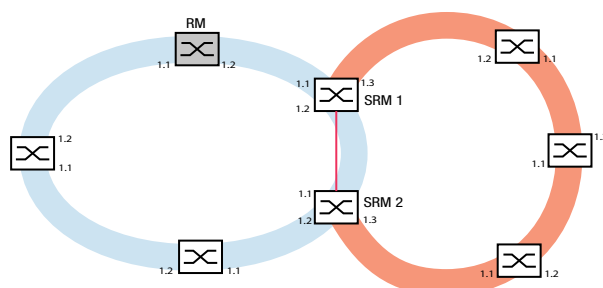
Abb. 51: Beispiel für eine Subring-Struktur blauer Ring = Hauptring oranger Ring = Subring rote Linie = redundante Verbindung des Subrings SRM = Subring-Manager RM = Ring-Manager
