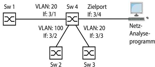
Abb. 76: Beispielkonfiguration für VLAN-Mirroring
