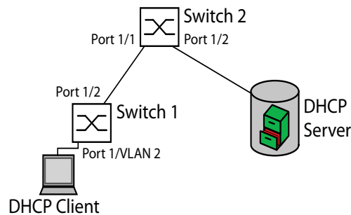
Abb. 77: Beispiel: DHCP-Schicht-2-Netz
