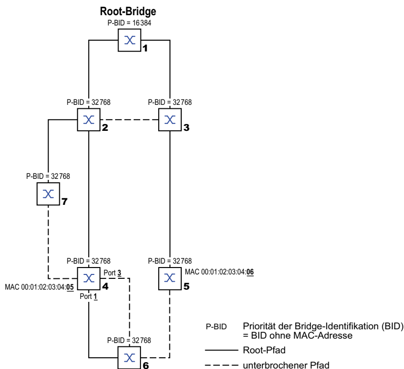
Abb. 45: Beispiel eines Netzplans für die Bestimmung des Root-Pfads
