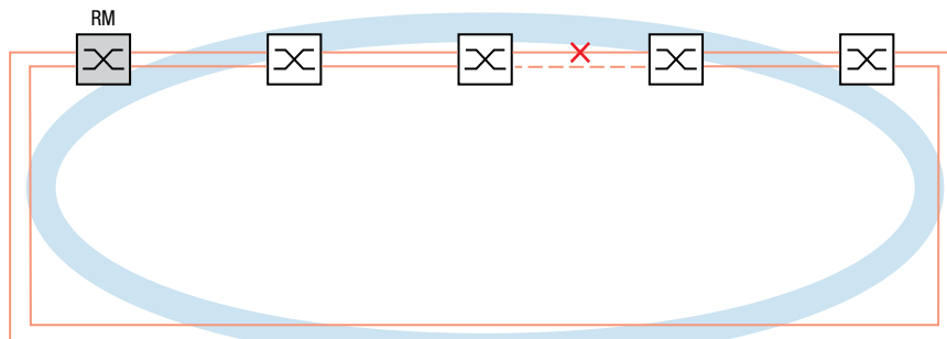
Abb. 37: Unterbrechung einer Verbindung in einem MRP-Ring
