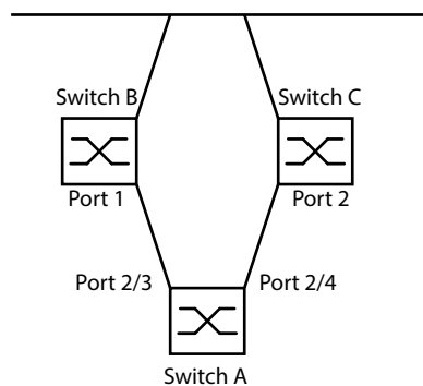
Abb. 50: Link-Backup Beispiel-Netzwerk
