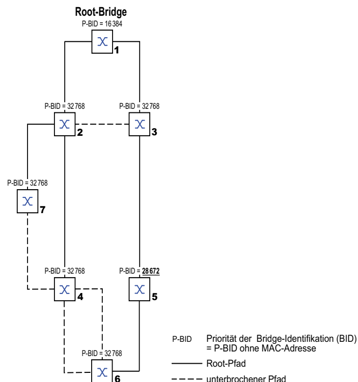
Abb. 46: Beispiel eines Netzplans für die Manipulation des Root-Pfads
