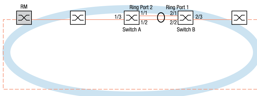
Abb. 38: Beispielkonfiguration für MRP-over-LAG
