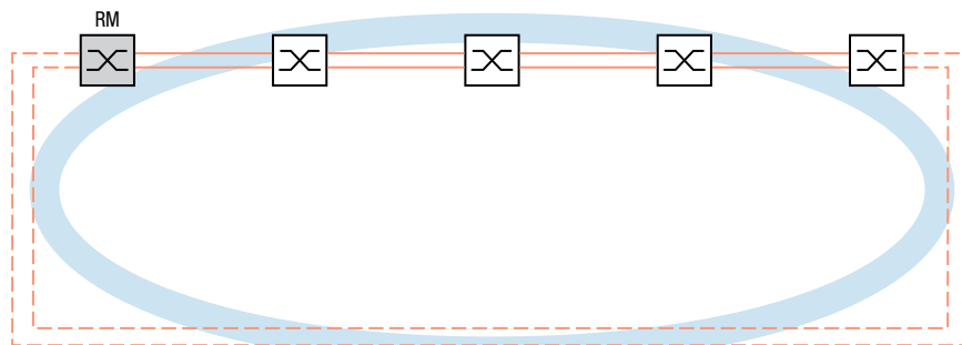
Abb. 36: Link-Aggregation für den gesamten MRP-Ring
