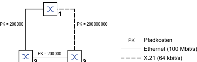
Abb. 40: Pfadkosten
