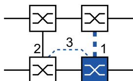
Abb. 71: 2-Switch-Kopplung mit Steuerleitung, Standby-Gerät 1: Kopplungs-Port 2: Partner-Kopplungs-Port 3: Steuerleitung
