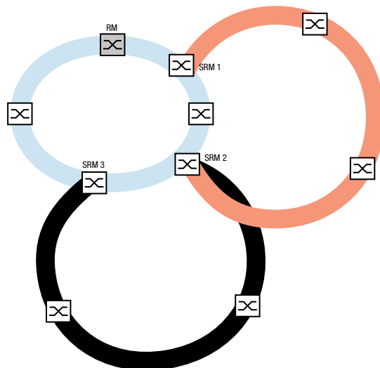
Abb. 53: Sonderfall: Ein Subring-Manager verwaltet 2 Subringe (2 Instanzen). Der Subring-Manager ist in der Lage, bis zu 8 Instanzen zu verwalten.
