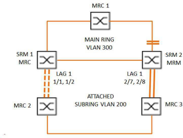
Abb. 56: Subring mit Link-Aggregation
